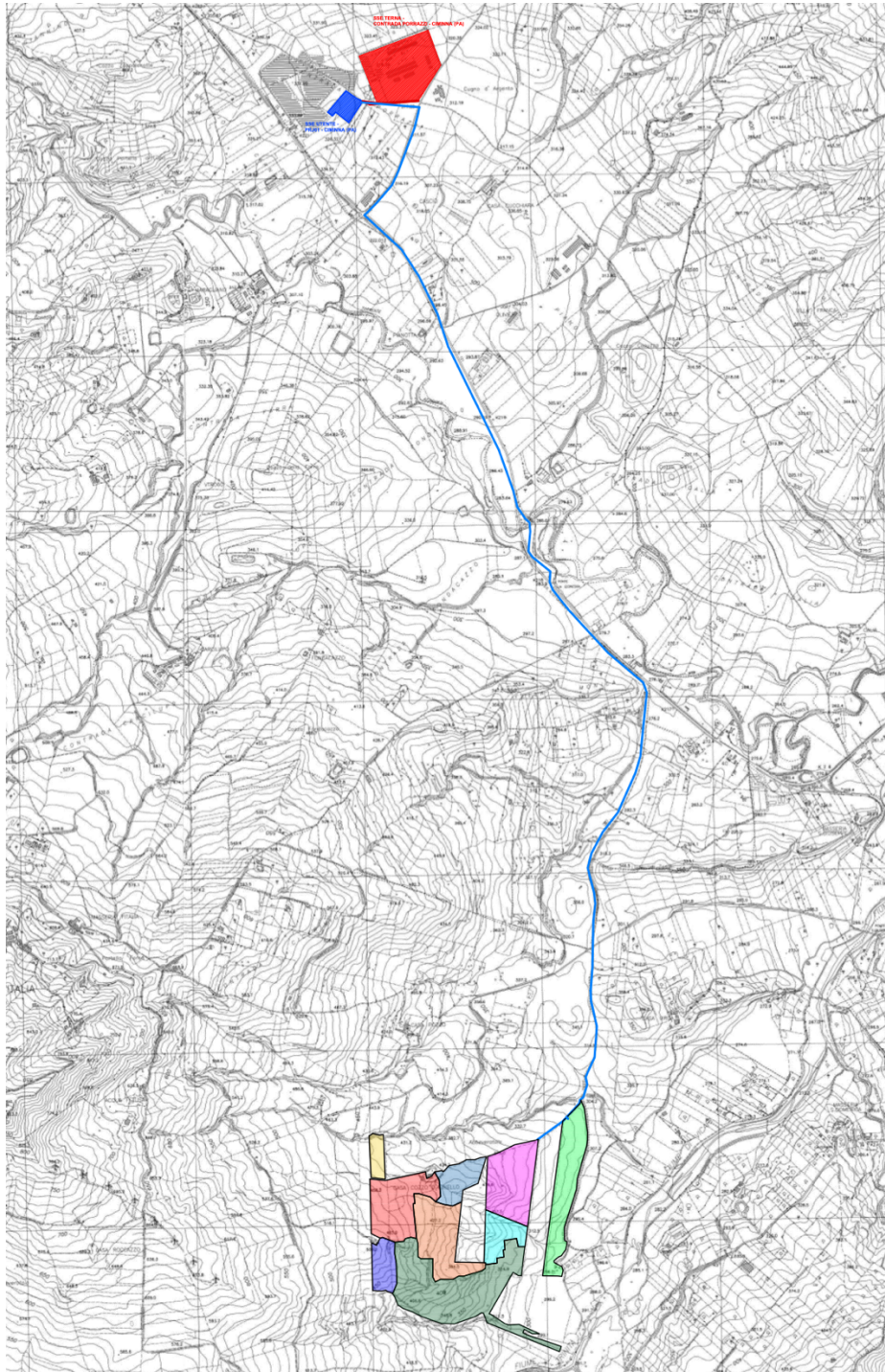
Figura 4 - Layout generale impianto agro-fotovoltaico e relative opere connesse
