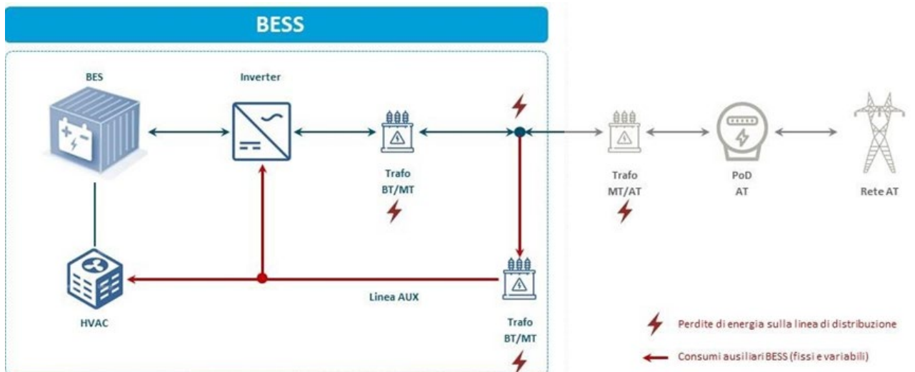
Figura 1 - Schema di impianto generico ed illustrativo
