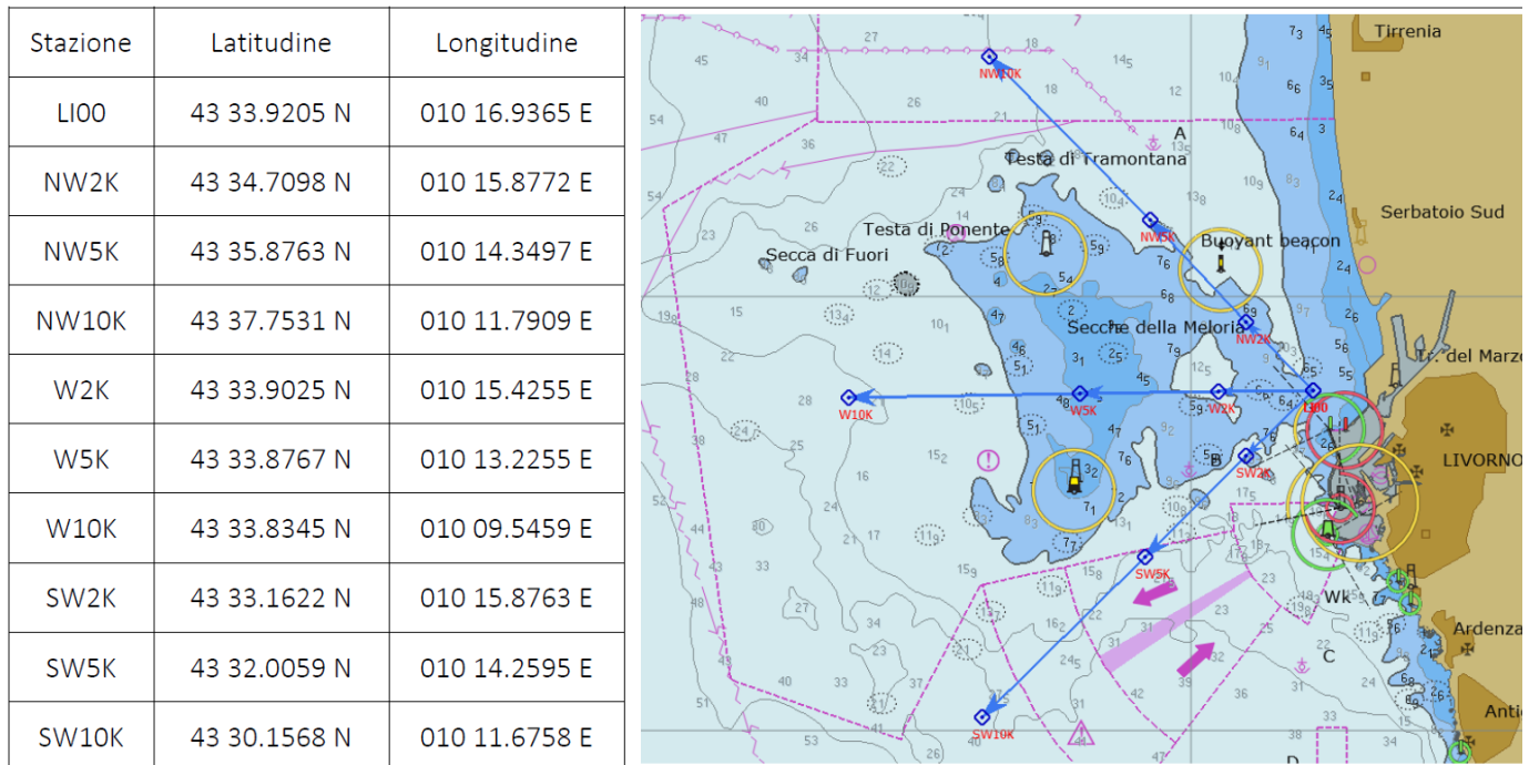
Figura 8: Stazioni di campionamento acustico sottomarino
