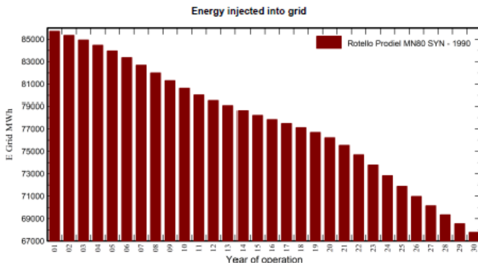
Fig. 30 – Producibilità dell’impianto con degrado moduli (30 anni)
