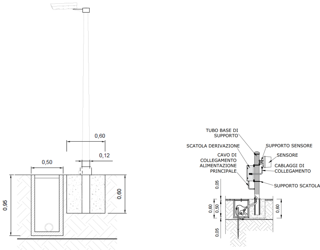
Fig. 24 – Sistema antintrusione
