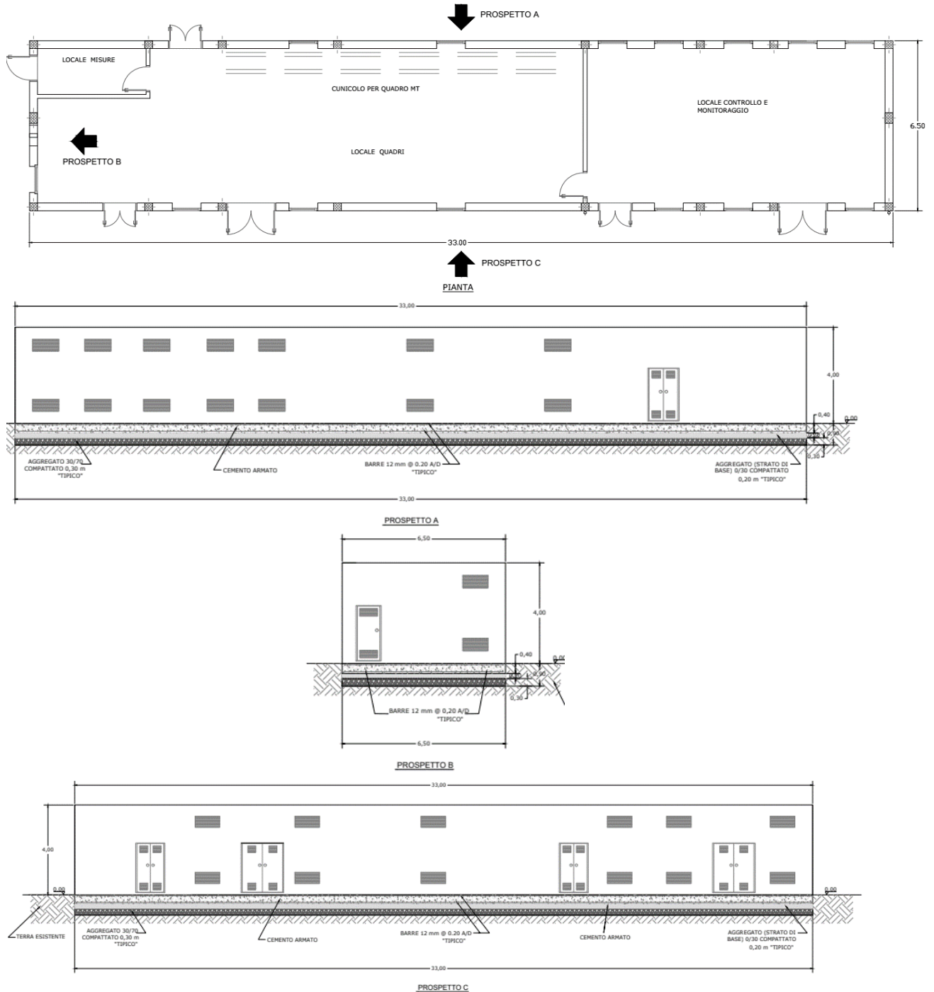
Fig. 22 - Cabina di ricezione
