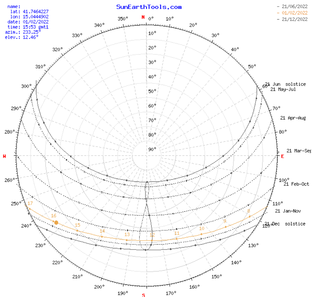
Fig. 27 - Diagramma Solare Polare
