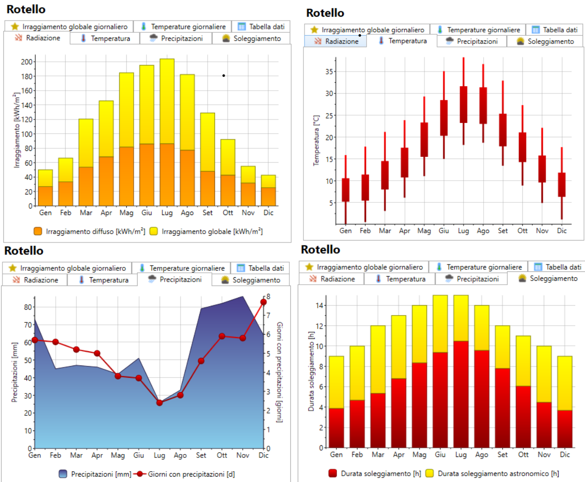
Fig. 26 – Dati di radiazione, temperatura, precipitazioni e soleggiamento (Riferiti al sito di Rotello)
