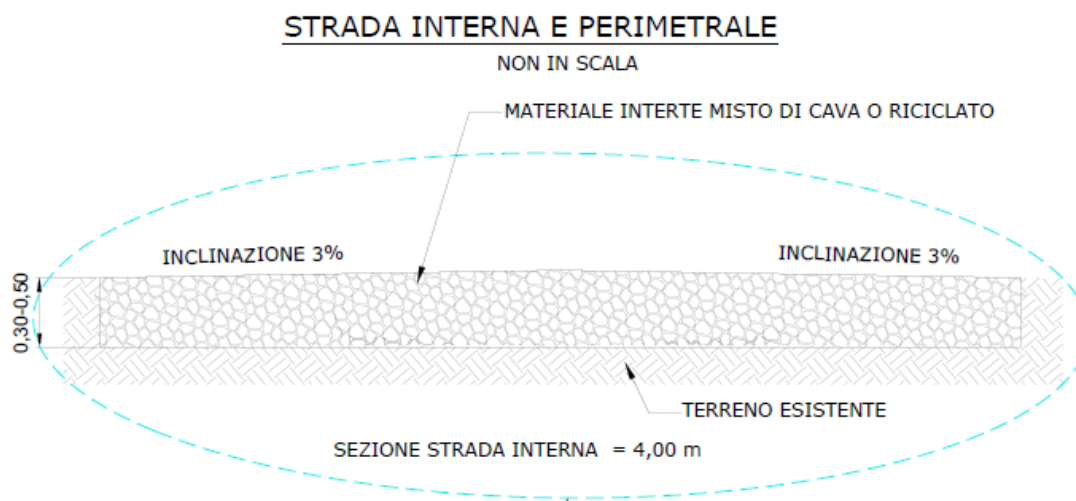
Fig. 19 – Viabilità interna
