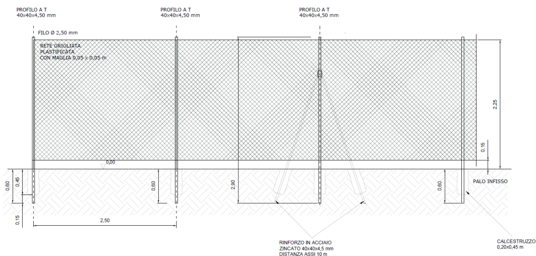
Fig. 17 – Recinzione perimetrale
