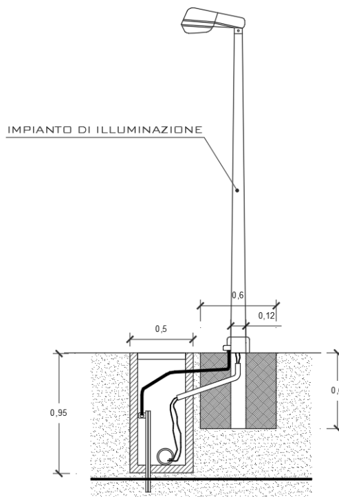
Fig. 25 – Sistema di illuminazione
