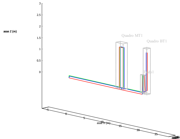
Fig.7 - Modello spaziale cablaggi nelle cabine di ricezione
