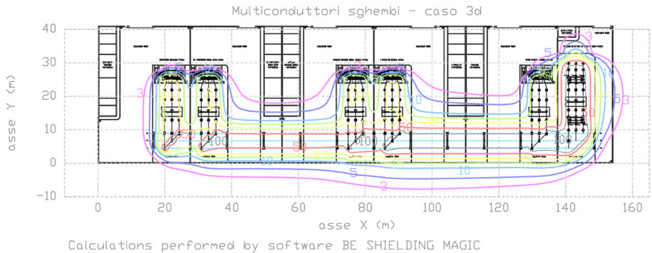
Figura 6 – Calcolo dei livelli di campo magnetico a 6 m da terra
