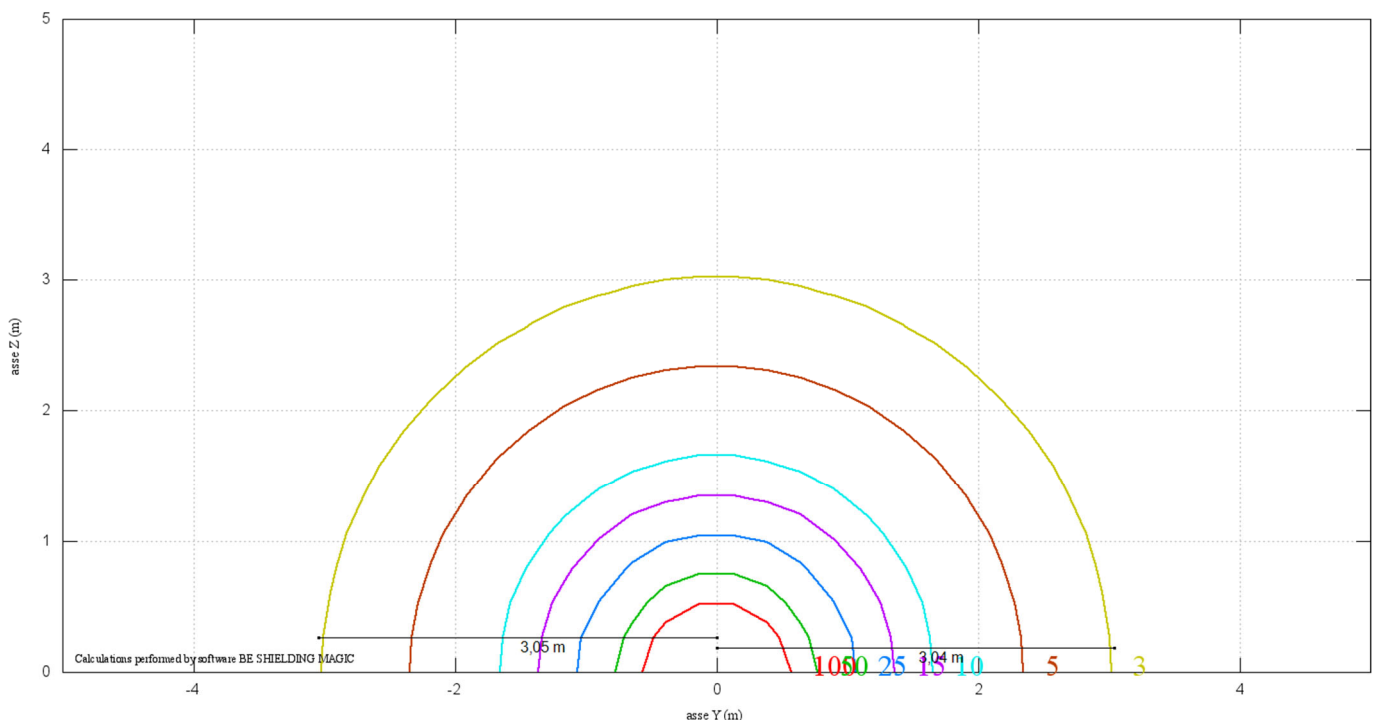
Figura 7 – Calcolo dei livelli di campo prodotto dal cavo AT comune
