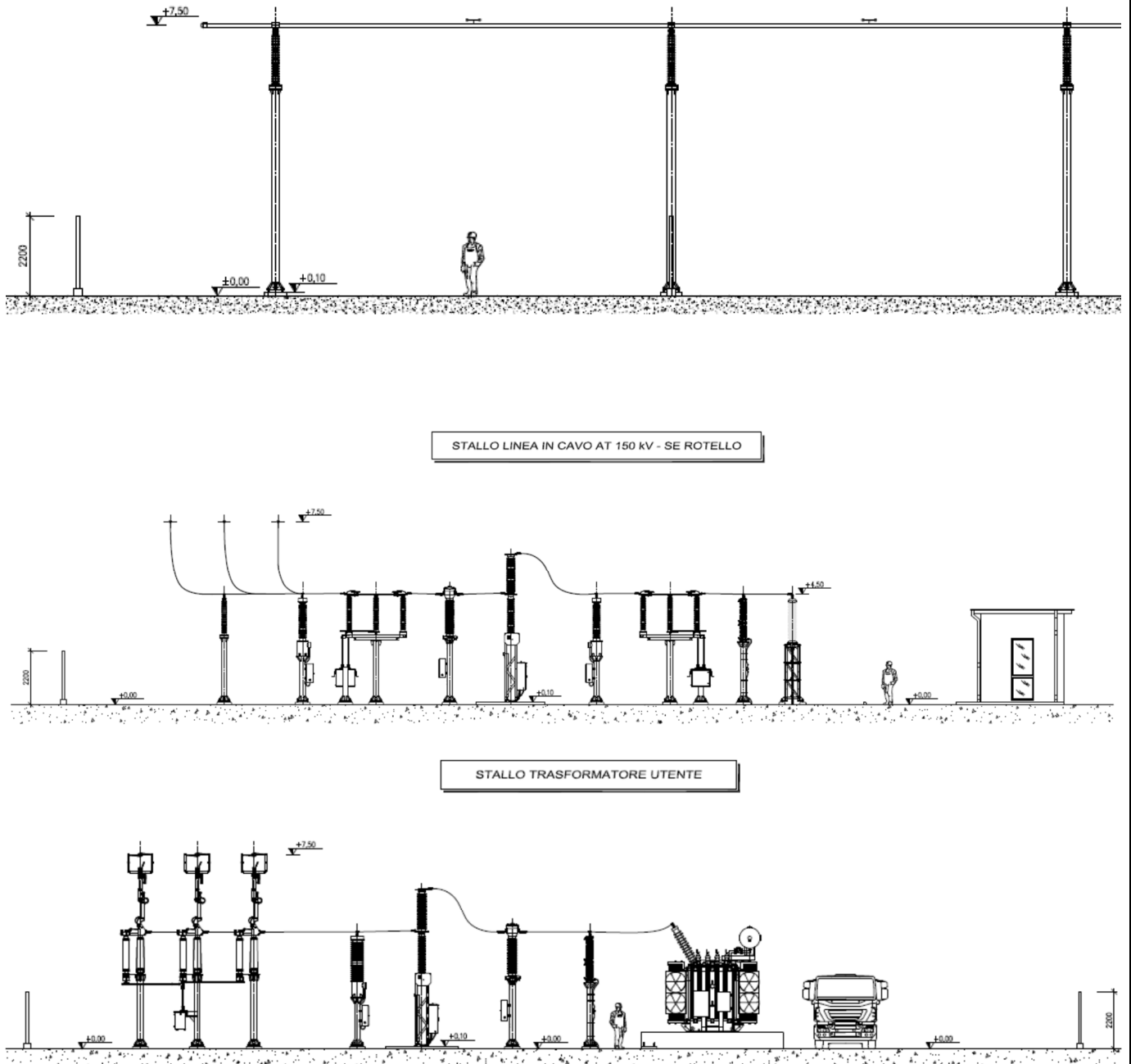
Figura 2 – Sezioni del Punto di Raccolta con individuazione delle altezze
