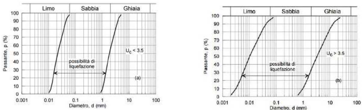
Figura 34: Fusi granulometrici di terreni suscettibili di liquefazione ai sensi delle NTC
