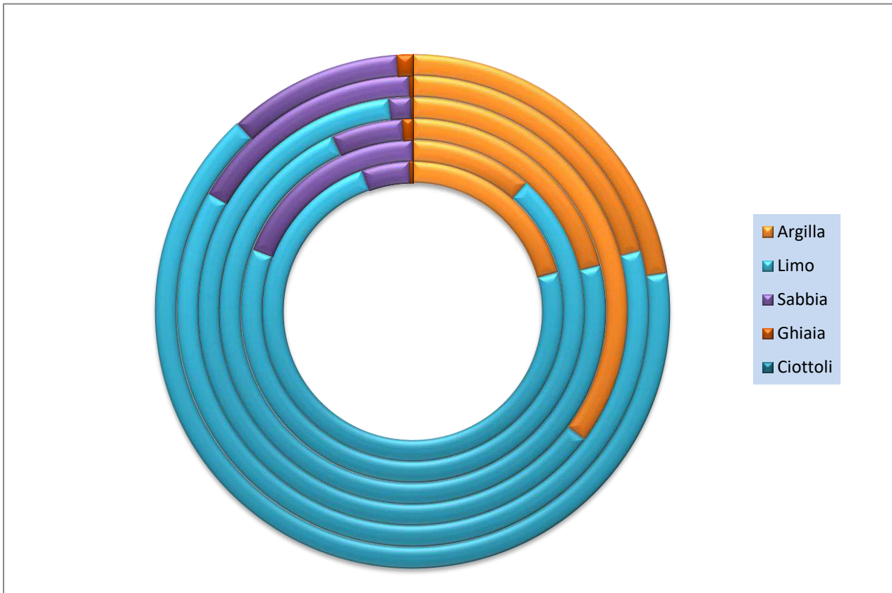
Figura 26: Rappresentazione grafica delle componenti granulometriche di tutti i campioni analizzati
