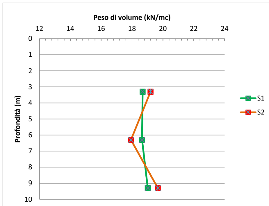
Figura 27: Andamento del peso dell'unità di volume \gamma con la profondità per tutti i campioni esaminati in laboratorio
