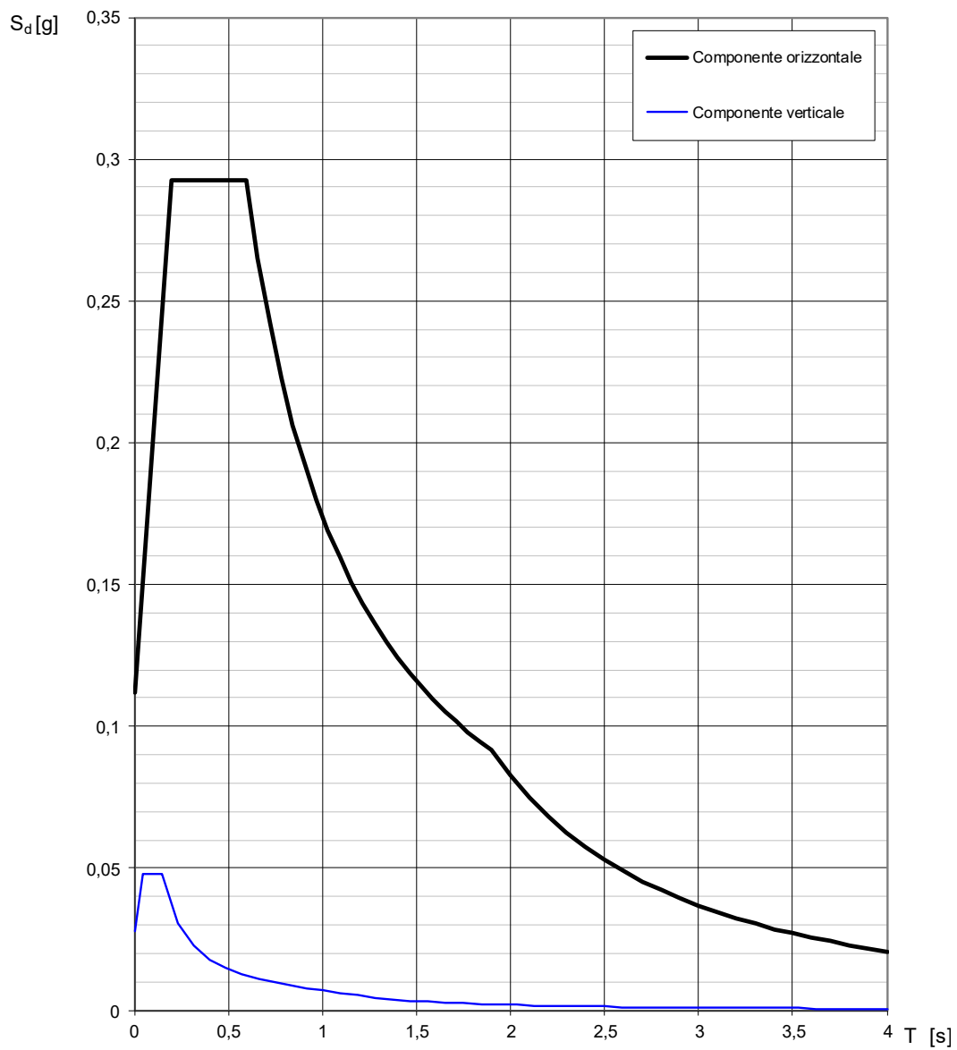
Figura 18: Spettro di risposta elastico in accelerazione per lo stato limite SLD.
