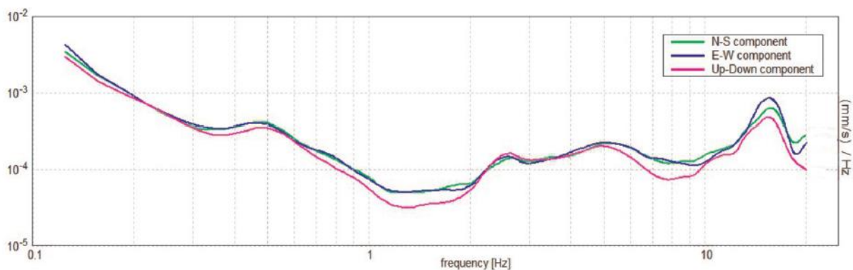
Figura 12- Andamenti degli spettri di ampiezza delle 3 componenti (N-S, E-W e V)
