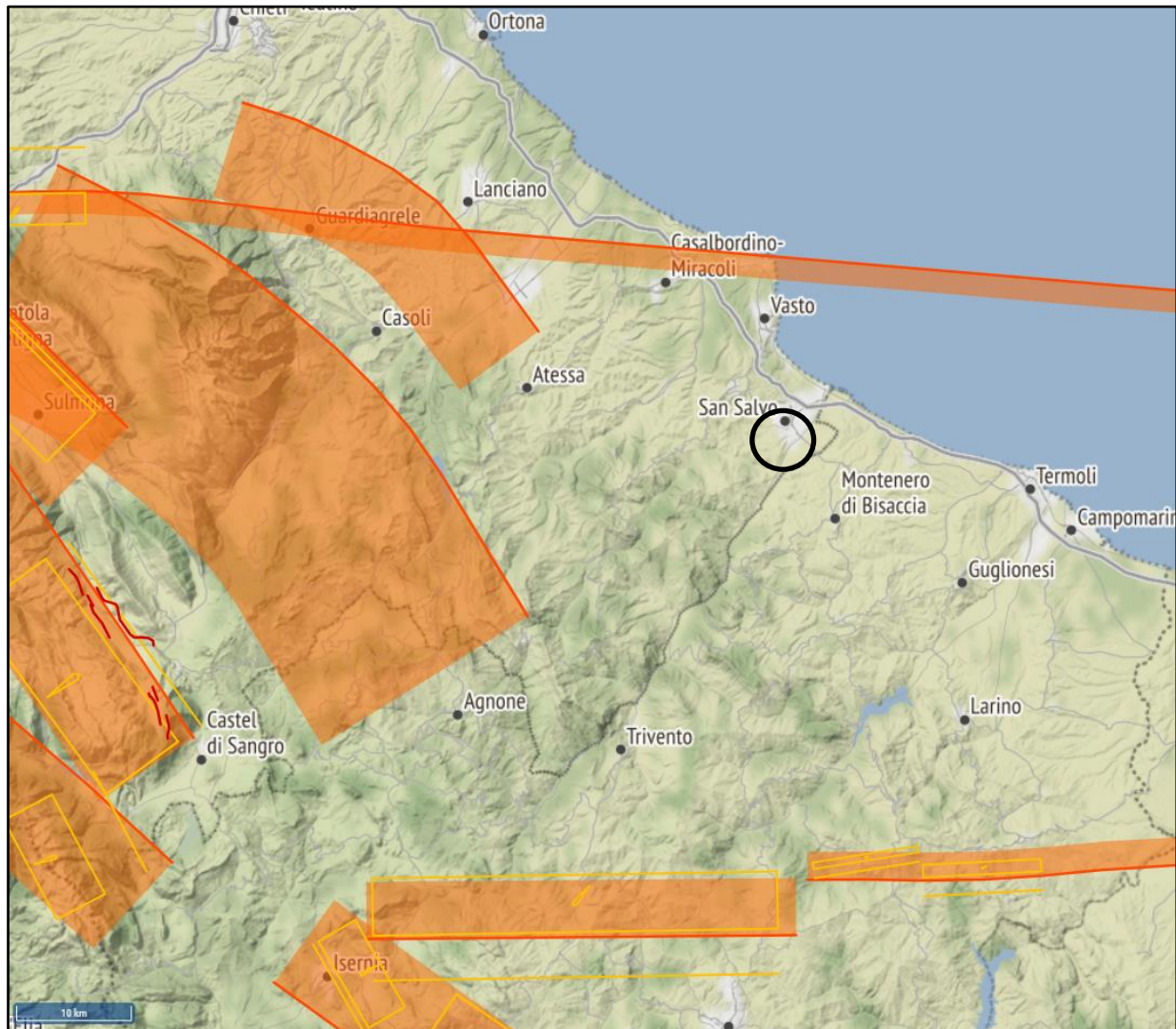
Figura 8- Le Sorgenti Sismogenetiche della Regione Abruzzo, contenute nella nuova versione del “ Database of Potential Sources for Earthquakes larger than M 5.5 in Italy ”; per l’ubicazione dell’area in esame ( DISS - Mapper (ingv.it) ).
