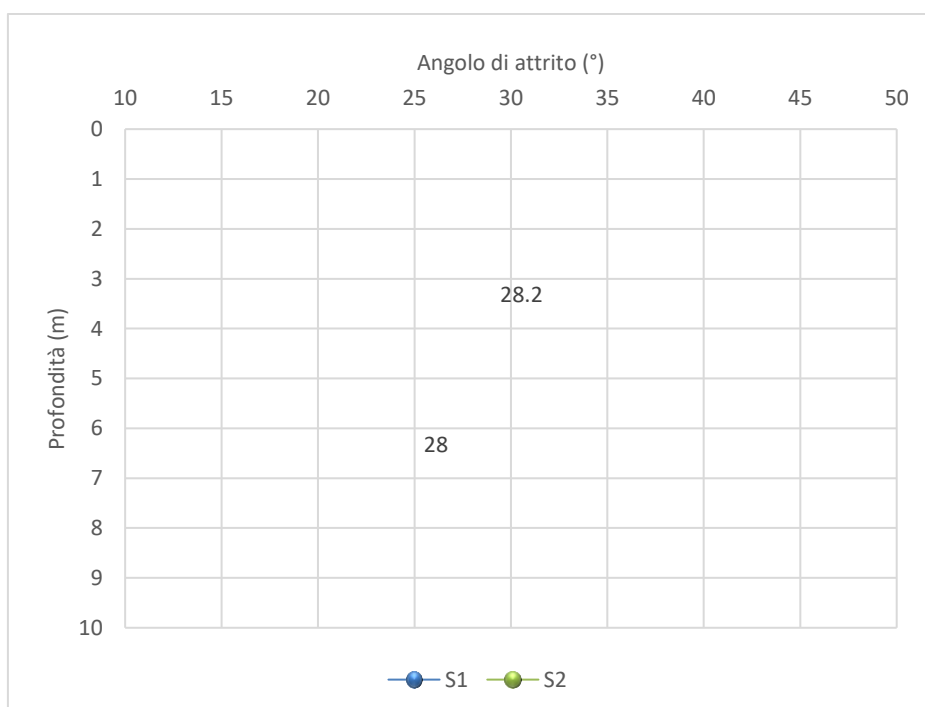
Figura 28: Dati di resistenza (angolo di attrito di picco), in condizioni drenate.
