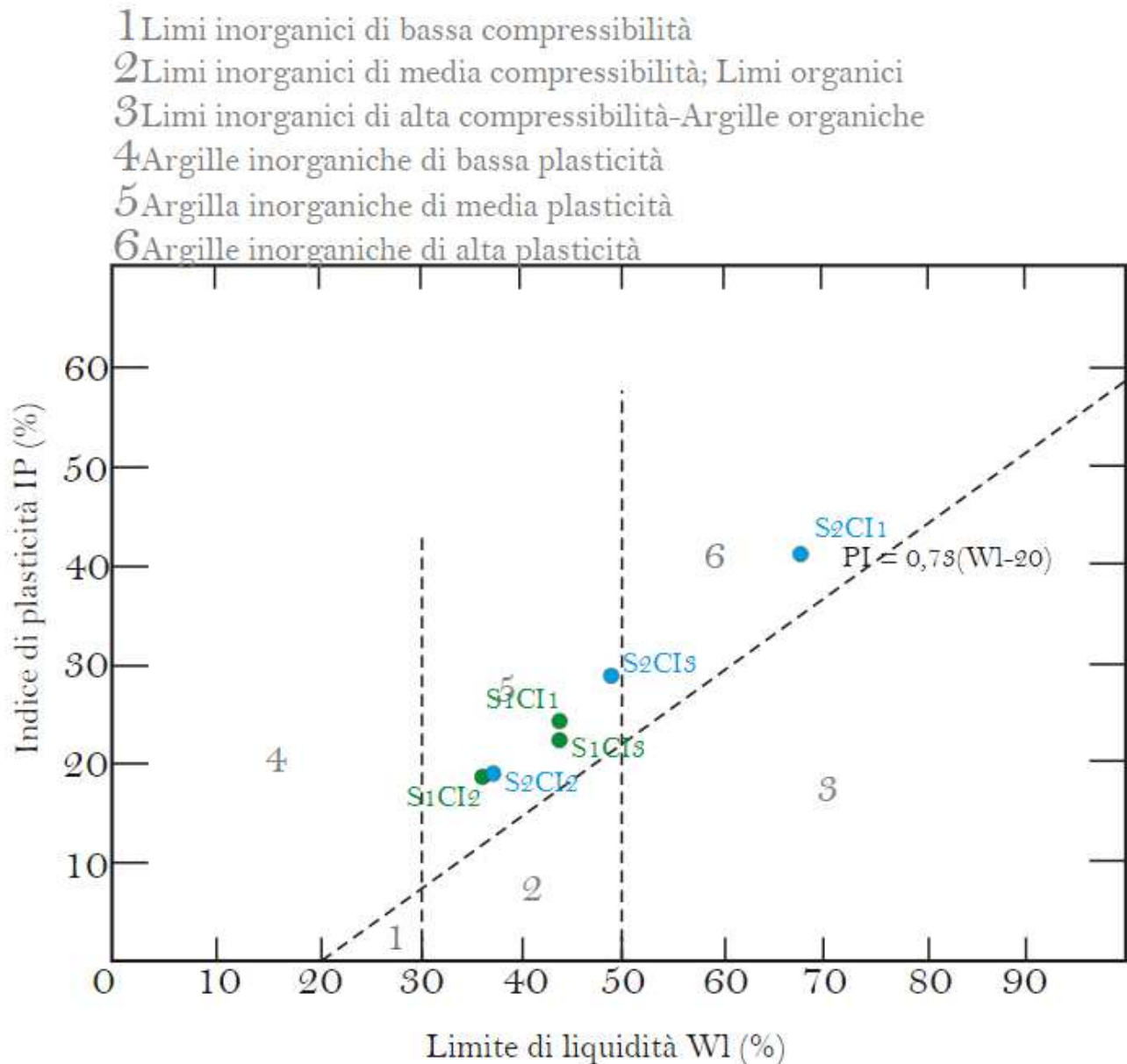
Figura 31: Carta di plasticità di Casagrande; tutti i campioni ricadono nel campo 5, ovvero “Argille inorganiche di media plasticità”, eccettuato il campione S2CI1, che ricade nel campo “Argille inorganiche di alta plasticità”.
