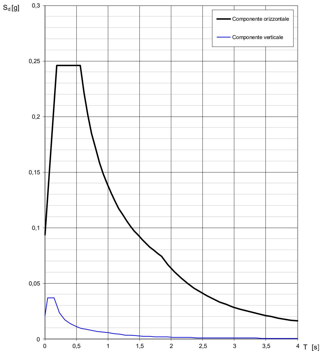
Figura 20: Spettro di risposta elastico in accelerazione per lo stato limite SLO. Tale scenario è quello meno severo, e le accelerazioni sono inferiori a 0,2 g.
