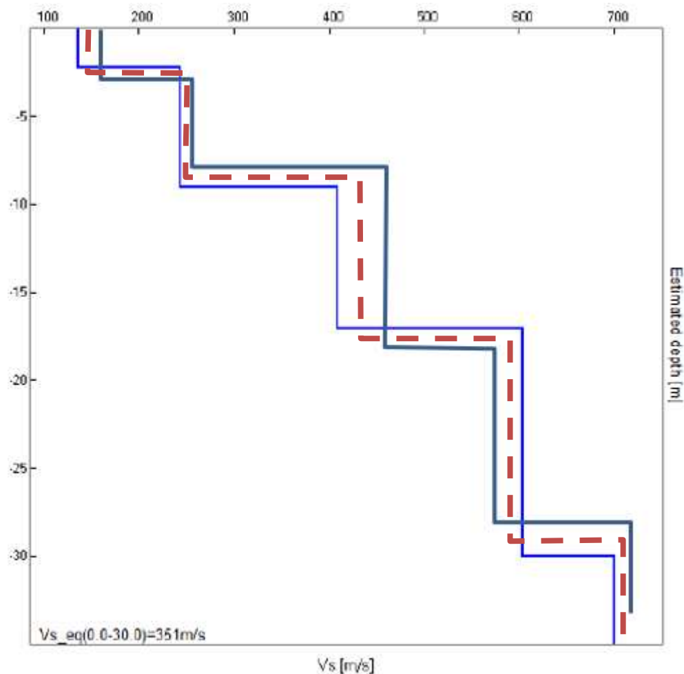
Figura 32: Confronto fra tutti i profili MASW eseguiti (in blu chiaro la MASW 1, in tono scuro la MASW 2); si nota una discreta corrispondenza dei due profili. In tratteggio rosso il profilo interpolato medio di riferimento.
