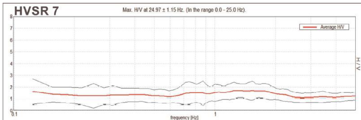
Figura 11- Curva H/V su frequenza (Hz)
