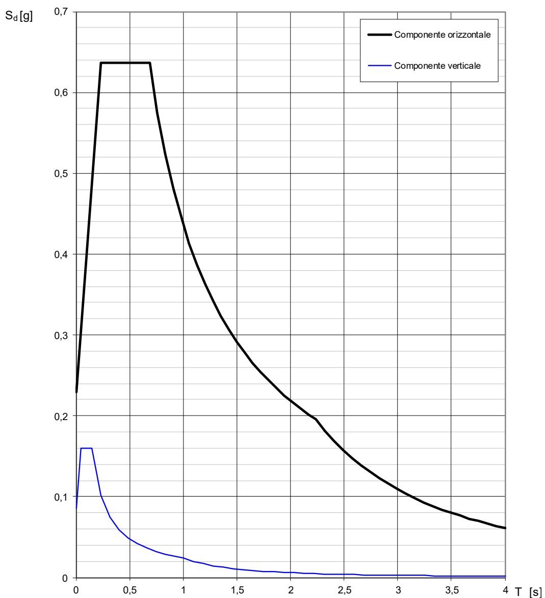
Figura 14: Spettro di risposta elastico in accelerazione per lo stato limite SLC. Si tratta dello scenario più severo, con accelerazioni che toccano 0,6 g.
