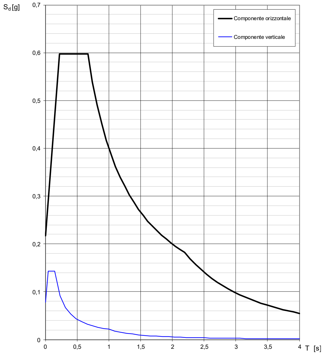
Figura 16: Spettro di risposta elastico in accelerazione per lo stato limite SLC. Tale scenario presenta accelerazioni che oltrepassano 0,5 g.
