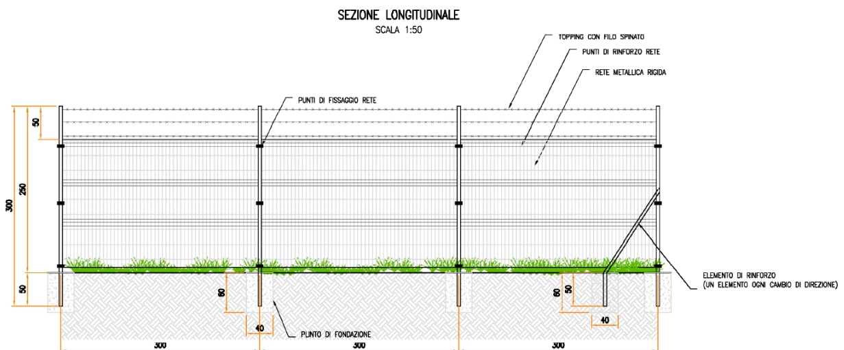
Figura 4.1: Tipico recinzione
