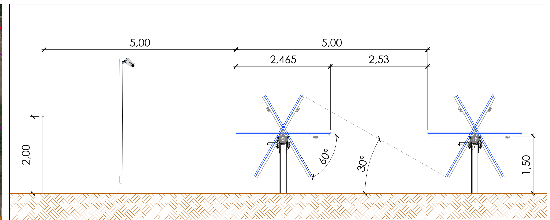
Dettaglio del tracker solare Scala 1:50
