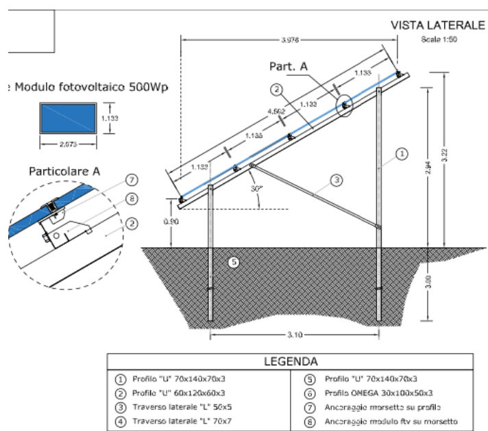
Figura 4 – Rappresentazione della struttura di supporto
