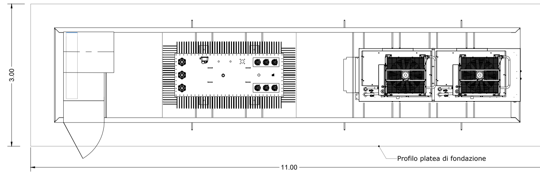
VISTA DALL'ALTO Scala 1:50
