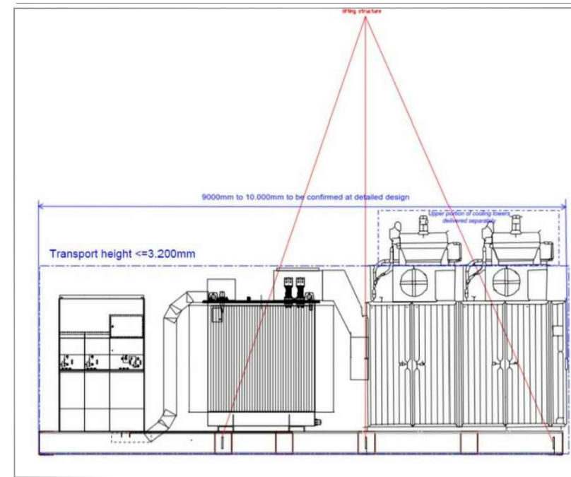
Immagine della POWER SKID
