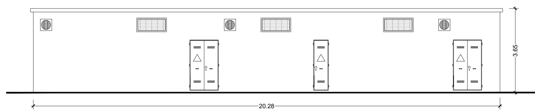
PROSPETTO B Scala 1:100
