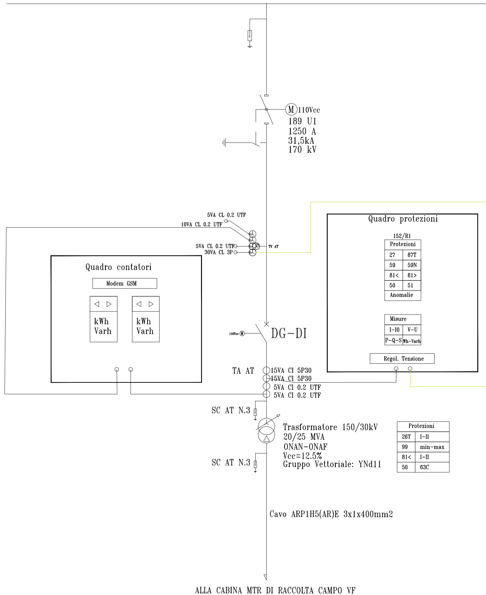
Schema Unifilare Sottostazione elettrica di trasformazione (30/150 kV) e consegna
