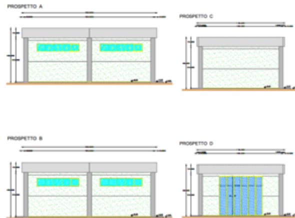
Figura 4: Prospetti edificio Magazzino
