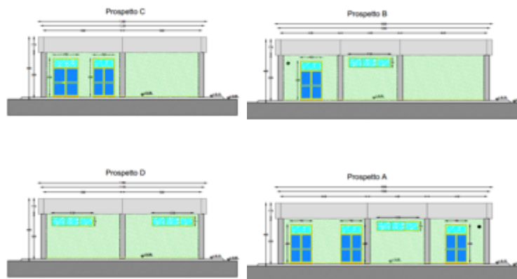
Figura 3: Prospetti edificio Servizi Ausiliari
