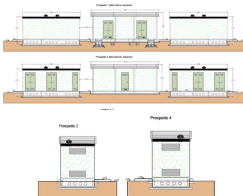
Figura 5: Prospetti edificio Consegna MT
