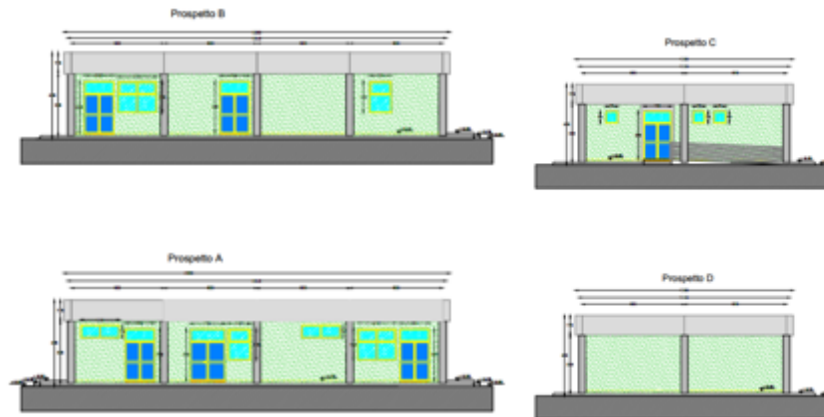
Figura 2: Prospetti edificio Comandi
