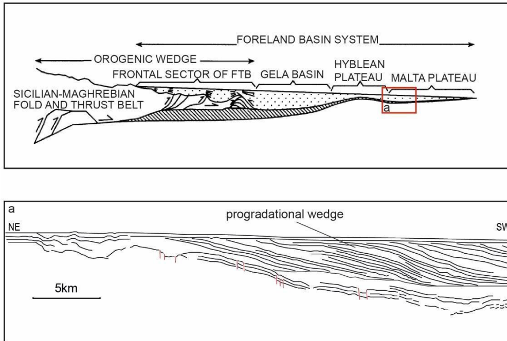
Figura 5: Modello schematico di un bacino di back-bulge (rettangolo rosso) (mod. da DeCelles e Giles, 1996). In a) il sistema di clinoformi progradati osservato nel Plateau di Malta accresciutisi all'interno del bacino di back-bulge .
