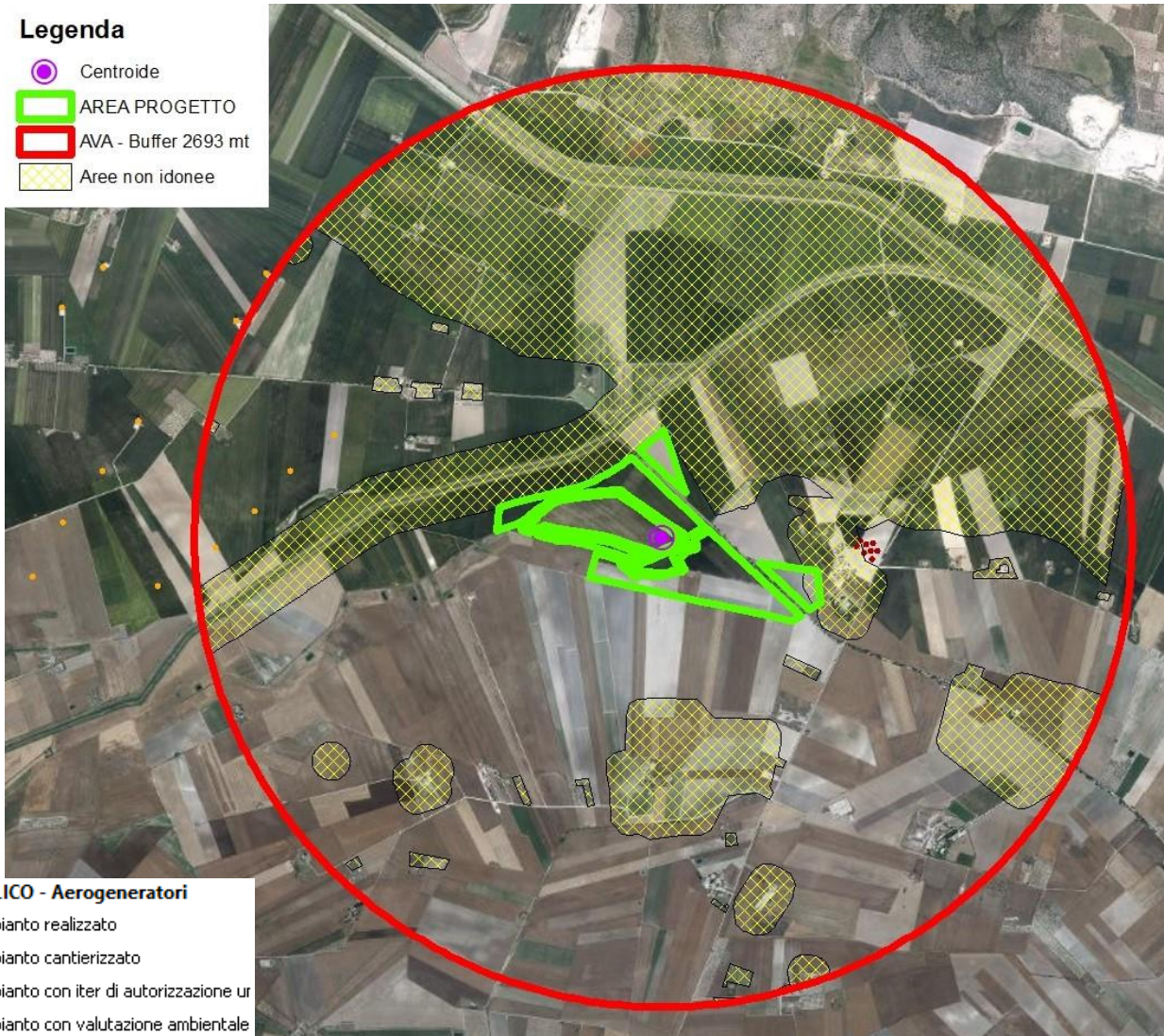
Fig. 5. Individuazione degli impianti eolici presenti nell'area del dominio.
