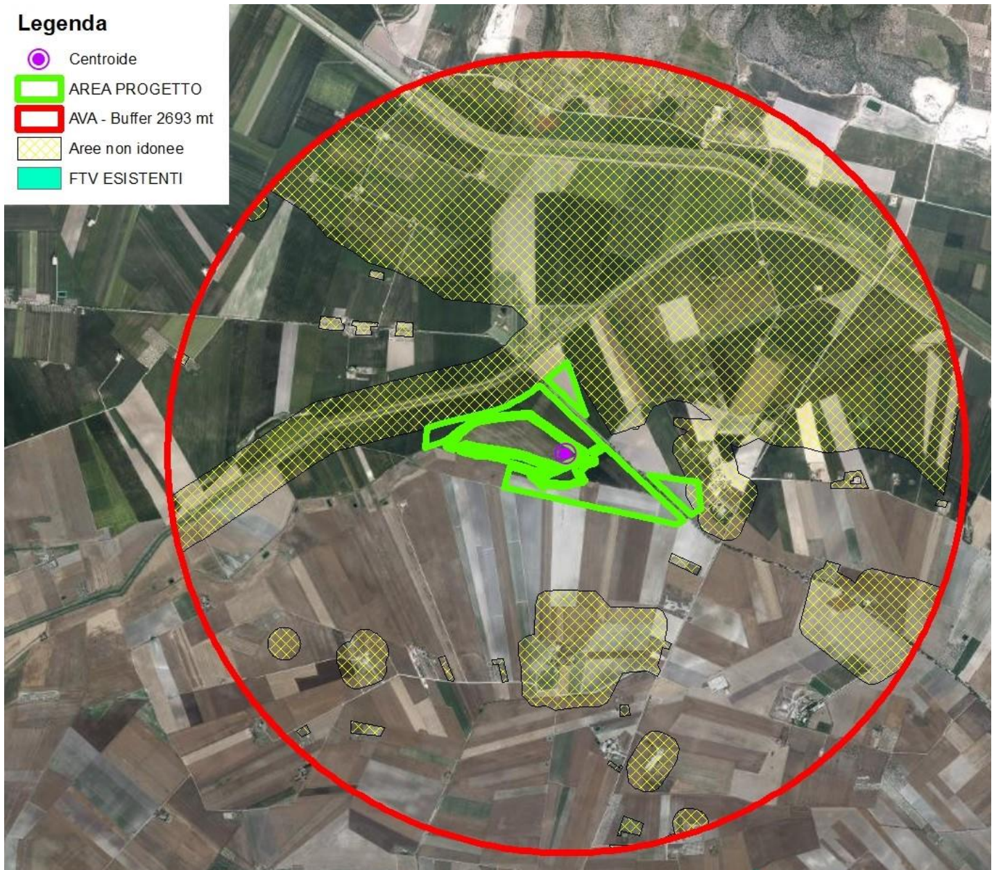
Fig. 4. Individuazione dell'area data da RAVA, delle aree non idonee e degli impianti del dominio.
