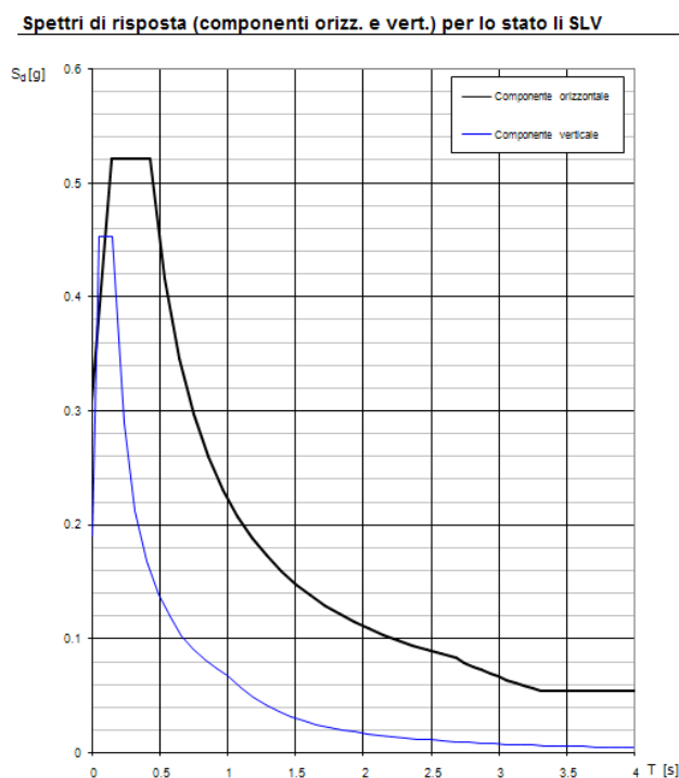
Figura 2.1: Spettri di risposta (componenti orizz. e vert.) per lo stato limite:SLV
