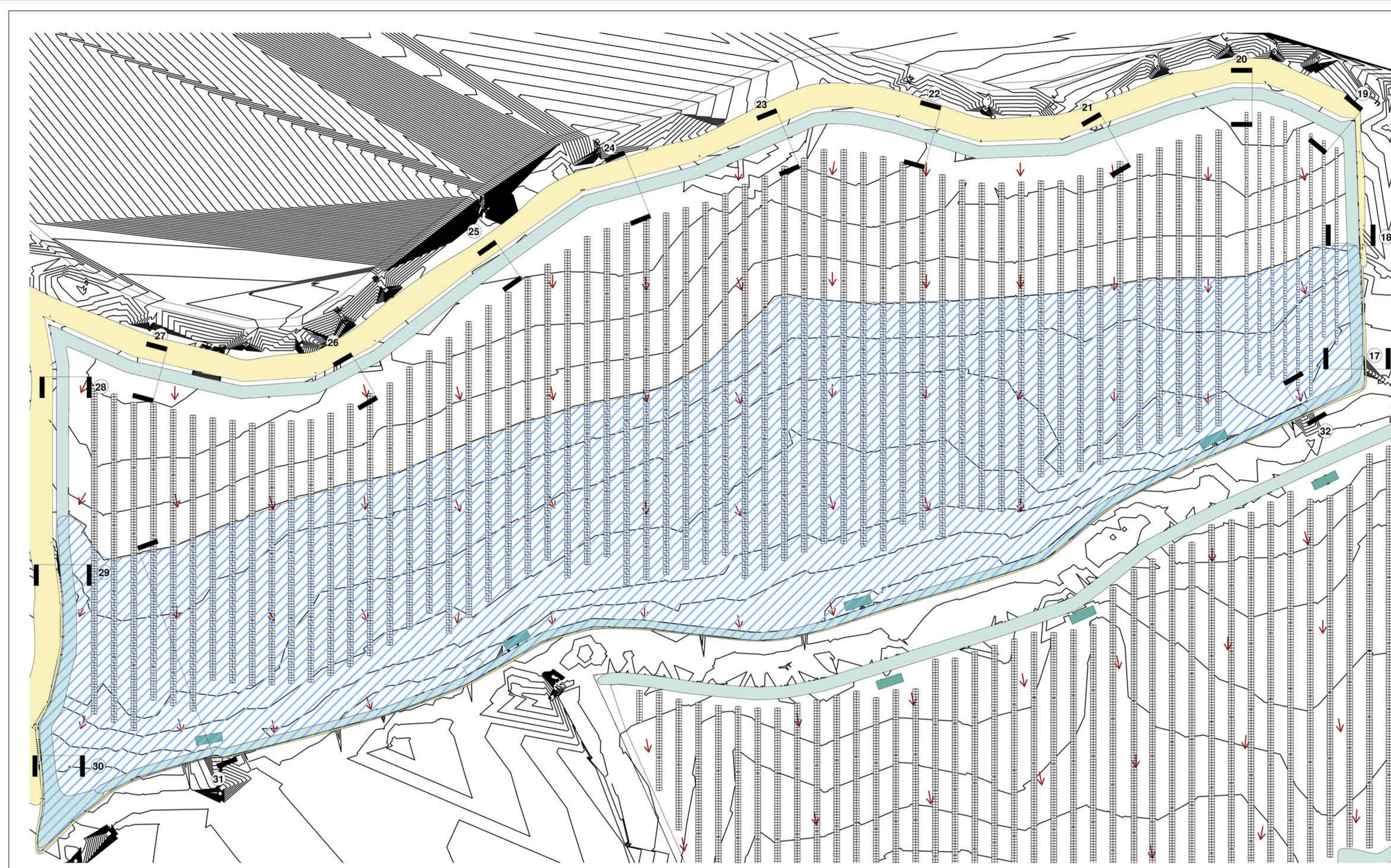
1 Planimetria B - 1.1000 1:1000 ■ Profondità scavo 0-50 cm ■ Profondità scavo 50-100 cm ■ Profondità scavo 200 cm ■ Mitigazione con argine ■ Mitigazione con argine ↑ Direzione scolo acqua
