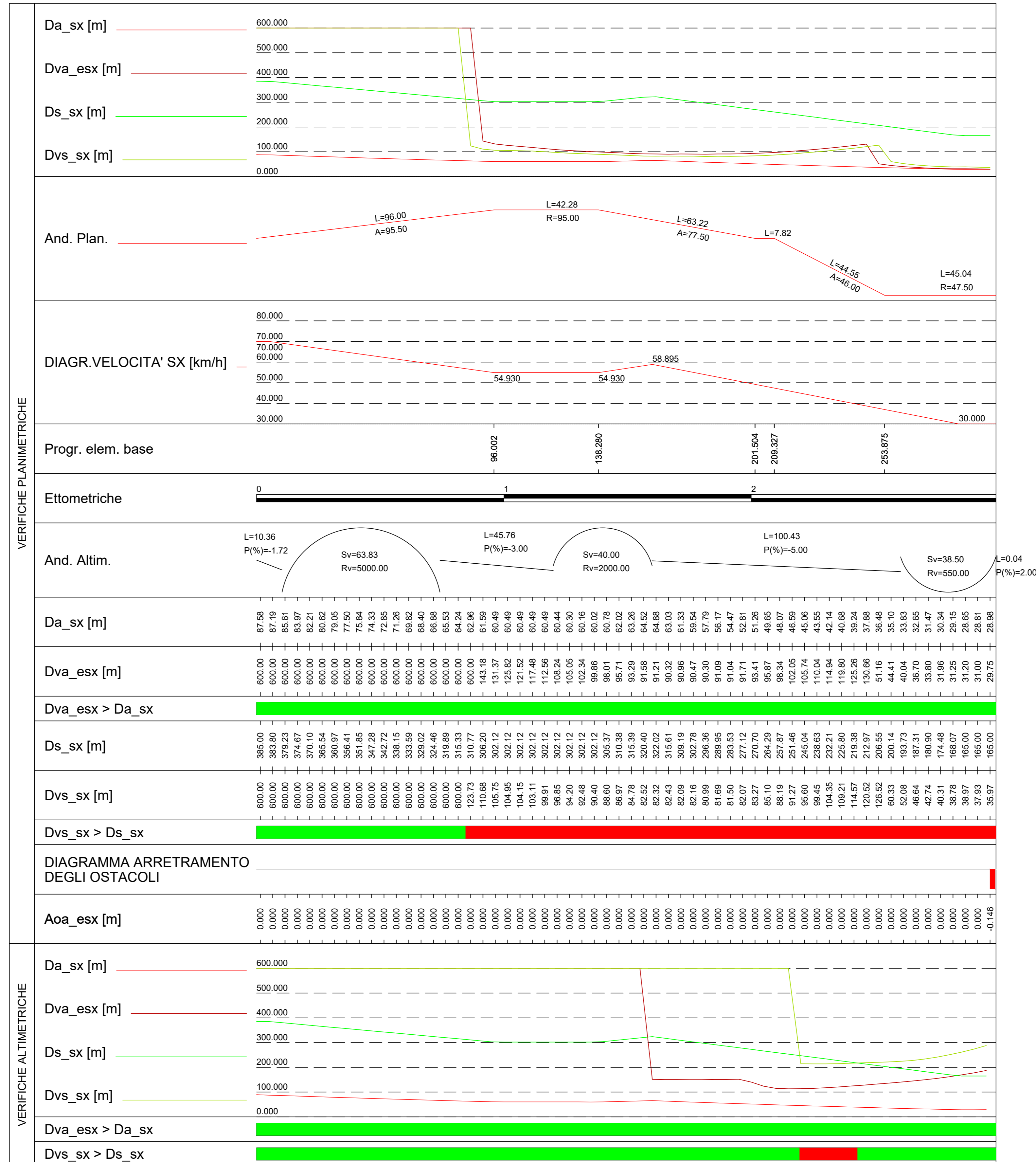
DIAGRAMMI DI VISIBILITA' - RITORNO Scala X 1:1000.000 Scala Y 1:1000.000
