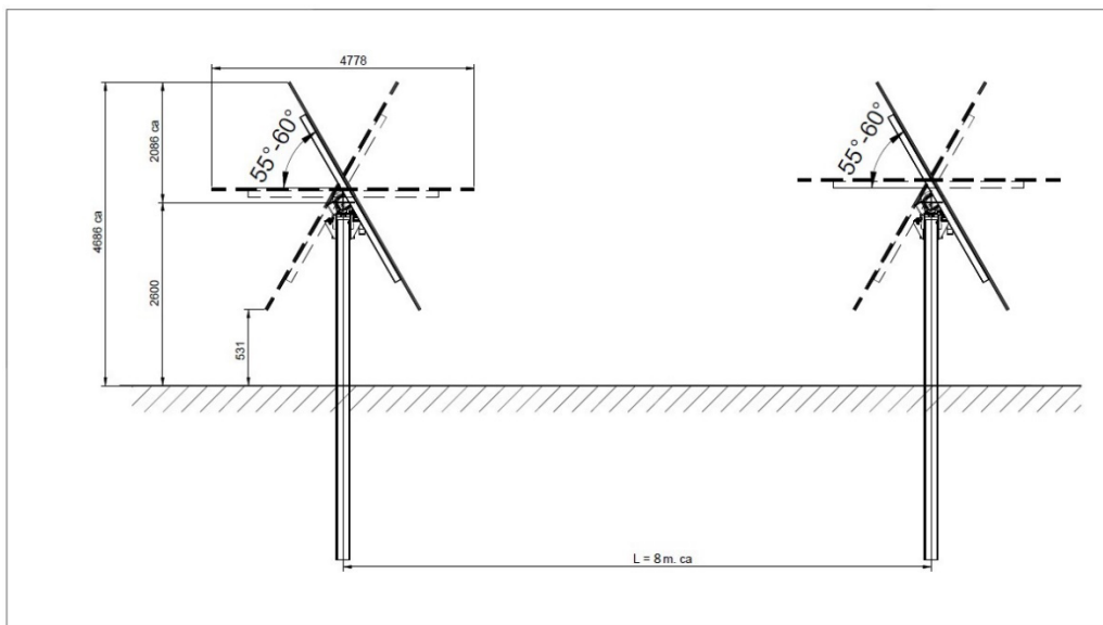
55 – tracker - particolare del pitch e altezza dal suolo
