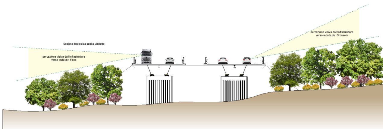
Figura 15 - Sezione tipologica mitigazione vegetazionale spalla viadotto/piede scarpata e ricucitura con la vegetazione esistente
