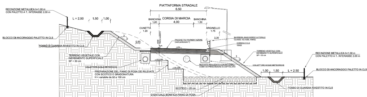
Figura 4 – Sezione tipo di rampa monodirezionale a mezzacosta in rettililo
