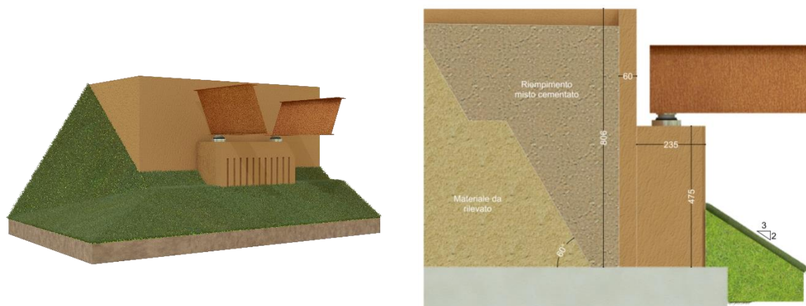
Figura 5: Modello 3d tipologico della spalla e sezione tipologica della spalla
