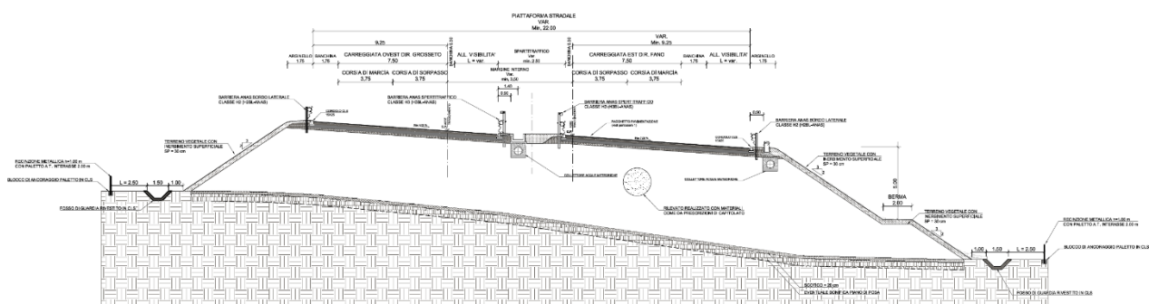
Figura 2 – Sezione tipo in rilevato in curva con allargamento
