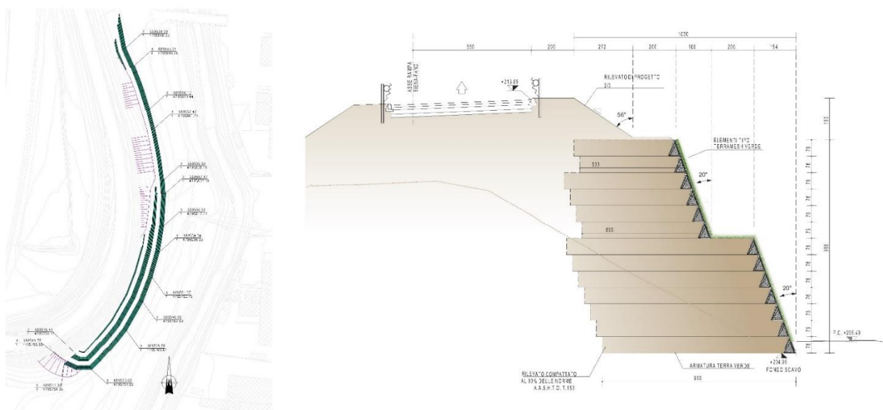
Figura 17 - Pianta e sezione dell'intervento in terra rinforzata con paramento rinverdito
