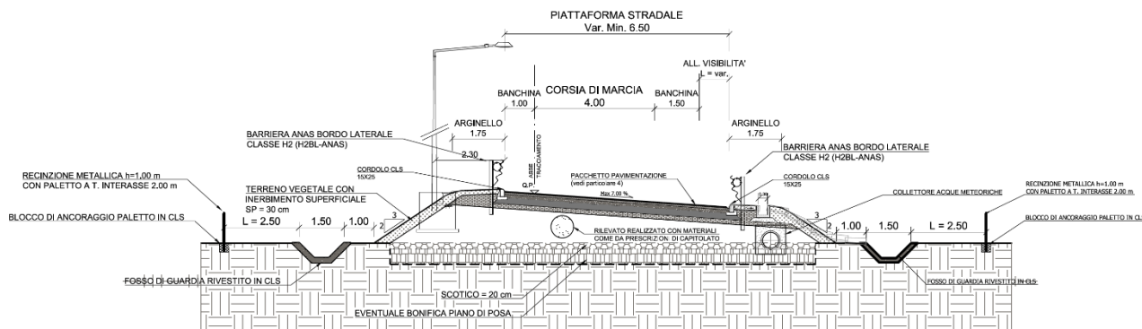
Figura 14 – Sezione tipo di rampa monodirezionale in rilevato in rettililo
