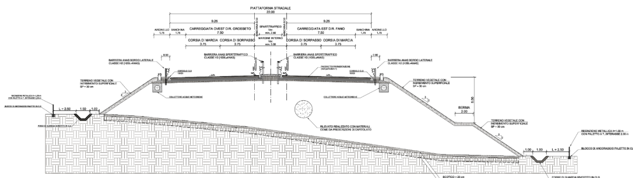
Figura 1 – Sezione tipo in rilevato in rettilineo
