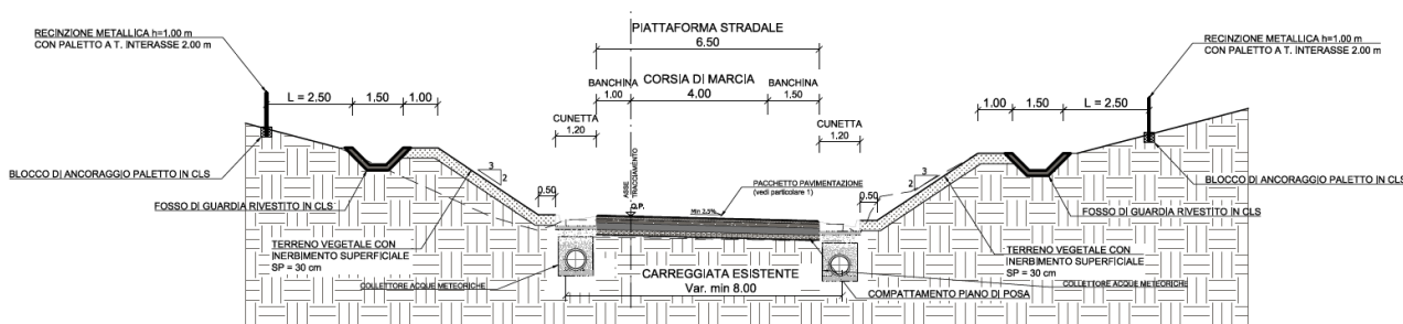
Figura 15 – Sezione tipo di rampa monodirezionale in trincea in rettilo
