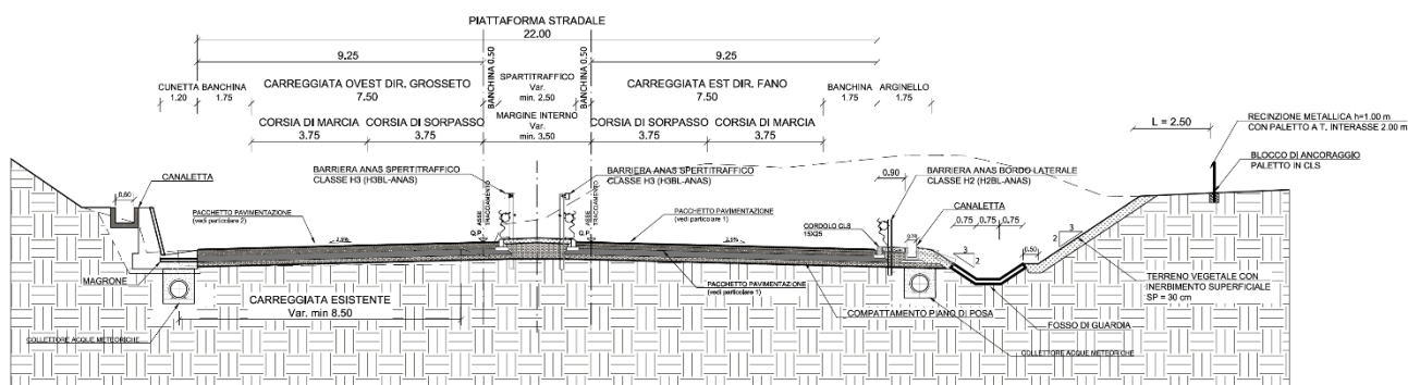
Figura 9 – Sezione tipo in trincea in rettilo con scavo laterale e muro a margine
