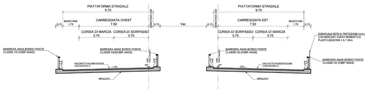
Figura 12 – Sezione tipo in viadotto in rettilo
