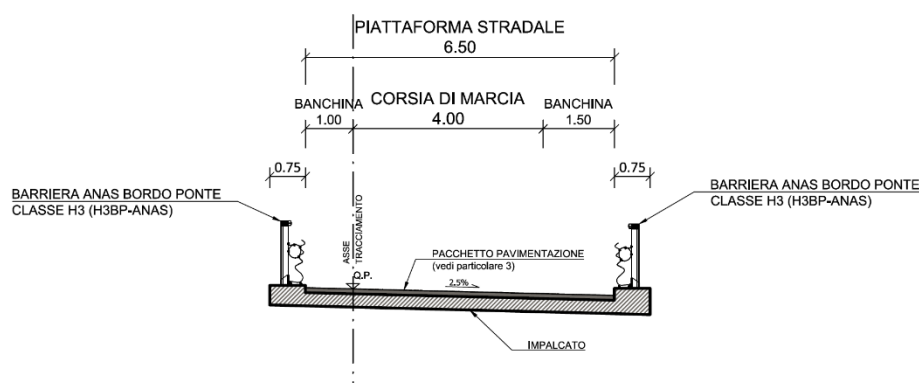
Figura 5 – Sezione tipo di rampa monodirezionale in viadotto in rettilo
