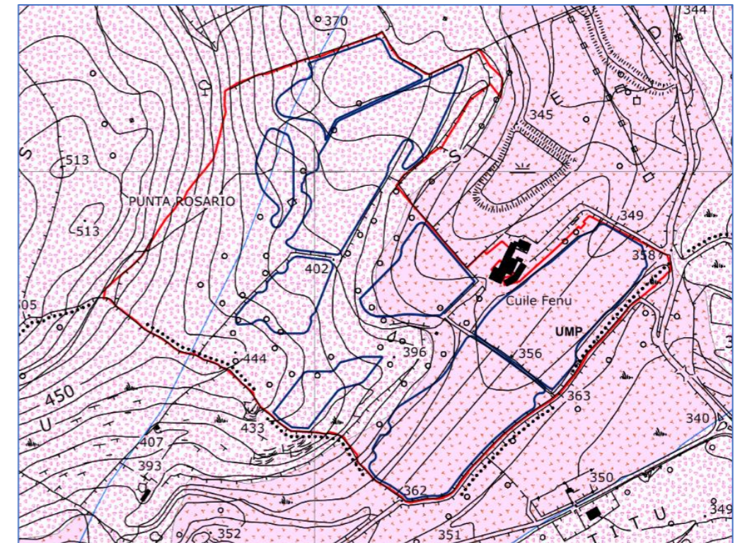
SEZIONE 6 - AREA SUD CARTA GEOLOGICA Scala 1:5.000
