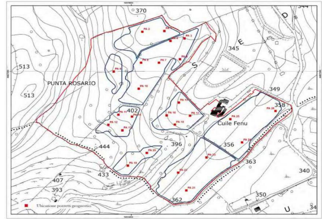
Area Sud – ubicazione dei pozzetti geognostici
