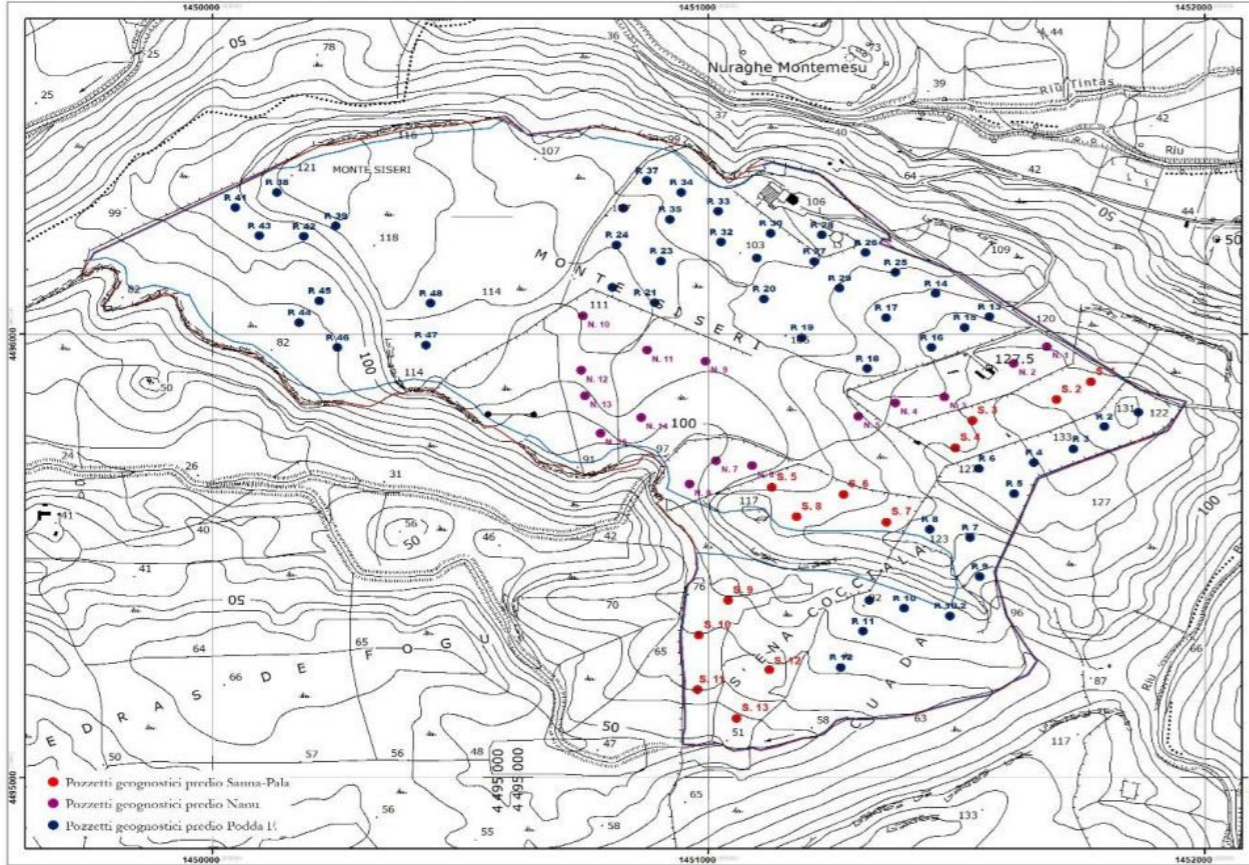
Area Nord – ubicazione dei pozzetti geognostici
