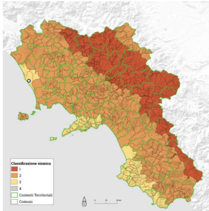
Classificazione sismica
