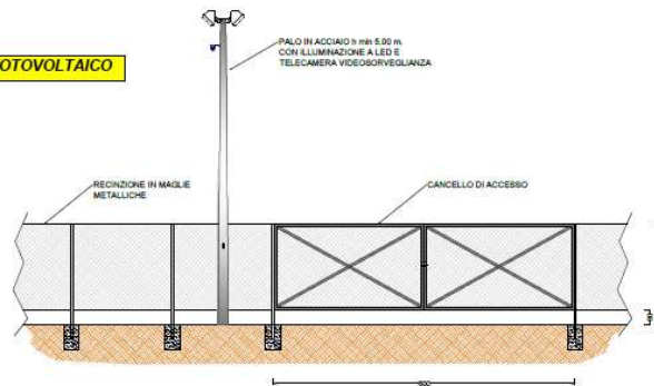
Particolare Recinzione
