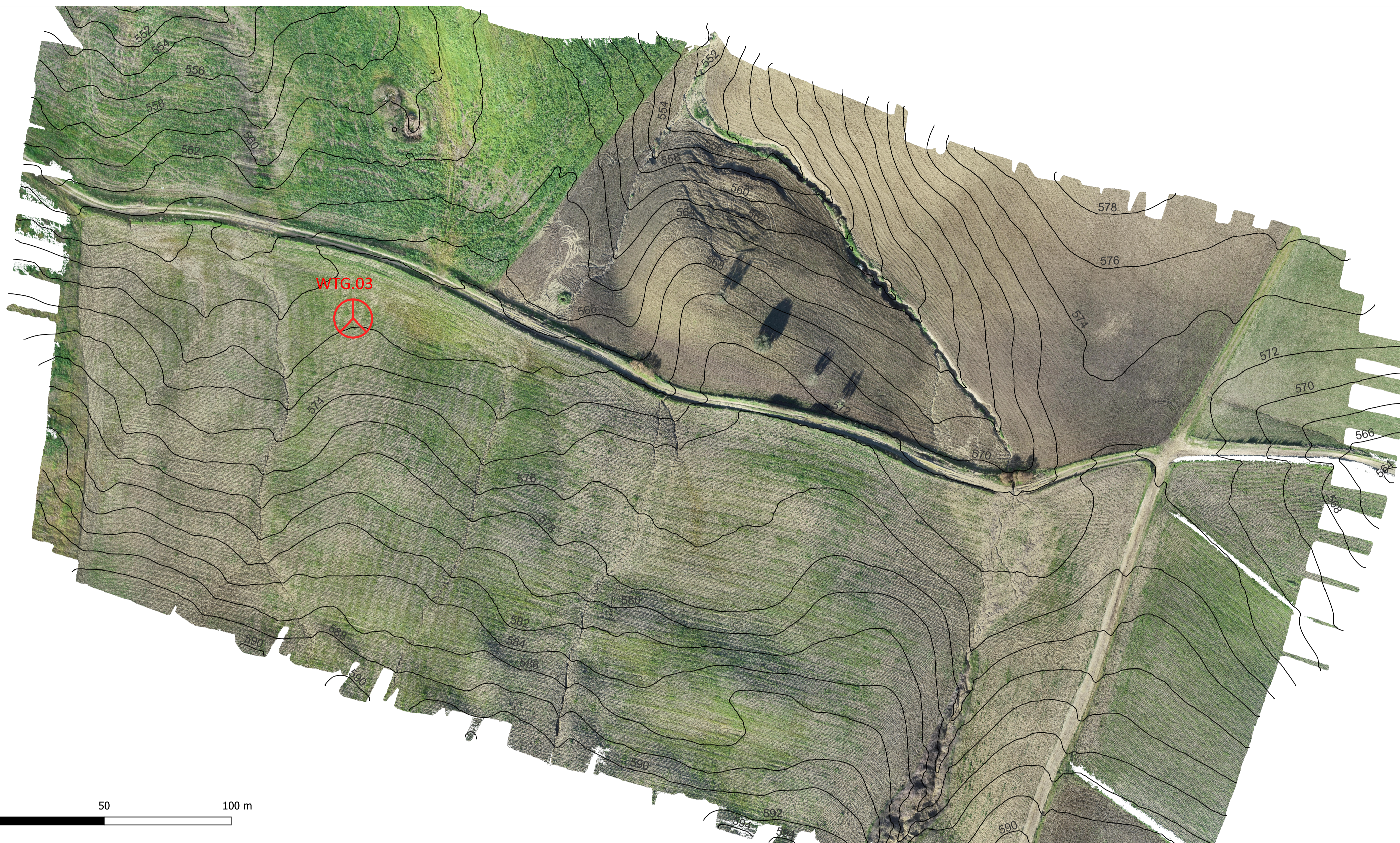
AREA WTG.03 ORTOFOTO DA RILIEVO DRONE CON CURVE DI LIVELLO risoluzione foto 15 cm/pixel - risoluzione DTMcm/pixel
