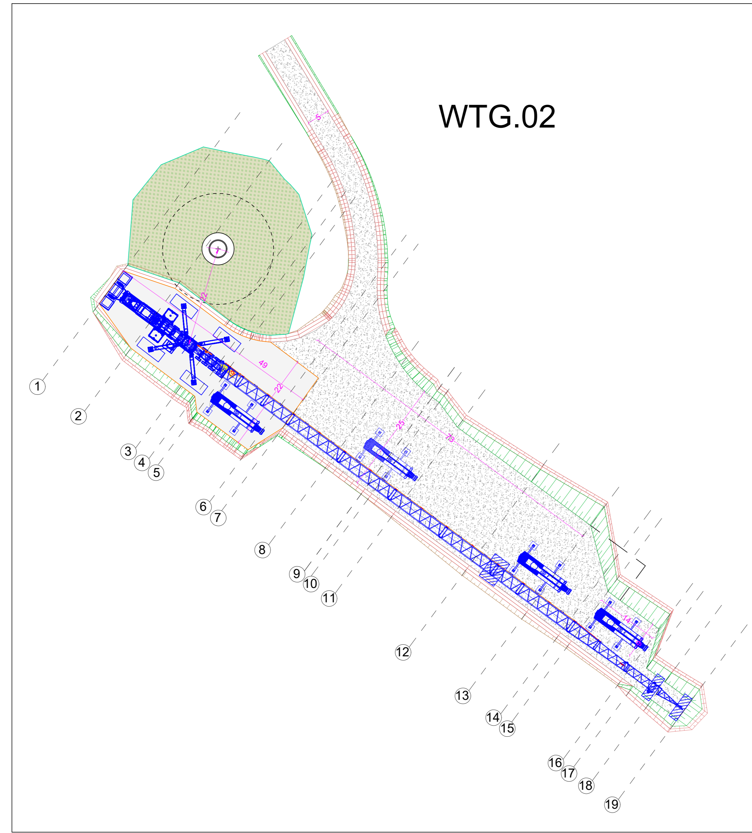
CONFIGURAZIONE 2 - MONTAGGIO GRU TRALICCIATA - SCALA 1:500
