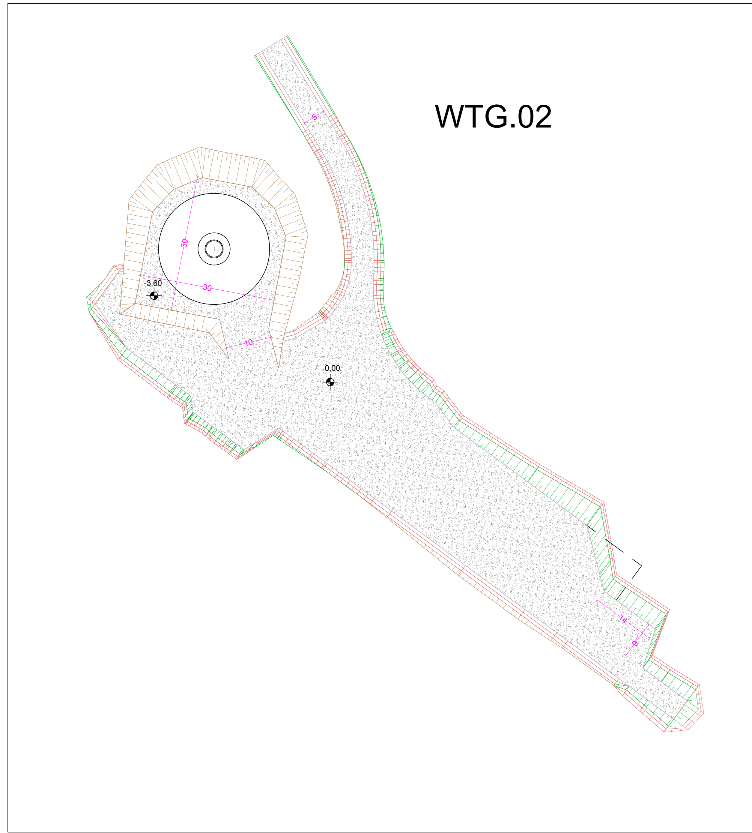
CONFIGURAZIONE 1 - SCAVO DI FONDAZIONE - SCALA 1:500
