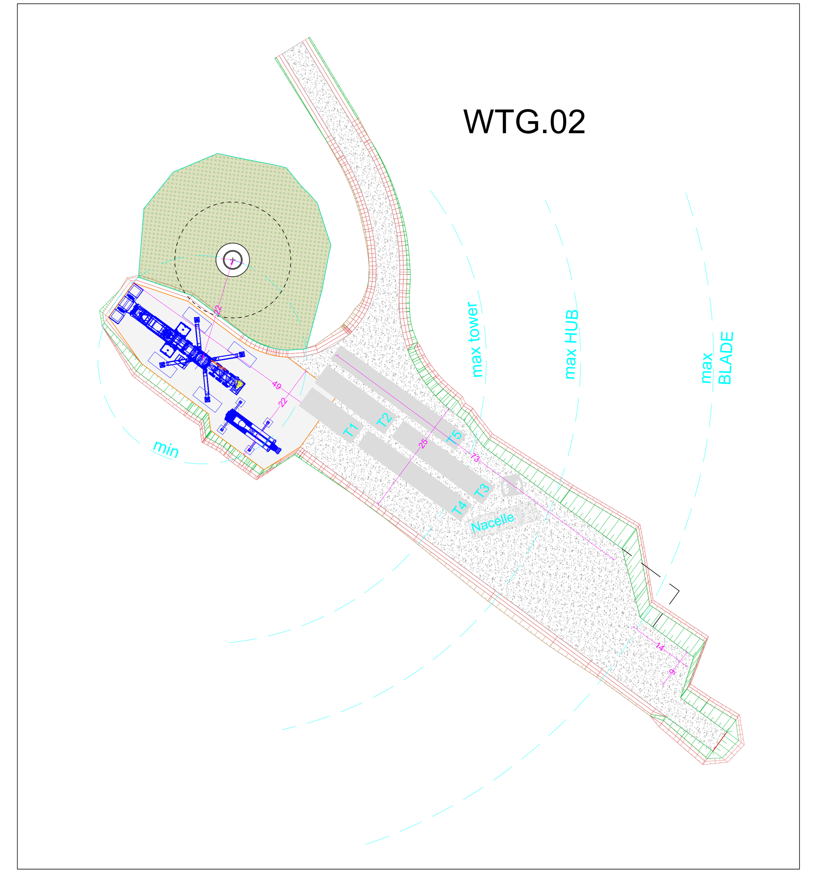
CONFIGURAZIONE 3 - MONTAGGIO TRAMI E NAVICELLA - SCALA 1:500
