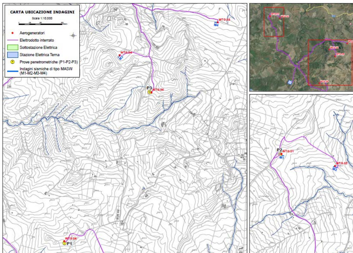
Fig. 9– Ubicazione prove in situ, su base c.t.r.
