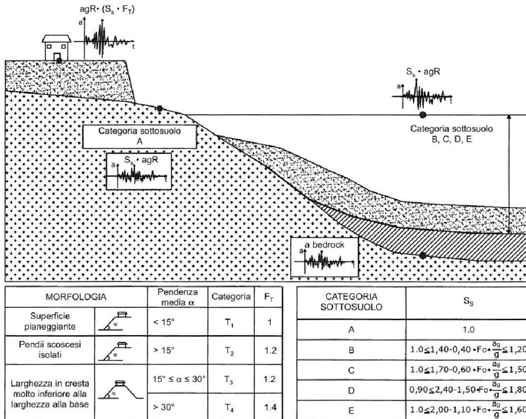
Fig. 16 - Rappresentazione schematica del significato delle accelerazioni, delle classi di categoria di suolo e del fattore topografico (da Microsism - procedure automatiche di microzonazione sismica, Giulio Riga)
