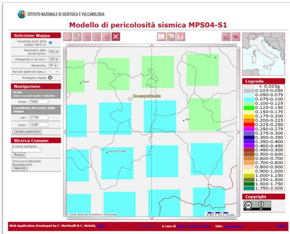
Fig. 15 - Stralcio della mappa interattiva di pericolosità sismica dei territori di Roccapalumba, Lercara Friddi e Castronovo di Sicilia. I punti visualizzati si riferiscono a: parametro dello scuotimento a(g) ; probabilità di superamento del 10% in 50 anni.
