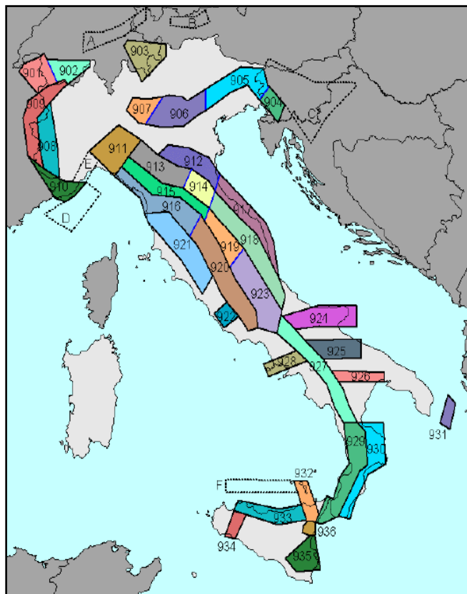
Fig. 13 - Zonazione Sismogenetica ZS9
