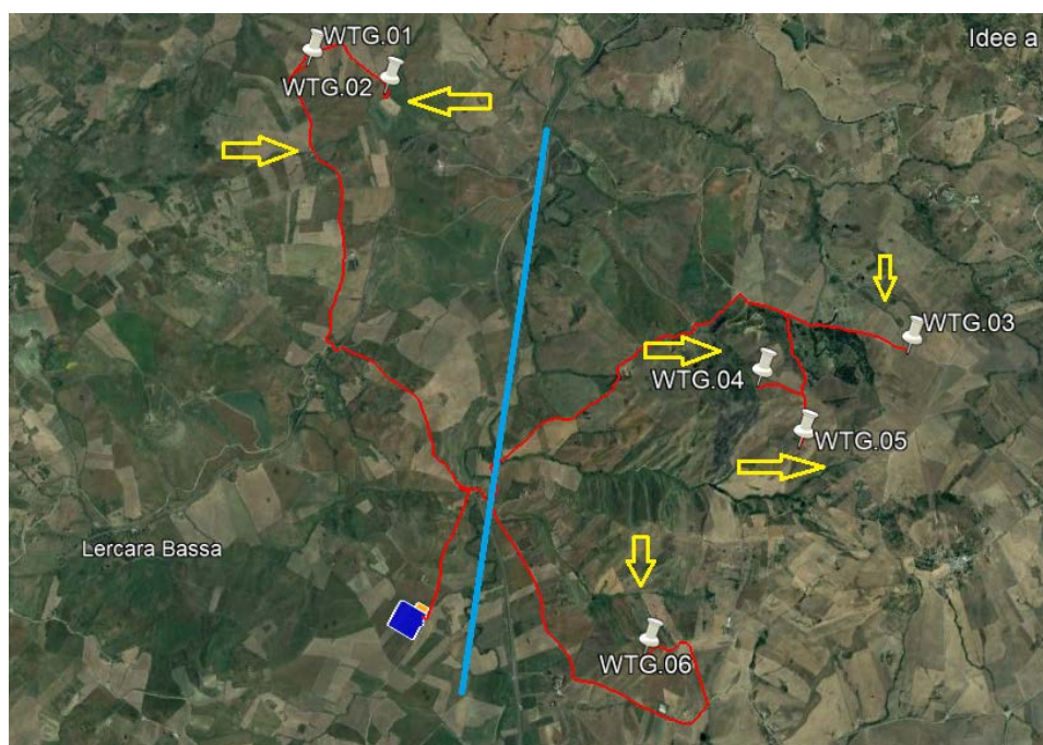
Fig. 6 – L'immagine indica l'ubicazione degli aerogeneratori (segnaposto binchi), cavidotto (segmento rosso) e sottostazione elettrica (poligoni blu e giallo) su base ortofoto; si evidenzia la presenza di numerose piccole aste (freccie gialle) di bassissimo ordine gerarchico che hanno solcato il rilievo favorendo la formazione di numerose creste morfologiche e picchi isolati; il segmento azzurro indica l'asse principale del Torrente Torto .
