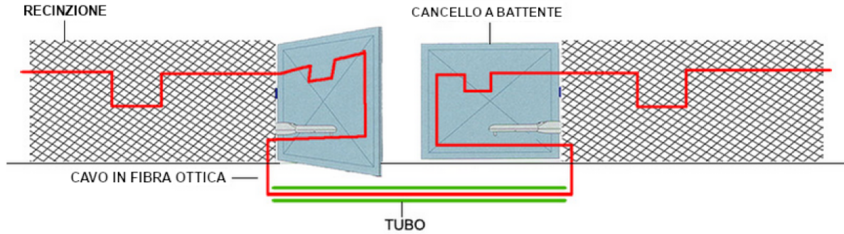
Figura 4.9 – Schema di installazione cavo in fibra ottica su recinzione.
