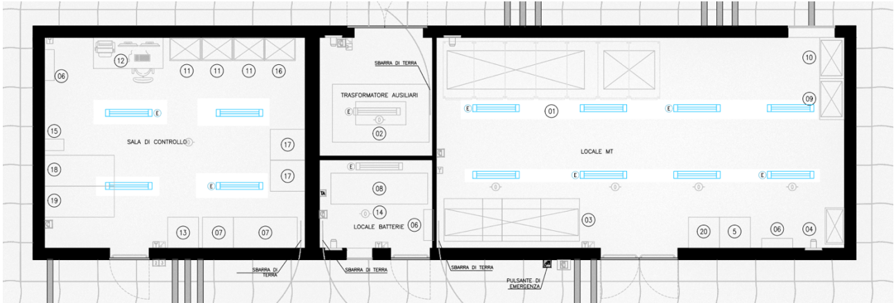
Figura 4.5 – Posizionamento plafoniere Cabina BT/MT.
