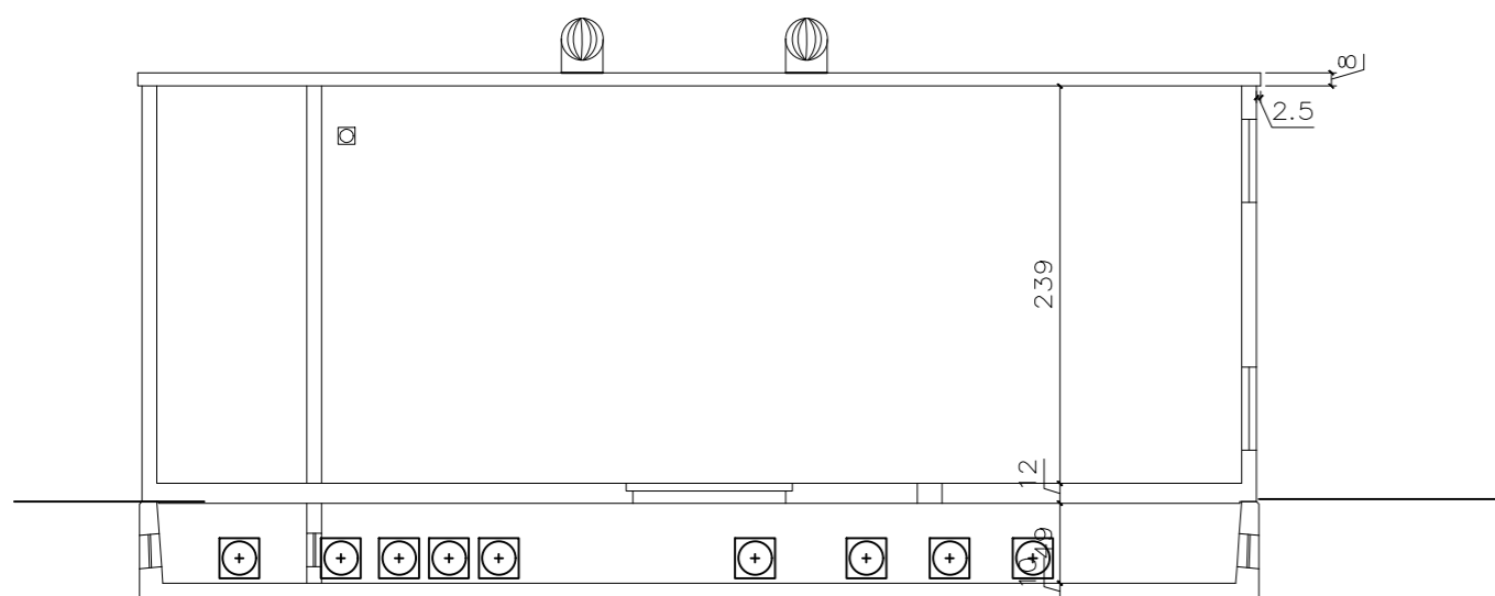
sezione X-X
