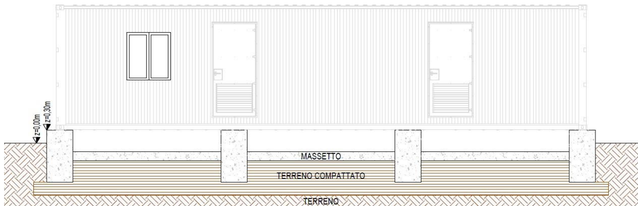
Figura 7 - Cabina MT di smistamento - Vista esterna e fondazioni
