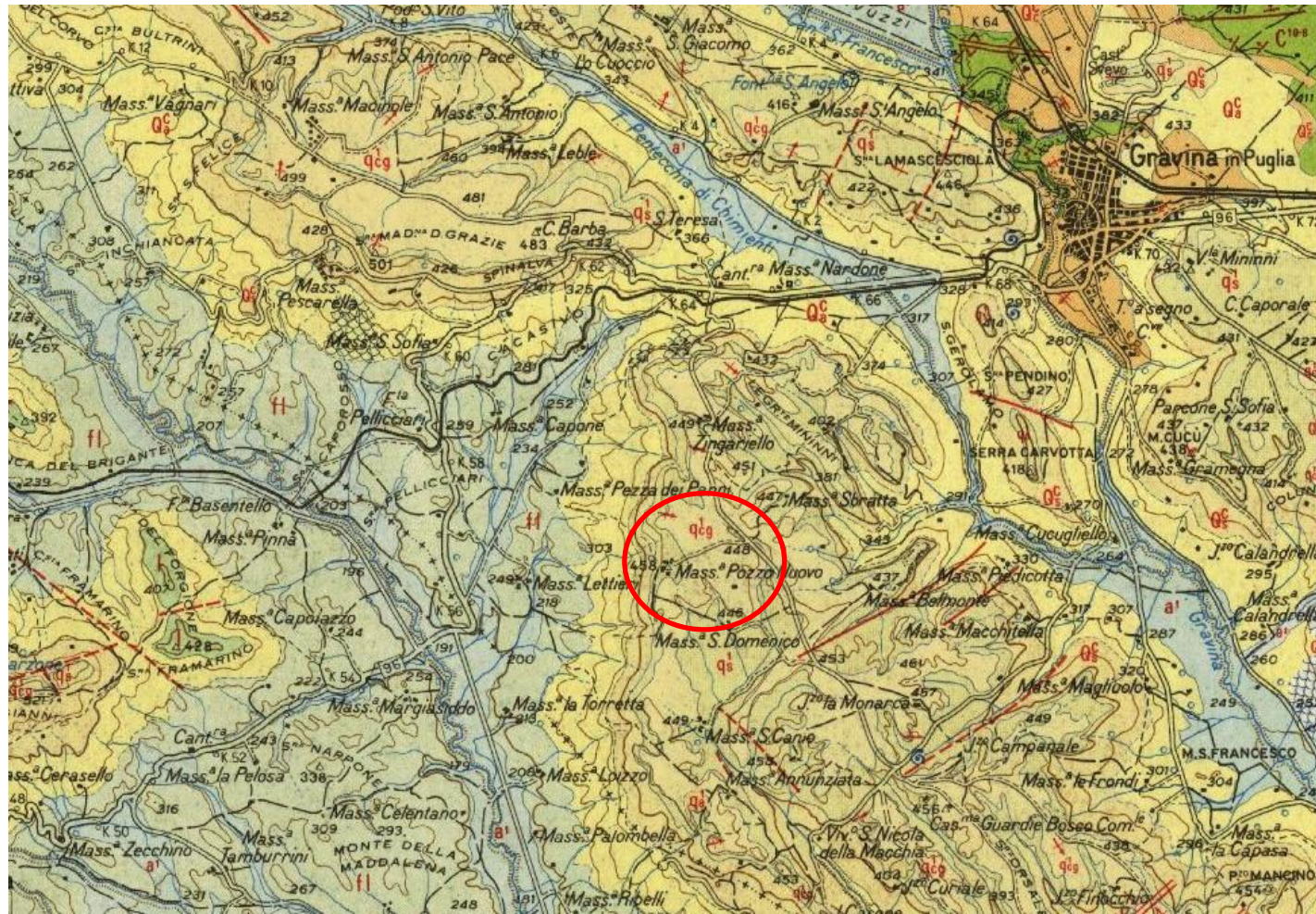
Figura 8: Stralcio del Foglio 188 della Carta Geologica D'Italia
