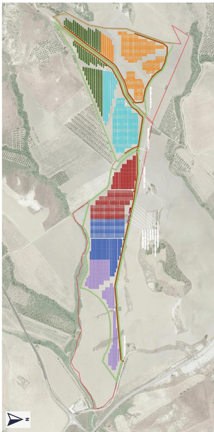
Fig.2 - Lay-out del parco fotovoltaico in località Montagnola
