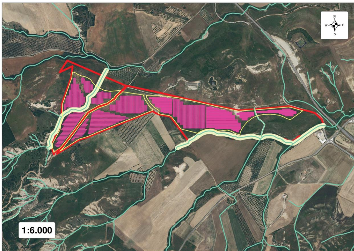
Figura 8 – Area di pertinenza del progetto con indicazione dell'ubicazione dei pannelli fotovoltaici, della recinzione perimetrale, dell'idrologia superficiale e delle aree inondabili.
