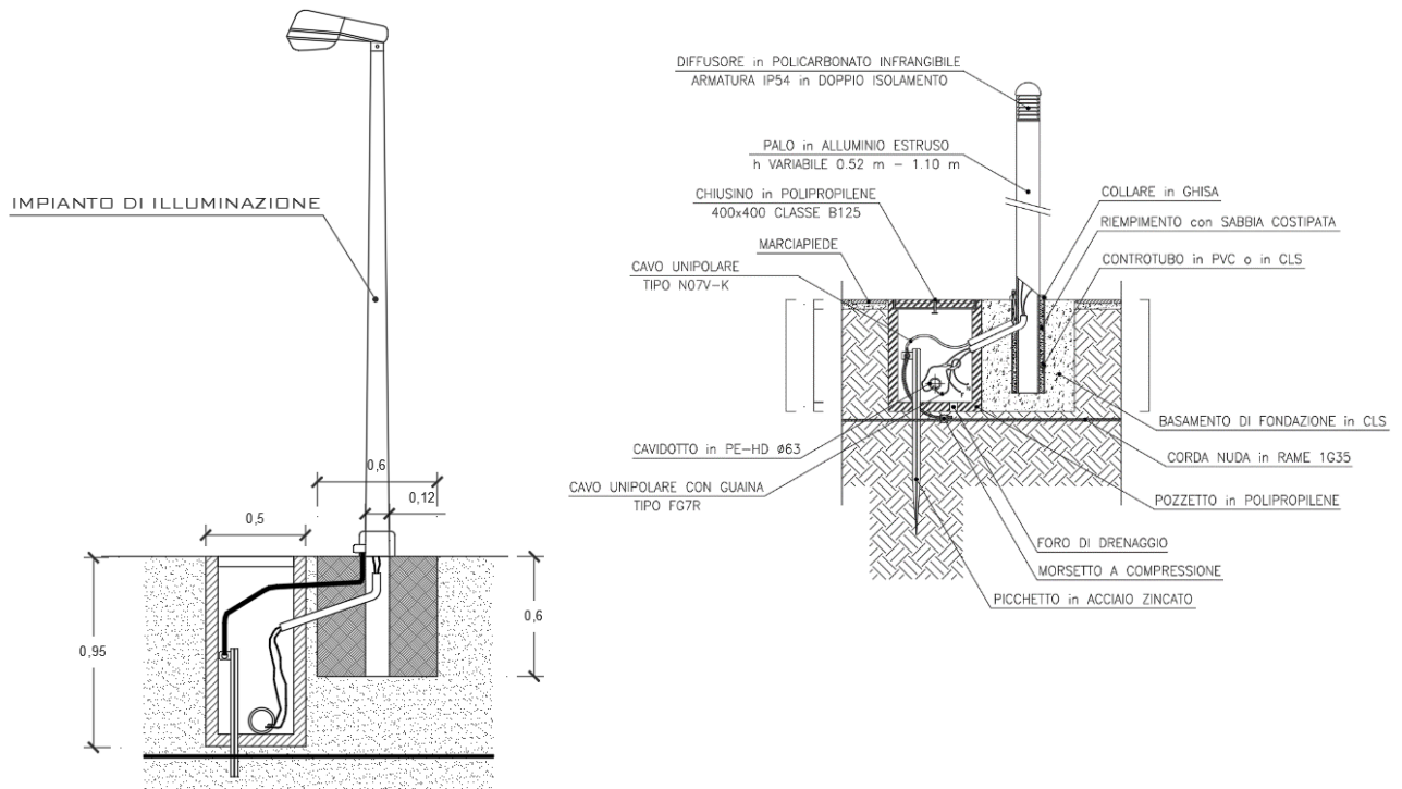
Fig. 20 – Sistema di illuminazione
