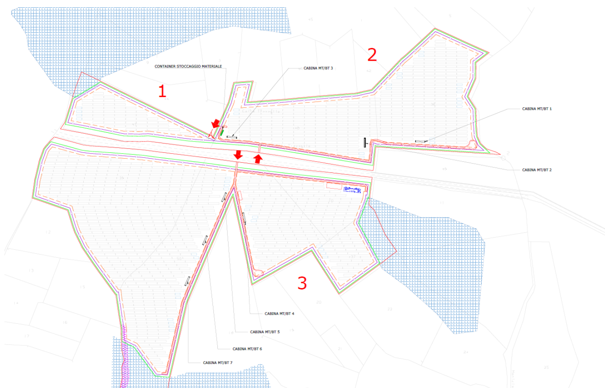
Fig. 3 - Layout di impianto
