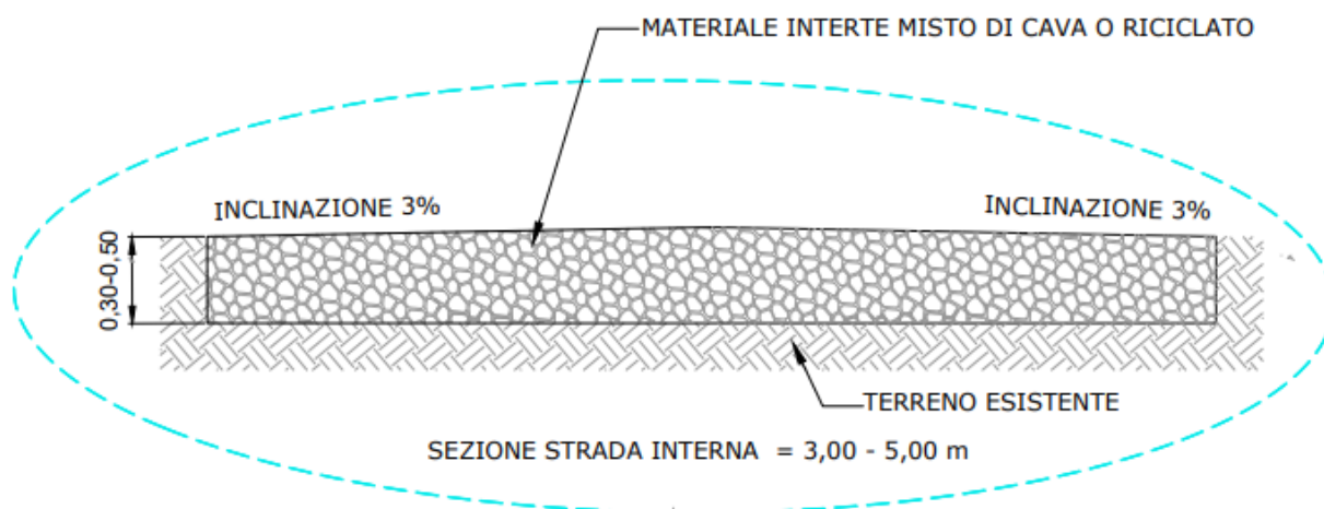
Fig. 14 – Viabilità interna
