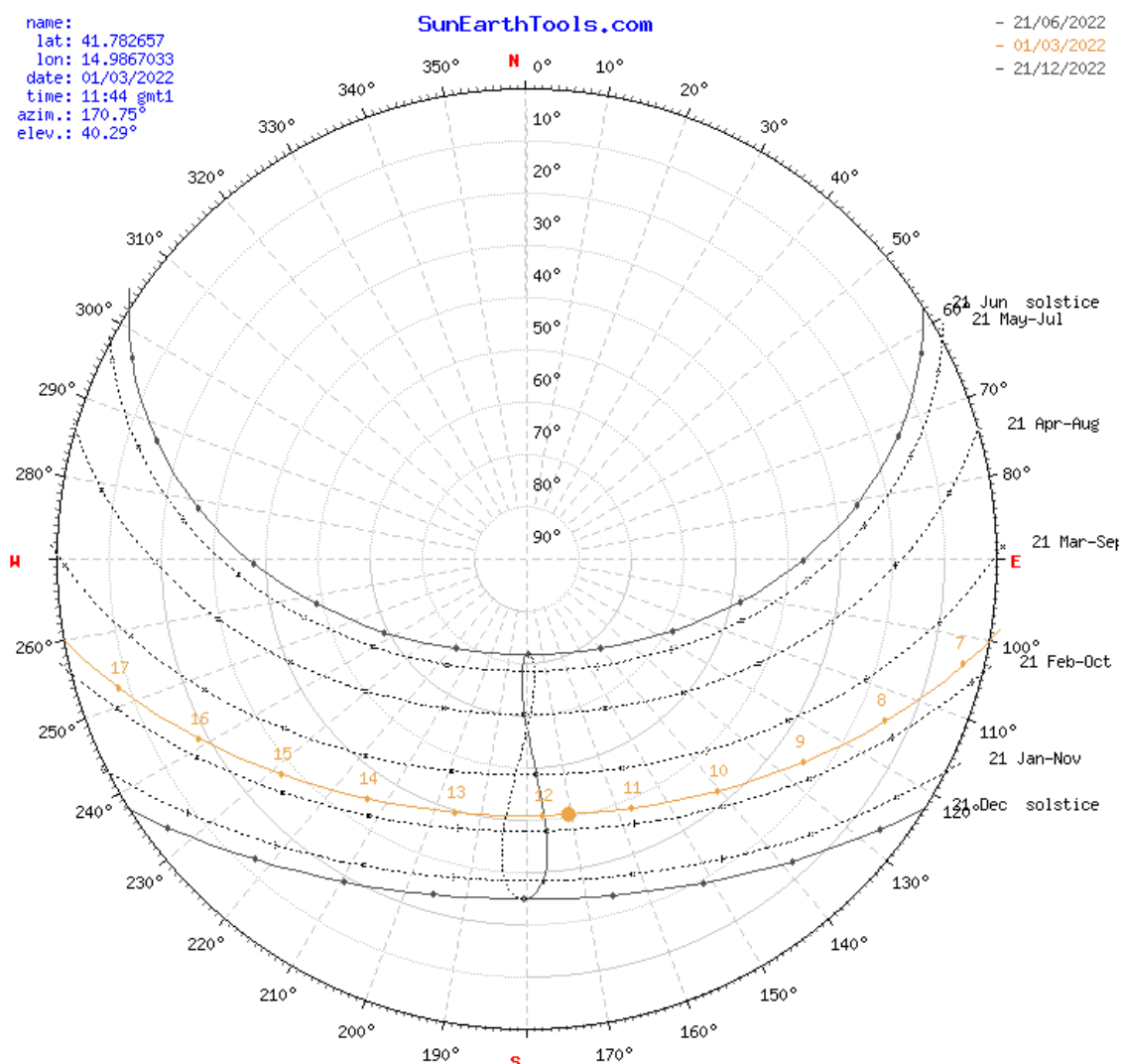
Fig. 22 - Diagramma Solare Polare (Montorio nei Frentani)
