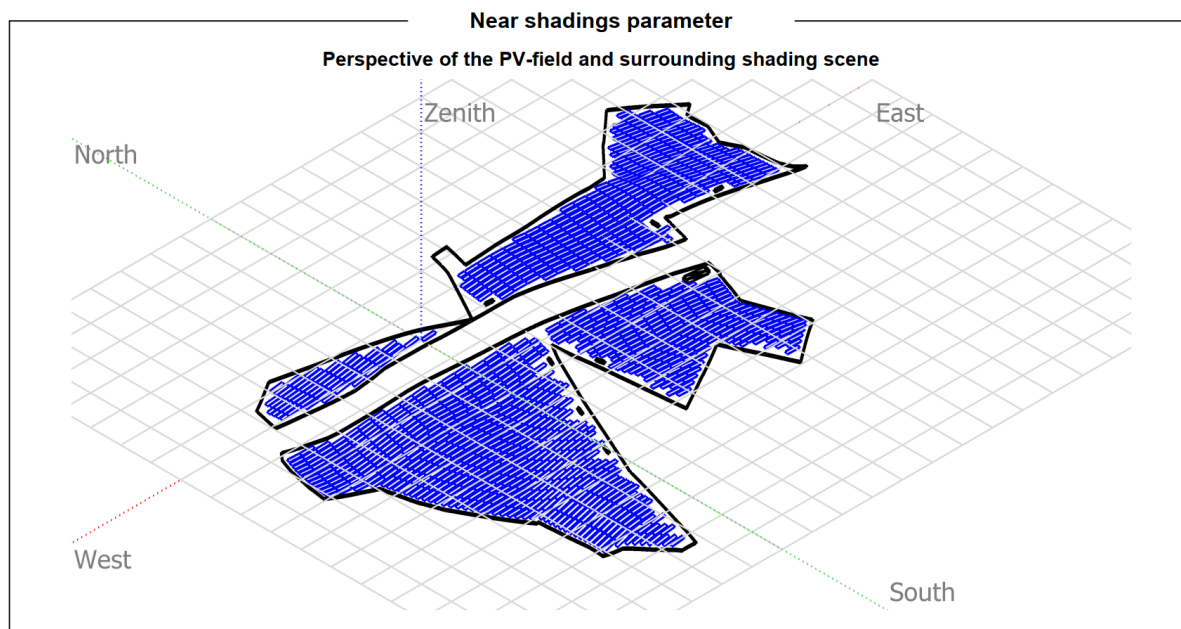
Fig. 24 – Modellizzazione 3D PVSyst (Montorio nei Frentani)
