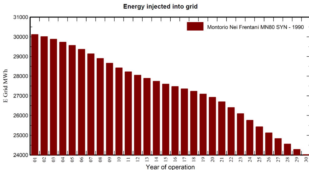
Fig. 26 – Producibilità dell’impianto con degrado moduli (30 anni)
