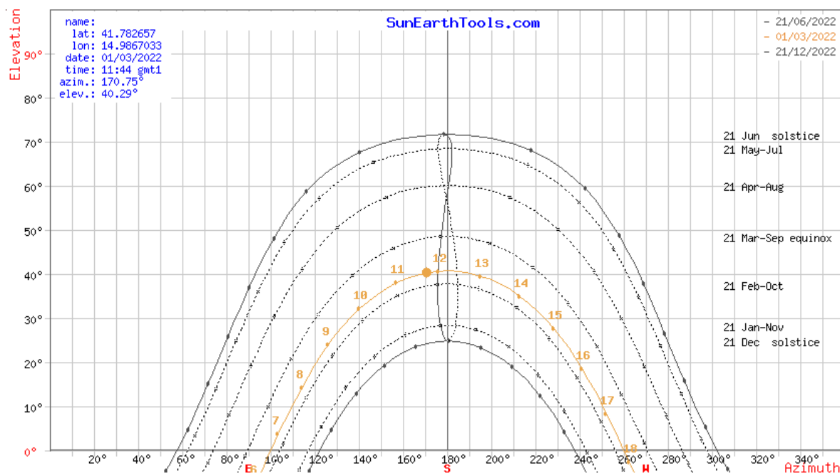
Fig. 23 - Diagramma Solare Polare (Montorio nei Frentani)
