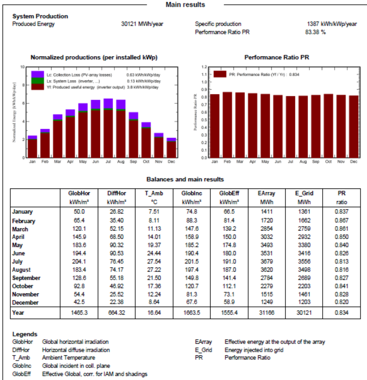
Fig. 25 - Risultati di calcolo (Fonte: PVsyst - Meteonorm)
