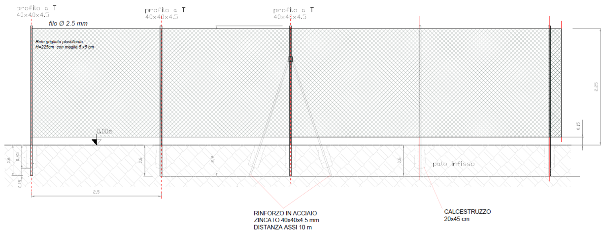
Fig. 12 – Recinzione perimetrale
