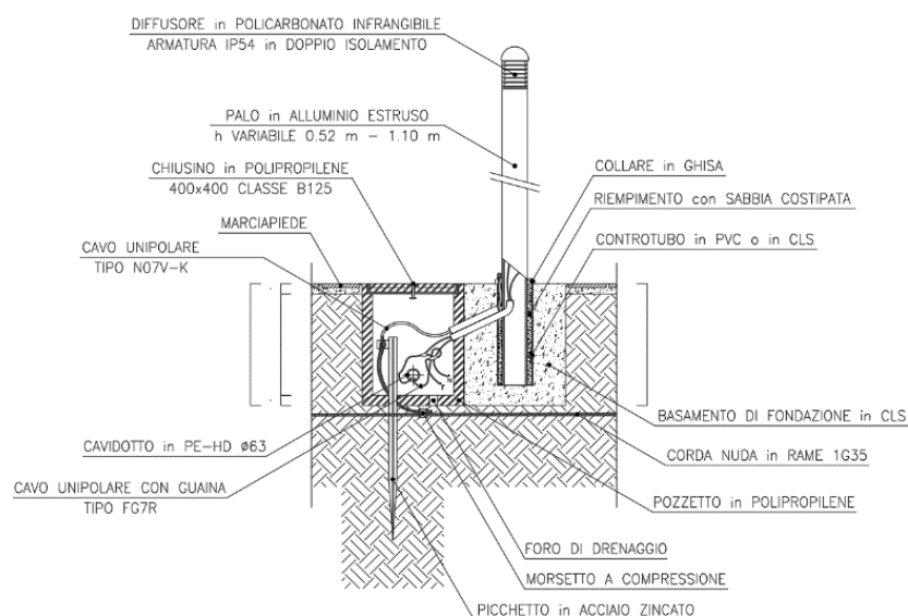
Fig. 3 - Tipologia di corpi illuminanti nei pressi delle cabine
