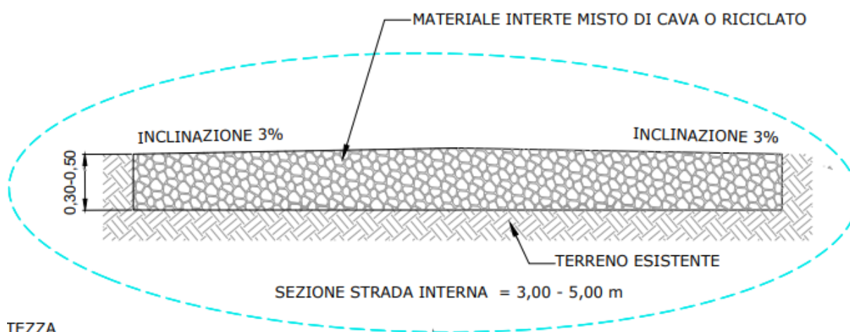
Fig. 20 – Sezione strada perimetrale
