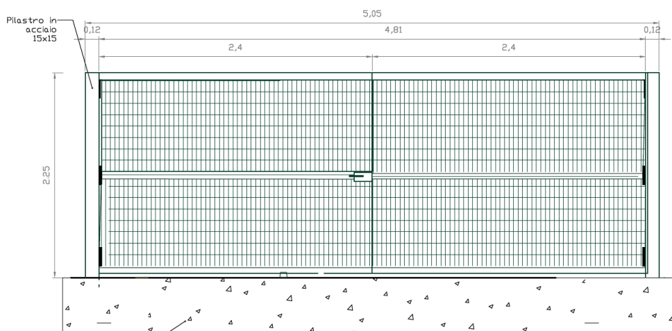
Fig. 19 – Cannello carrabile
