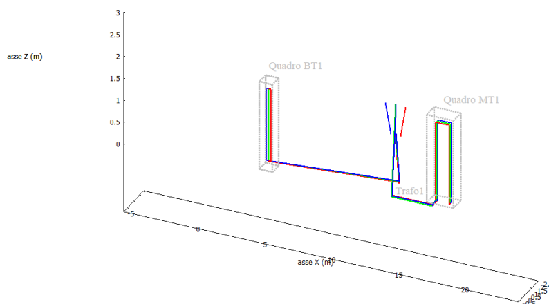
Fig.6 - Modello spaziale cablaggi nelle cabine di trasformazione MT/BT
