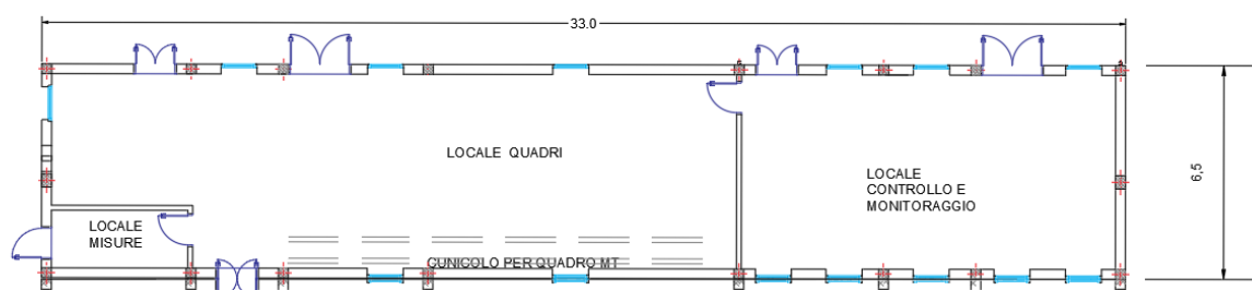
Fig.5 - Ingombri cabine di ricezione
