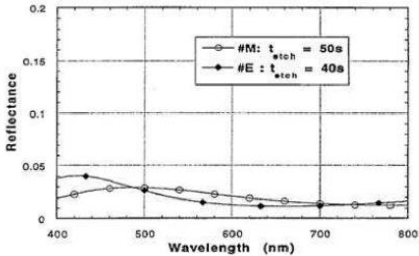
Figura 2 - Riflettanza di un modulo FV in funzione della lunghezza d'onda
