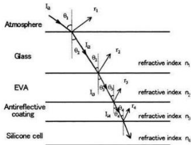
Figura 4 – Indici di rifrazione della luce solare all'interno dei vari strati componenti un modulo FV
