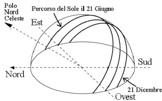
Figura 3: Movimento apparente del disco solare per un osservatore situato ad una latitudine nord attorno ai 45°. Per tutte le località situate tra il Tropico del Cancro e il Polo Nord Geografico il disco solare non raggiunge mai lo zenit.
