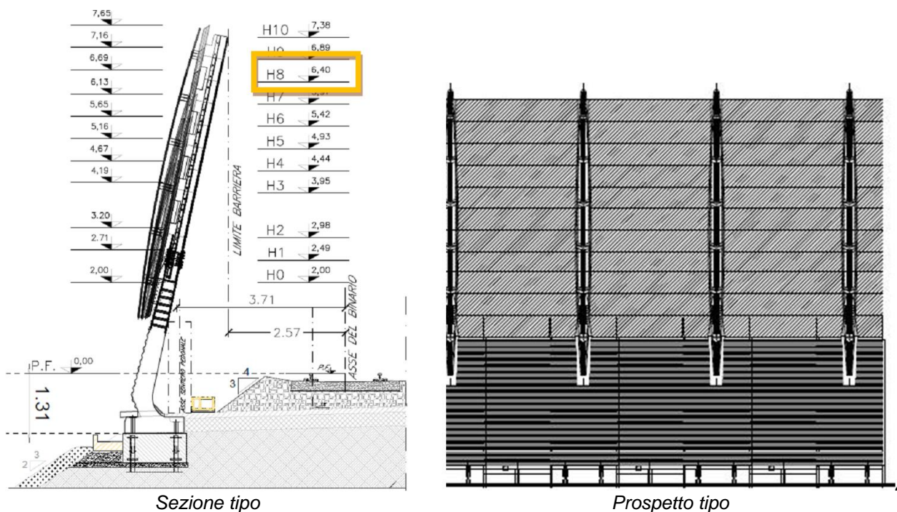
Figura 6 Sezione e prospetto tipo del modulo di barriera antirumore previsto nel caso specifico in studio (evidenziato in rettangolo colore giallo)
