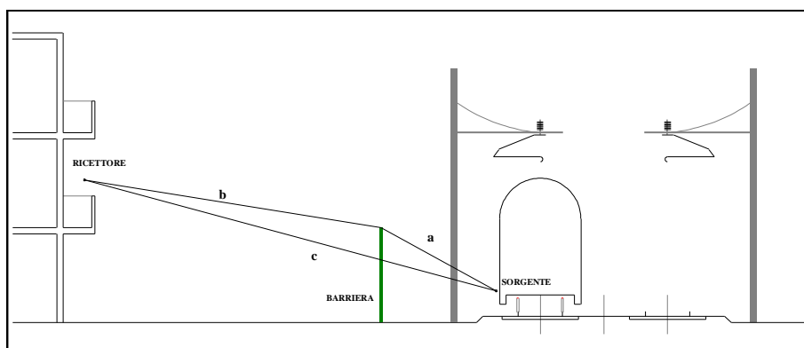
Figura 5 Propagazione dell'onda sonora con e senza barriera
