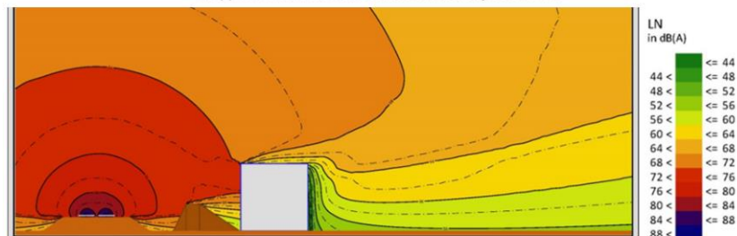
Mappa Verticale con Duna non interferente con edificio a 30m
