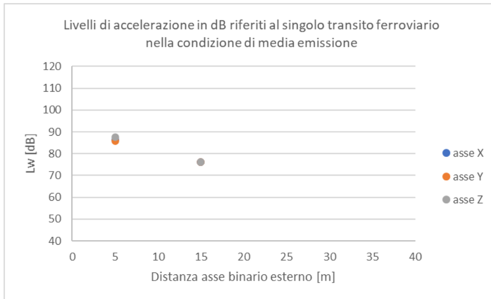
Figura 3-5 Livelli di accelerazione Lw,eq in dB riferiti ad un singolo transito di un convoglio nella condizione di media emissione rilevati in corrispondenza dei punti T1 e T2 a 5 e 15 m
