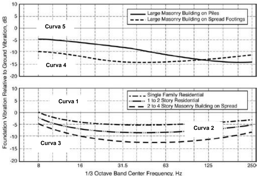
Figura 4-5 Fattori correttivi dovuti alla tipologia di fondazione
