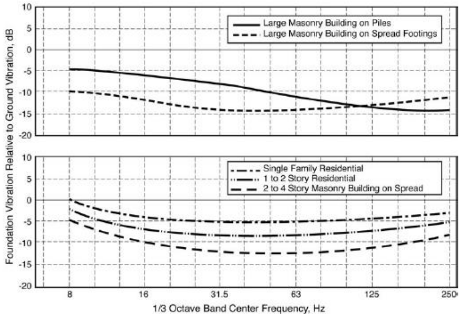
Figura 4-2 Risposta delle fondazioni per diverse tipologie di edifici (Fonte: FTA, USA)
