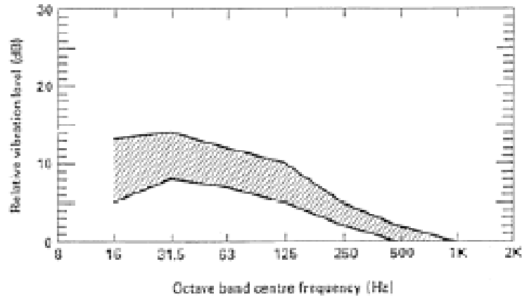
Figura 4-4 Amplificazione prodotta dai solai
