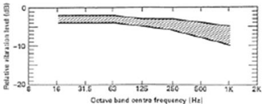
Figura 4-3 Attenuazione delle vibrazioni nel passaggio da un piano al successivo
