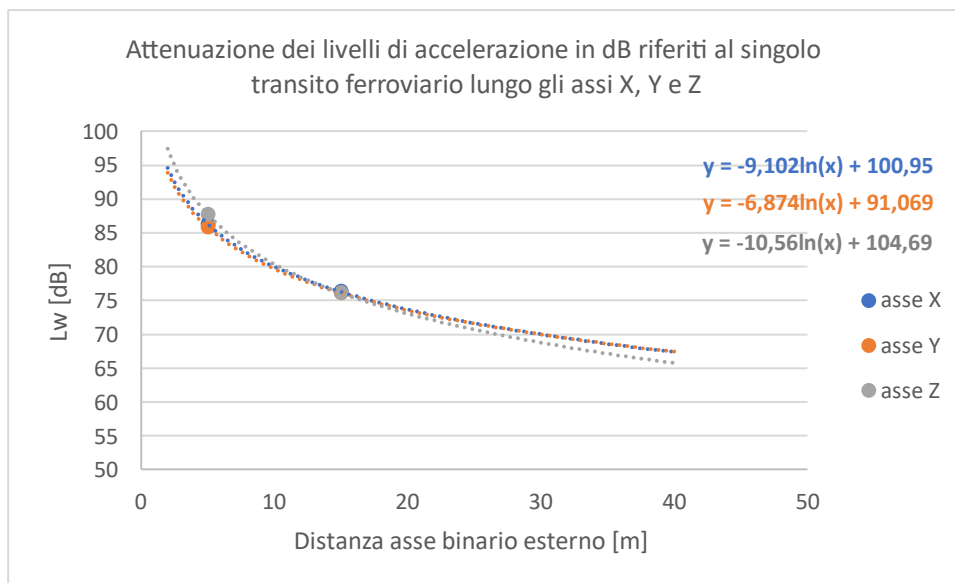
Figura 4-1 Attenuazione nel terreno delle vibrazioni indotte dal transito di un treno ferroviario
