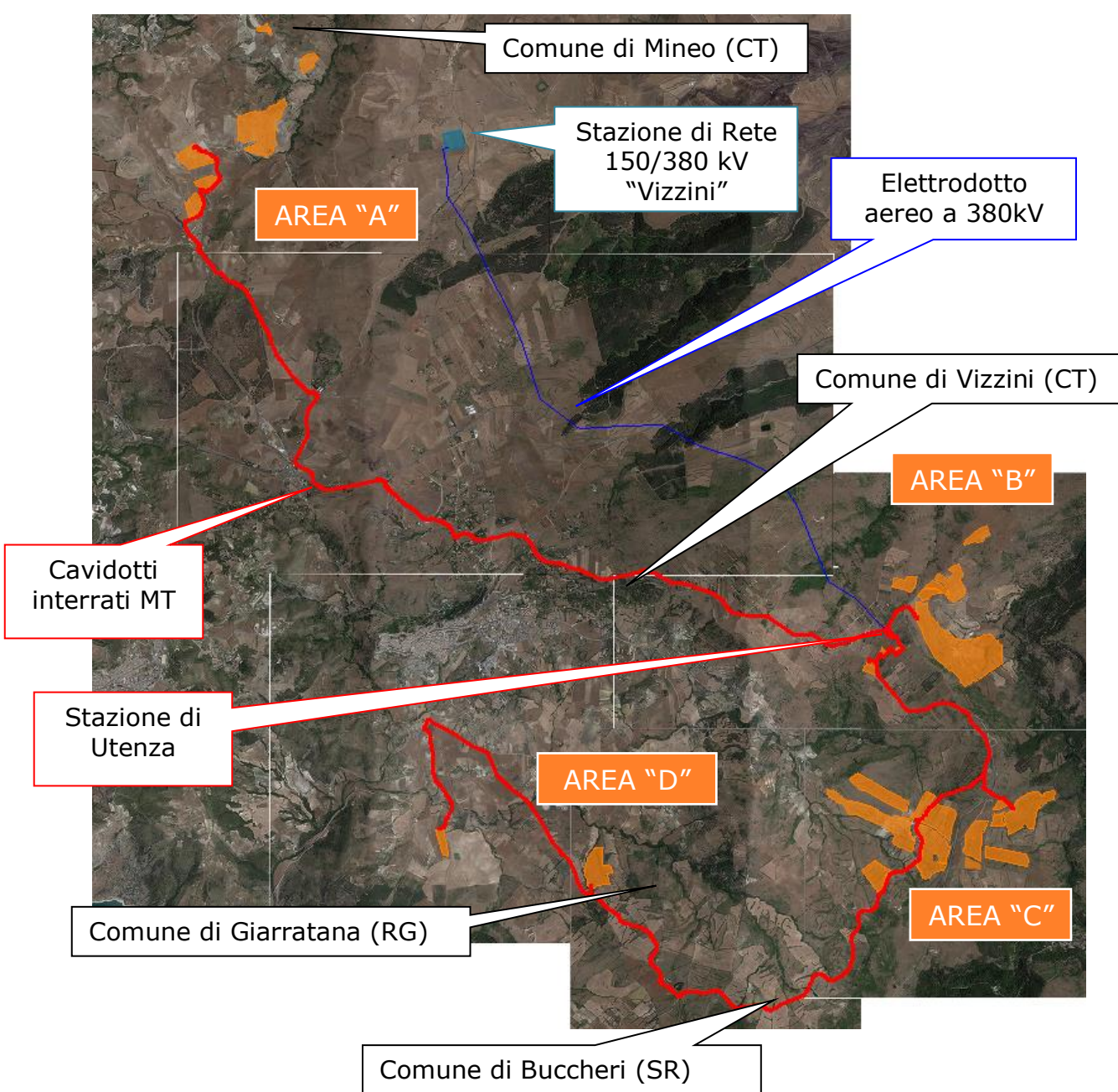
Figura 1 – Planimetria su ortofoto dell’impianto fotovoltaico e delle opere di connessione
