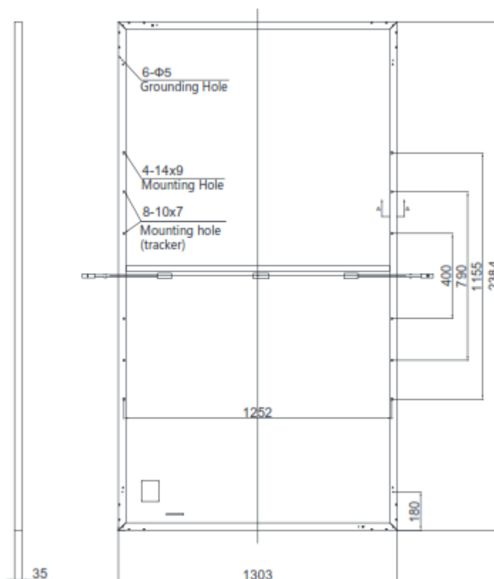
Figura 2 – Dimensioni del modulo fotovoltaico
