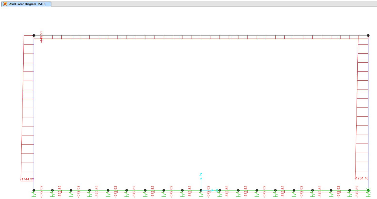
Figura 14: Sforzo assiale in combinazione SLU
