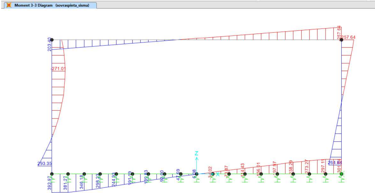
Figura 10: Momento flettente per la sovrappinta sismica
