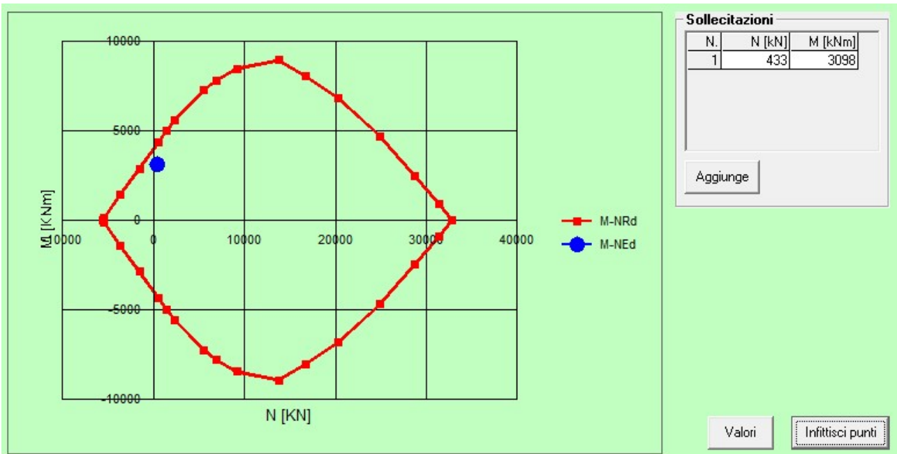
Figura 25: Combinazione SLU
