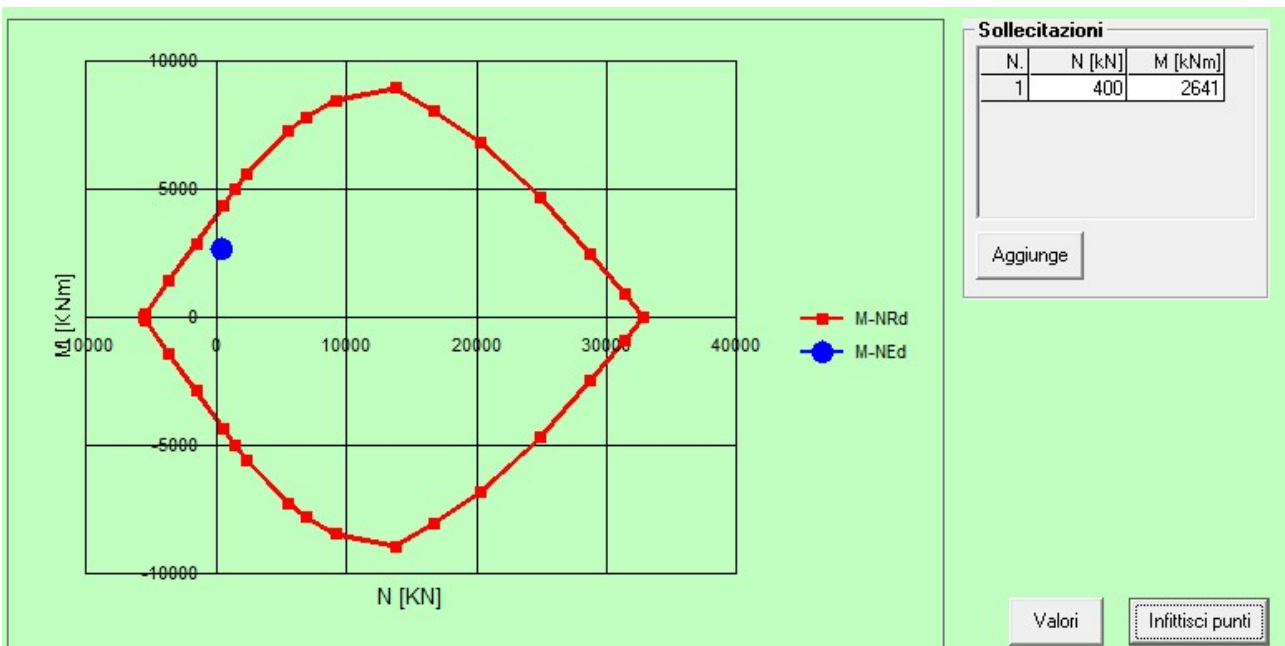
Figura 26: Combinazione SLV
