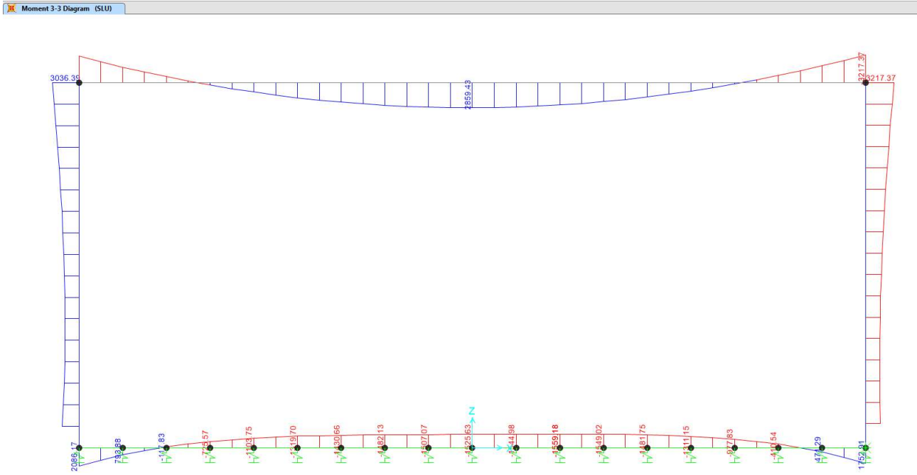
Figura 13: Momento flettente in combinazione SLU
