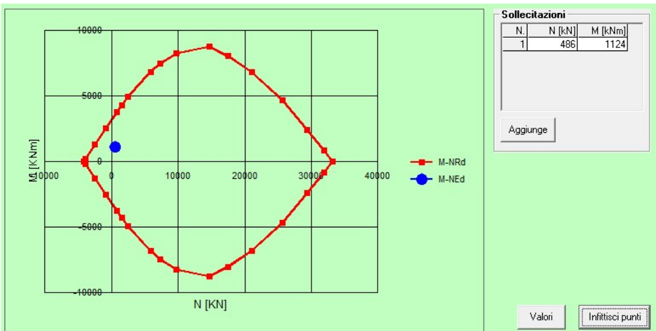
Figura 28: Combinazione SLV
