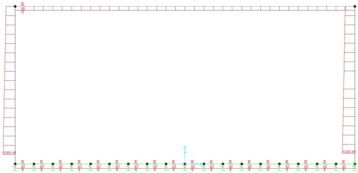
Figura 17: Sforzo assiale in combinazione SLV
