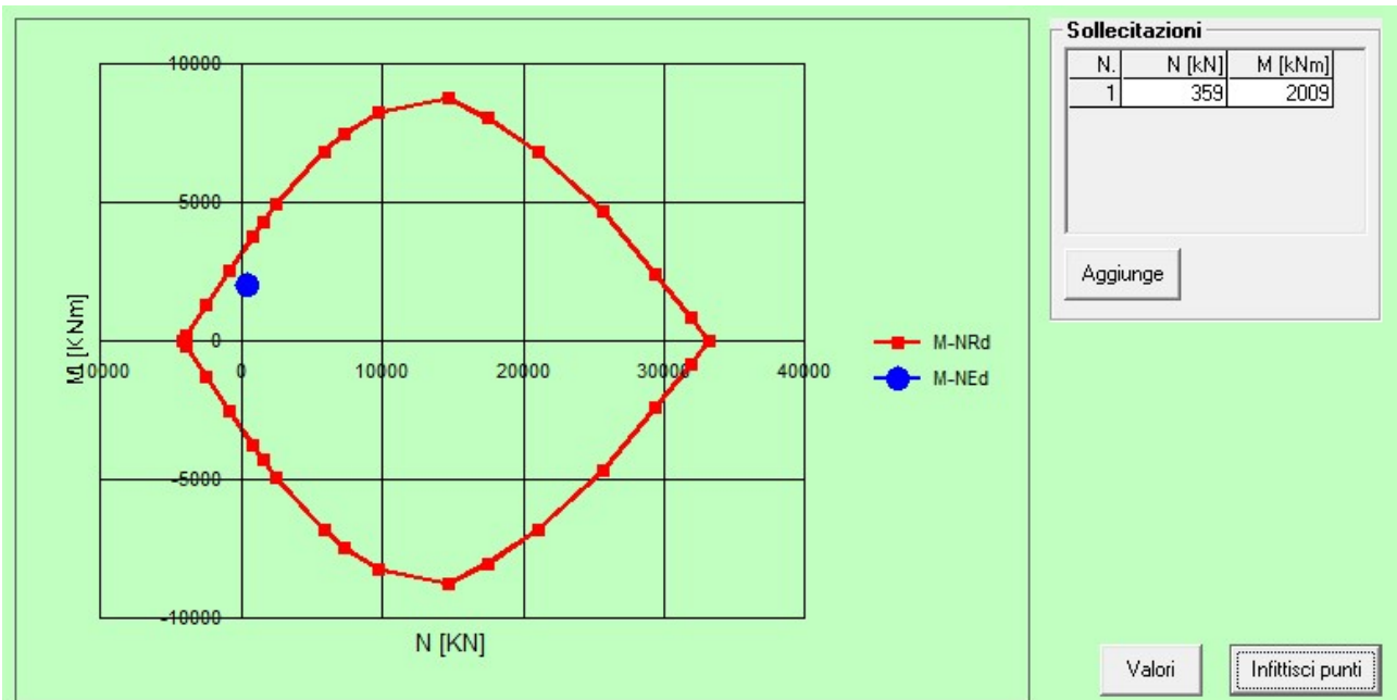
Figura 29: Combinazione SLU
