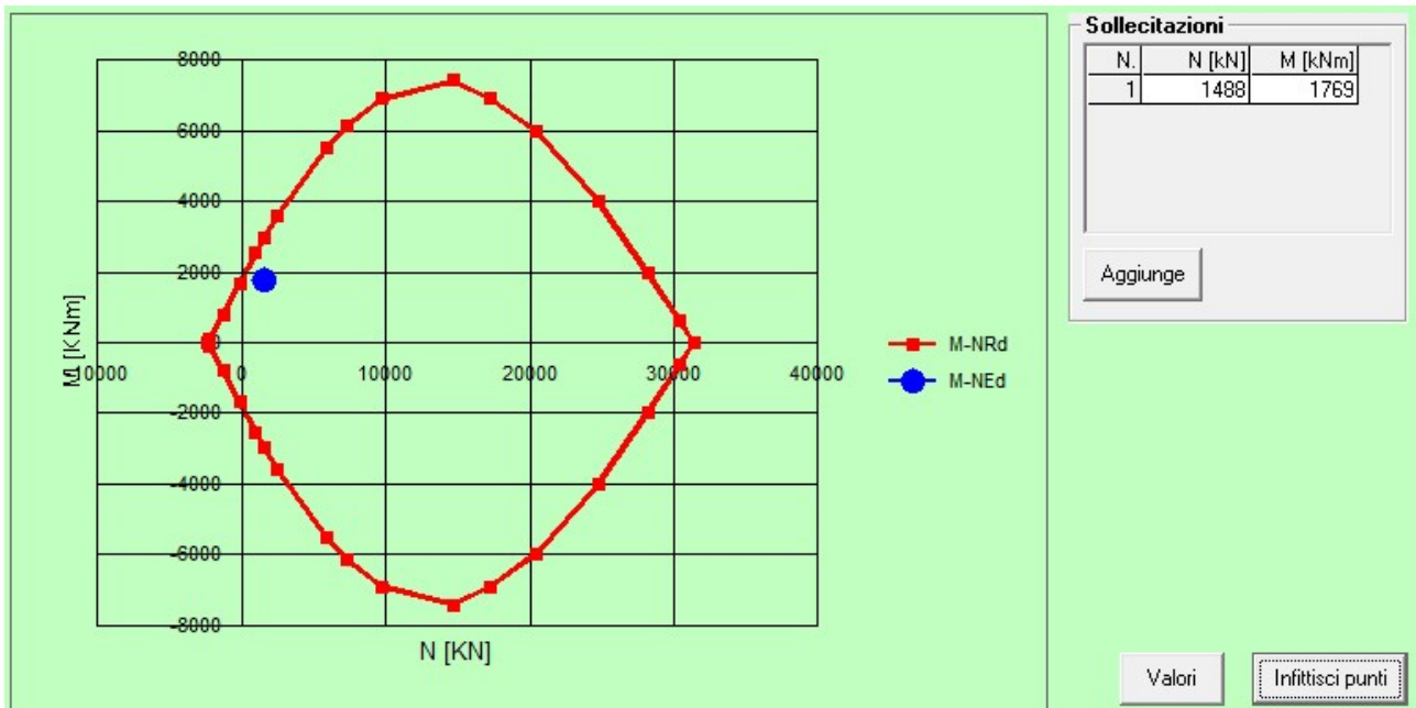
Figura 21: Combinazione SLU
