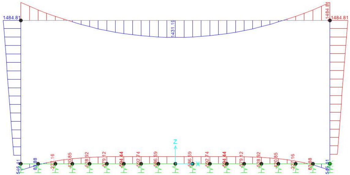
Moment 3-3 Diagram (q_terreno_superiore)
