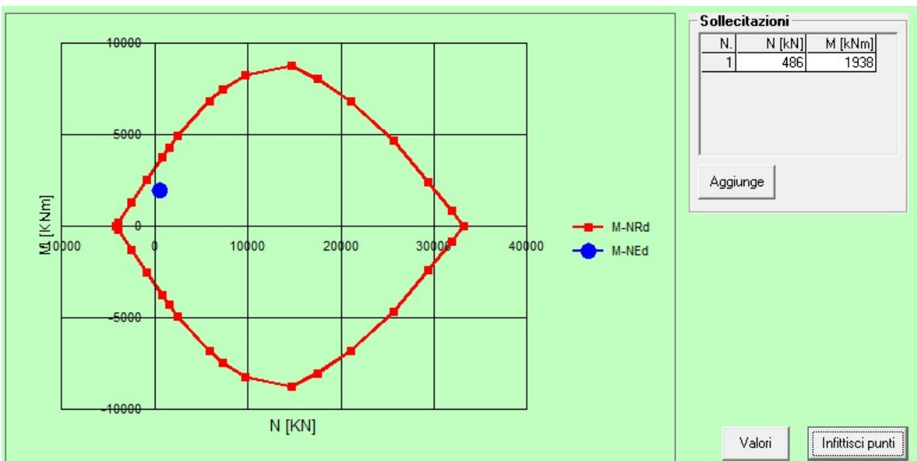
Figura 30: Combinazione SLV
