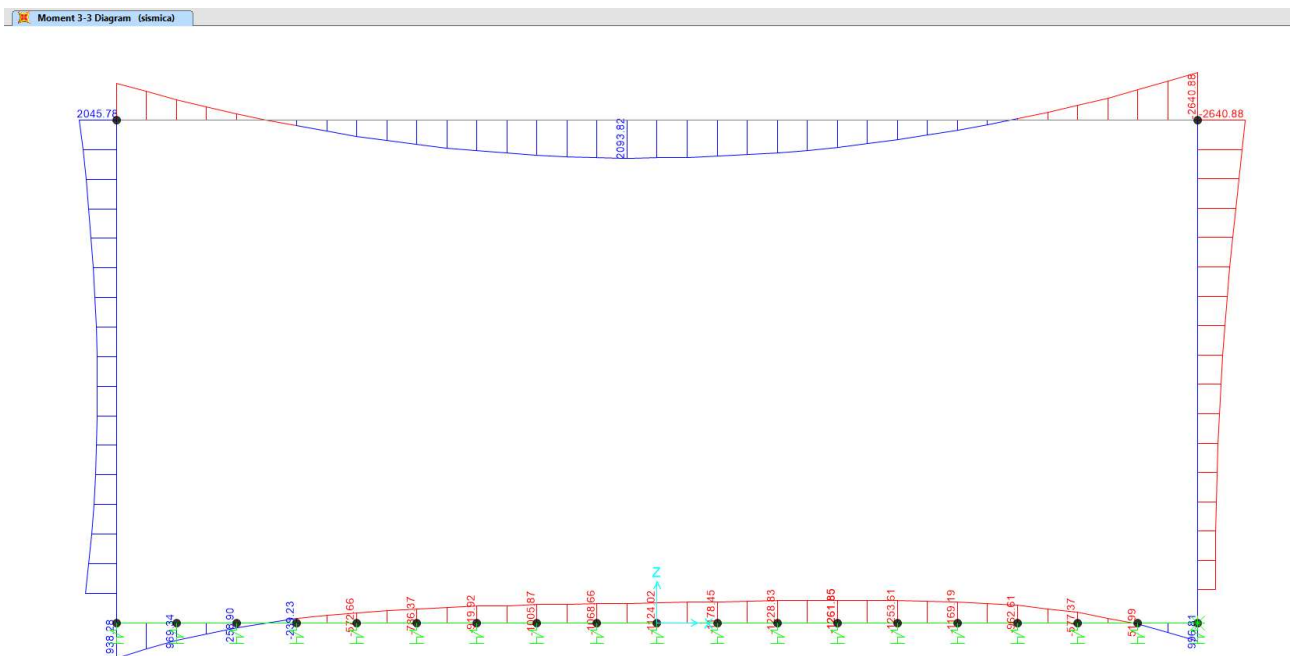
Figura 16: Momento flettente in combinazione SLV
