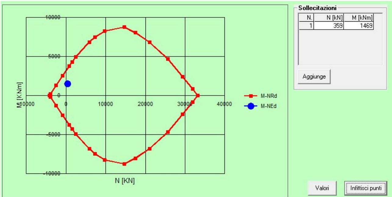
Figura 27: Combinazione SLU
