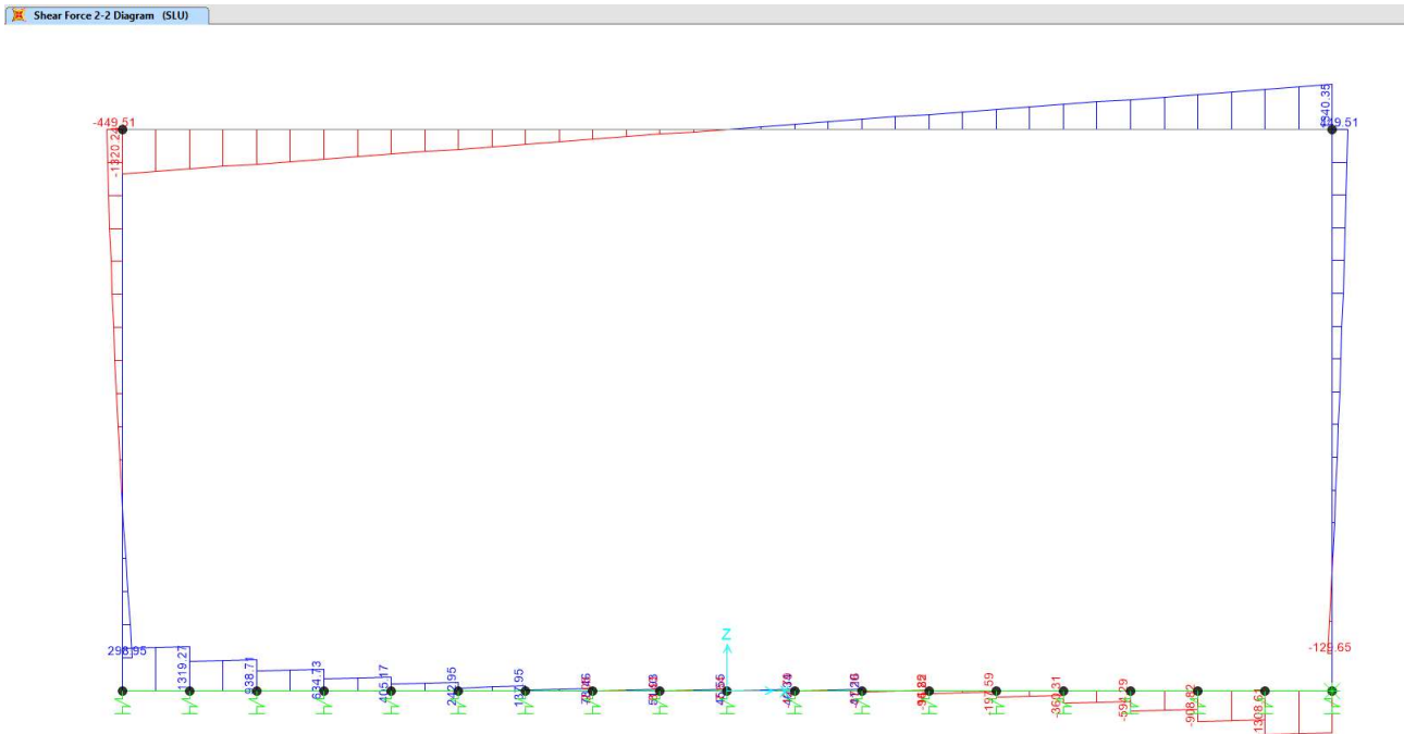
Figura 15: Taglio in combinazione SLU
