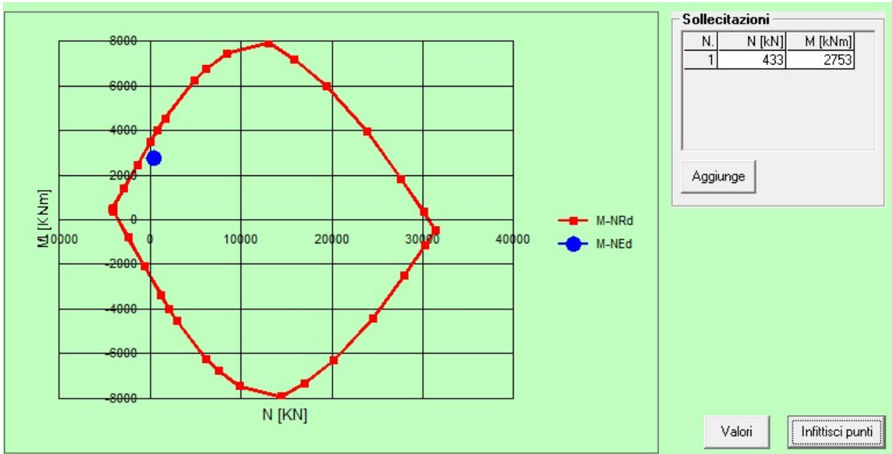
Figura 23: Combinazione SLU
