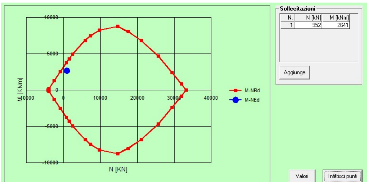
Figura 20: Combinazione SLV
