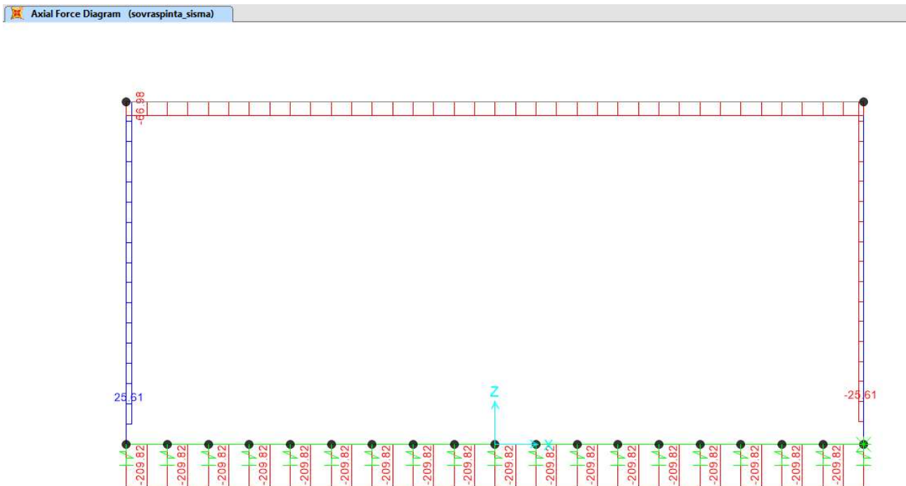
Figura 11: Sforzo assiale per la sovrappinta sismica
