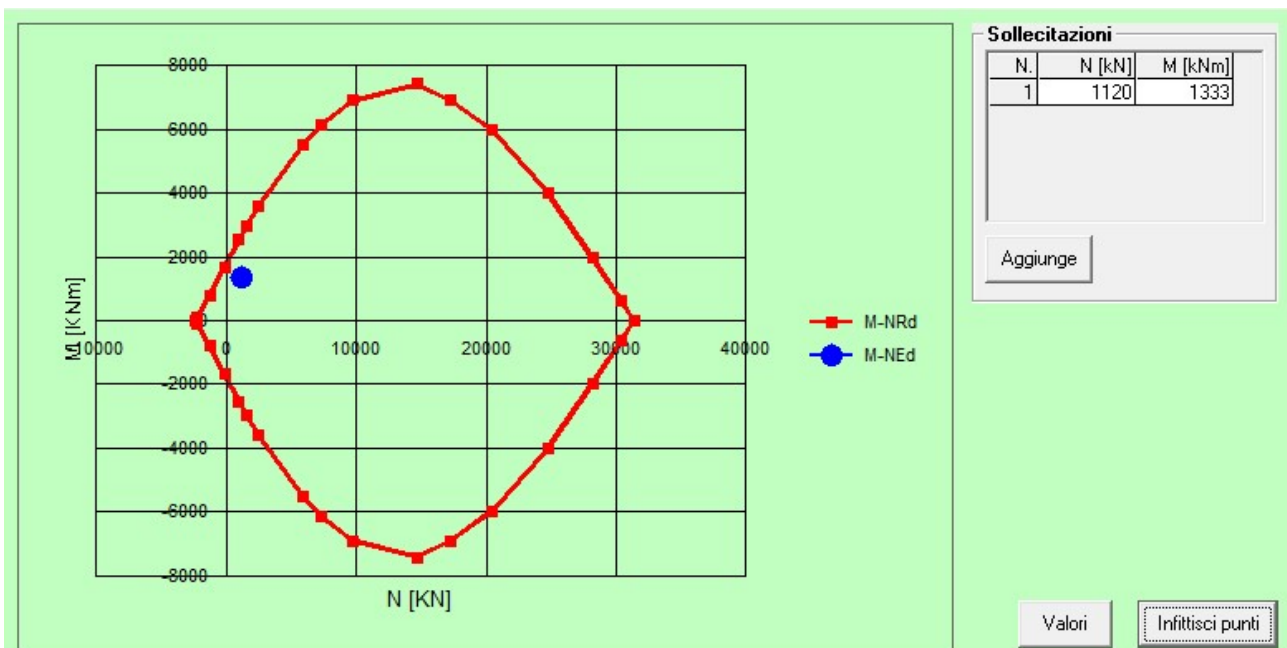
Figura 22: Combinazione SLV
