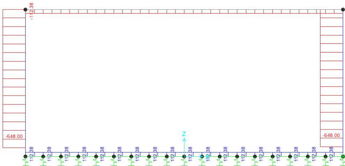
Figura 7: sforzo assiale dovuto alla presenza del terreno superiore
