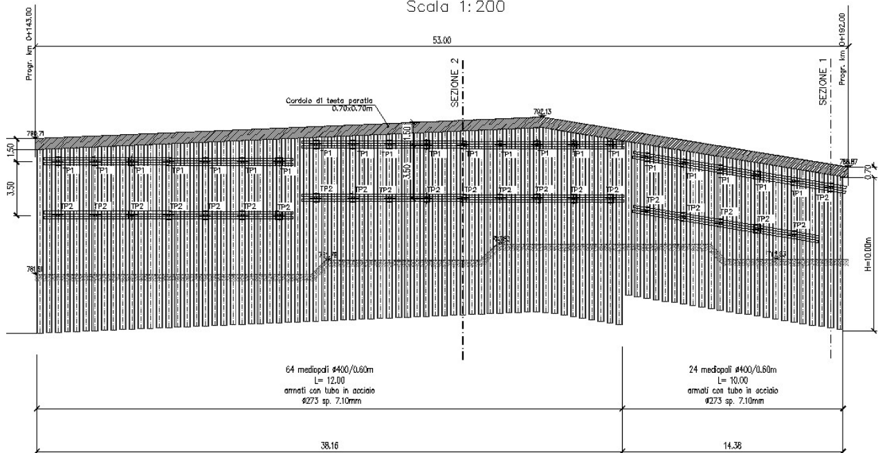
Figura 3: sviluppata paratia provvisoria
