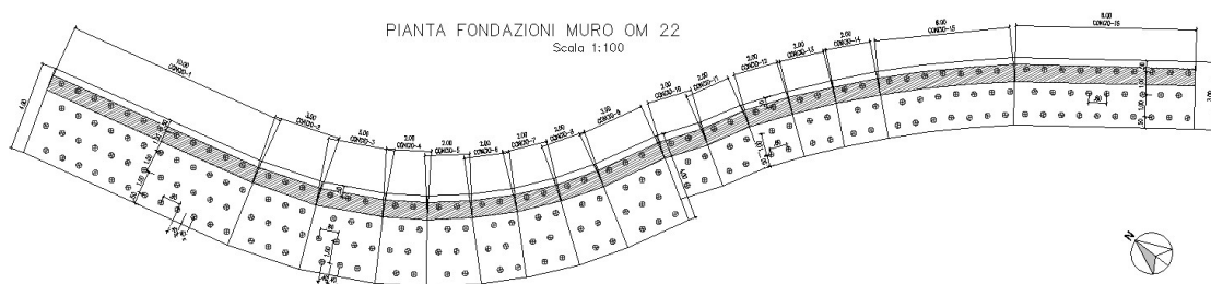
Figura 3: pianta del muro
