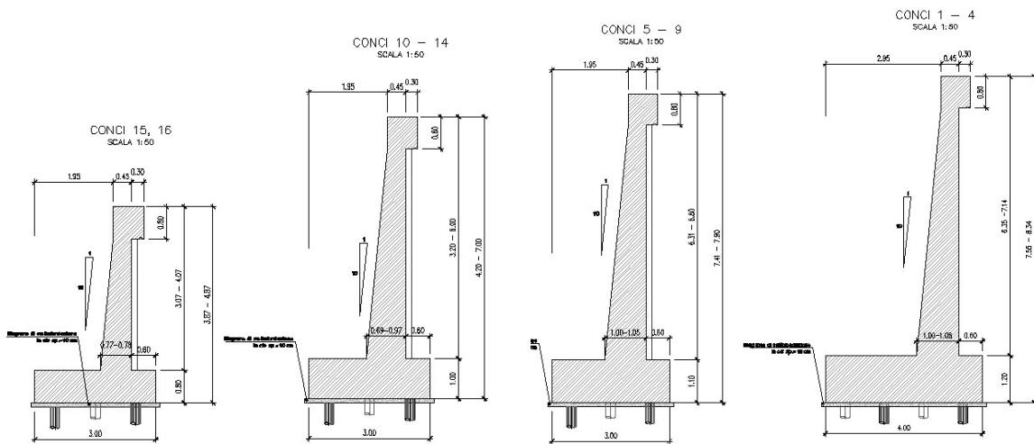
Figura 2: carpenteria del muro
