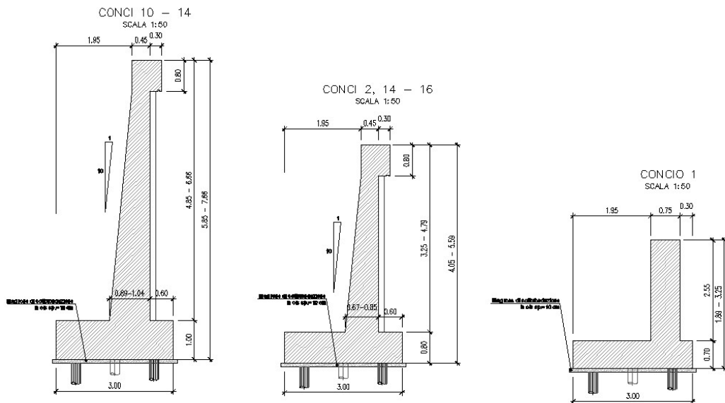
Figura 2: carpenteria del muro
