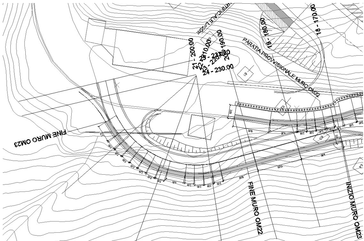
Figura 4: planimetria del muro
