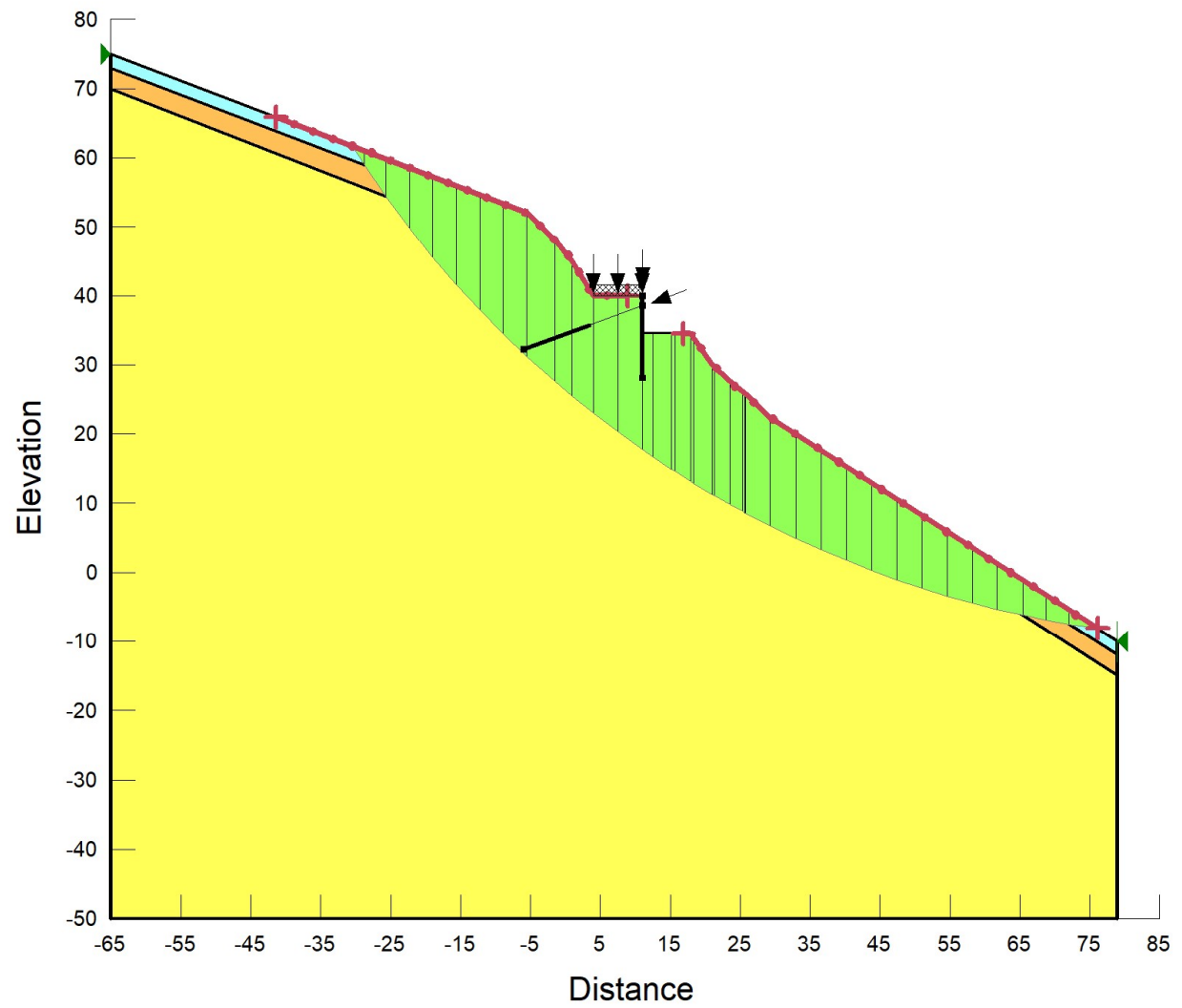
Figura 8 Coefficiente di sicurezza minimo per la stabilità globale in condizioni sismiche (EQK+M2) (+)
