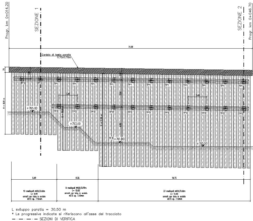
Figura 3: sviluppata paratia provvisoria
