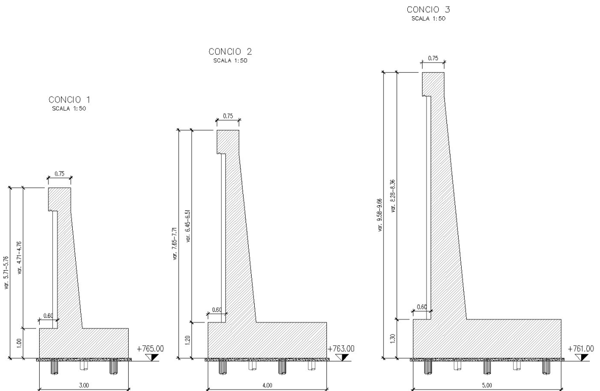
Figura 2: carpenteria del muro
