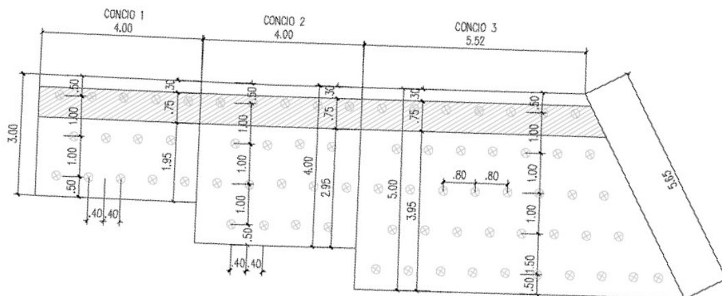
Figura 3: pianta del muro
