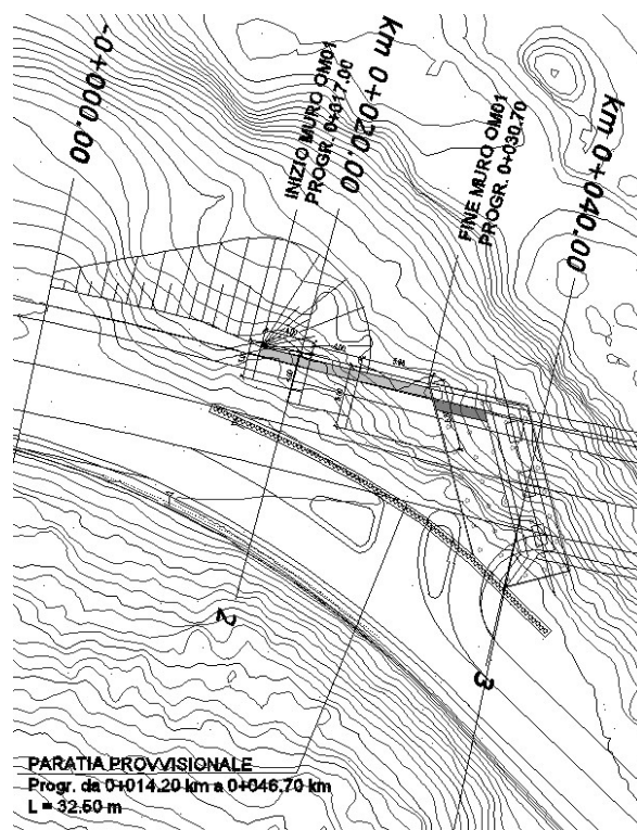
Figura 4 Planimetria d'intervento
