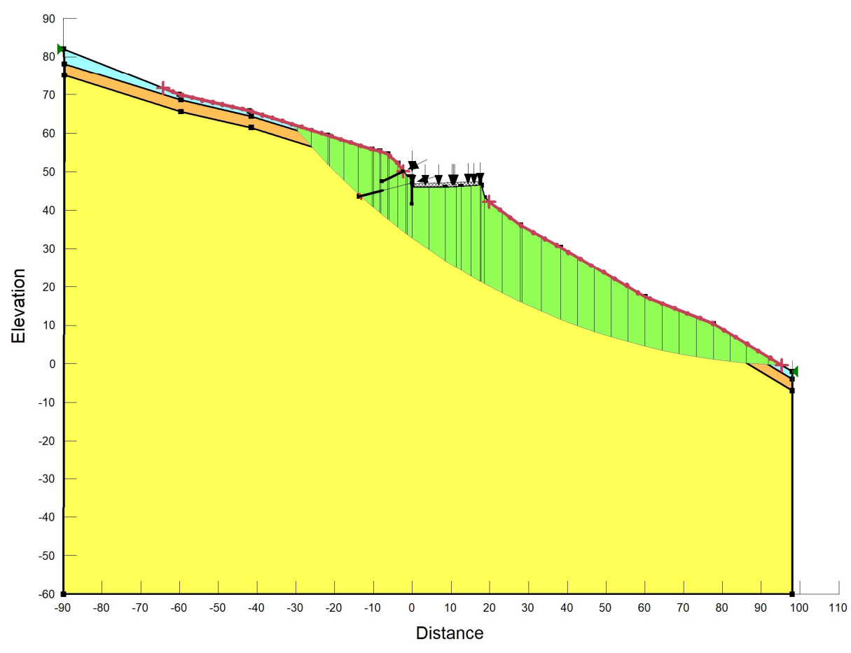
Figura 9 Coefficiente di sicurezza minimo per la stabilità globale in condizioni sismiche (EQK+M2) (+)
