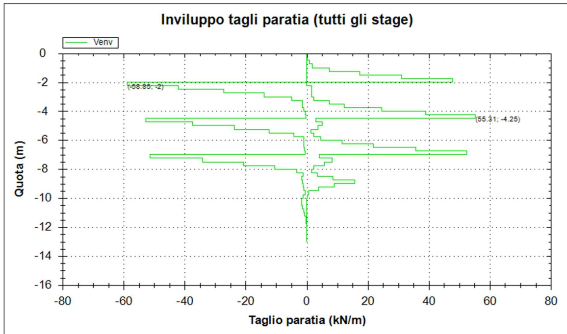
Figura 39: Diagramma del taglio (A1+M1+R1)
