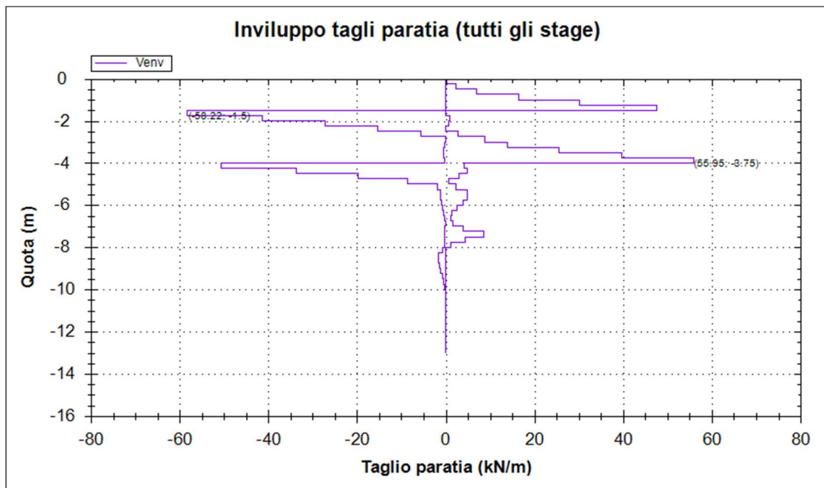
Figura 32: Diagramma del taglio (A1+M1+R1)
