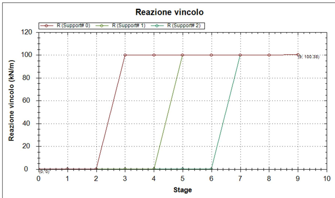
Figura 42: Reazioni tiranti (EQK+M1+R1)
