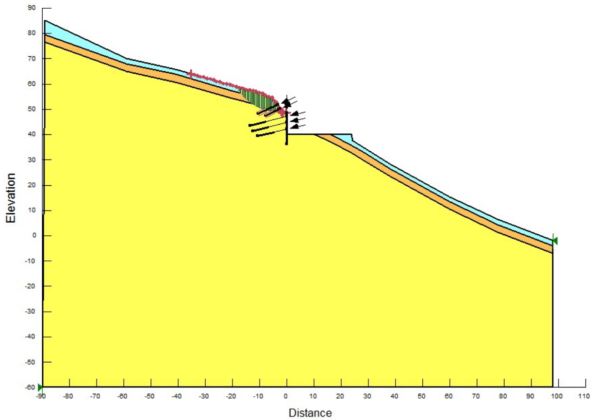
Figura 20: Coefficiente di sicurezza minimo per la stabilità globale in condizioni statiche (A2+M2)
