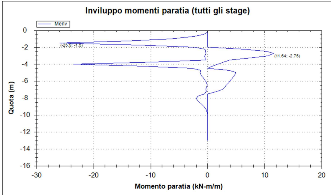
Figura 30: Diagramma dei momenti flettenti (A1+M1+R1)
