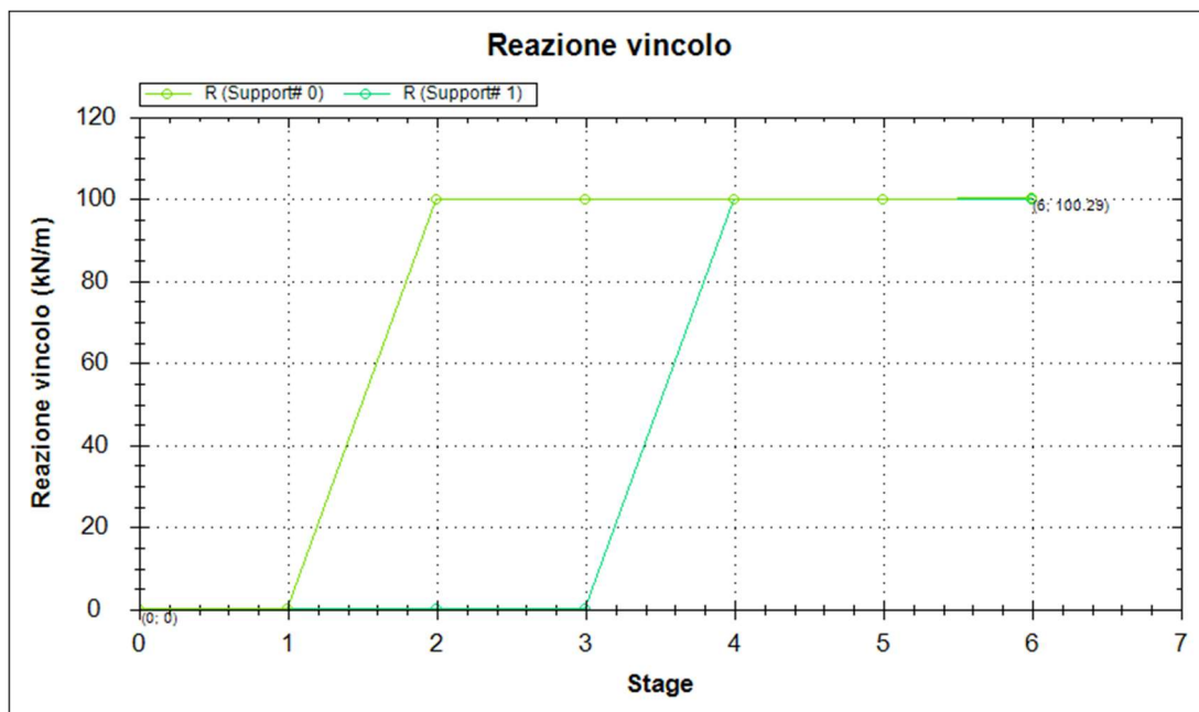
Figura 35: Reazioni tiranti (EQK+M1+R1)
