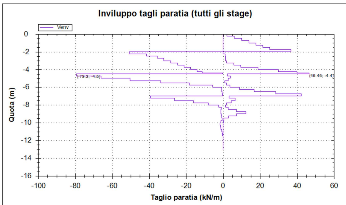
Figura 40: Diagramma del taglio (EQK+M1+R1)
