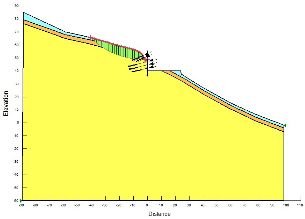
Figura 22: Coefficiente di sicurezza minimo per la stabilità globale in condizioni sismiche (EQK+M2) (-)
