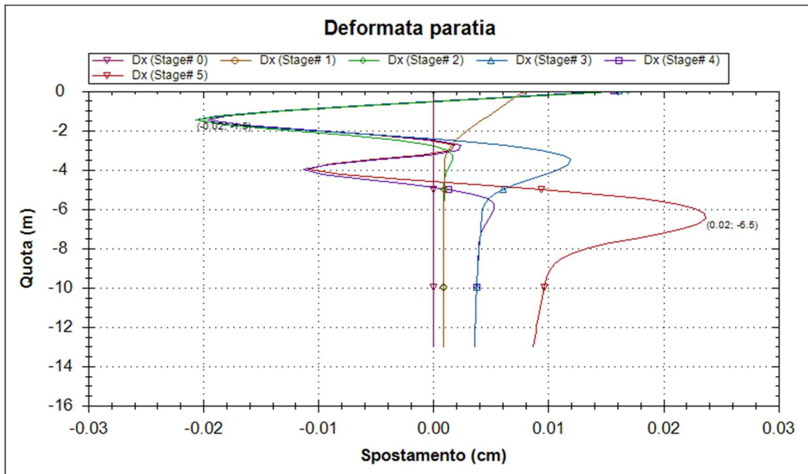
Figura 36: Diagramma degli spostamenti orizzontali (SLE)
