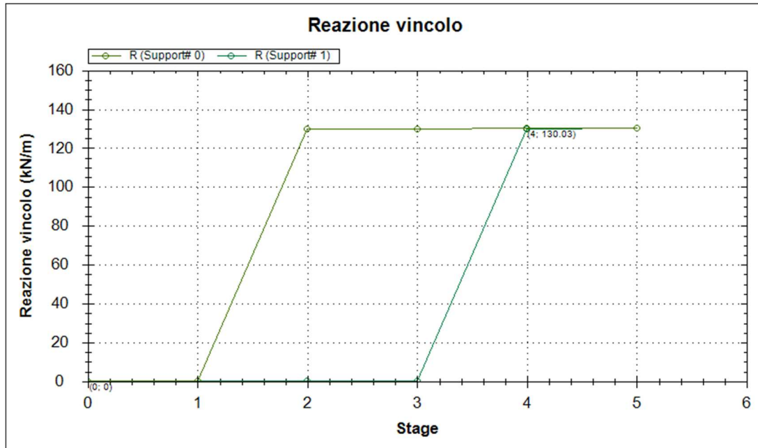
Figura 34: Reazioni tiranti (A1+M1+R1)
