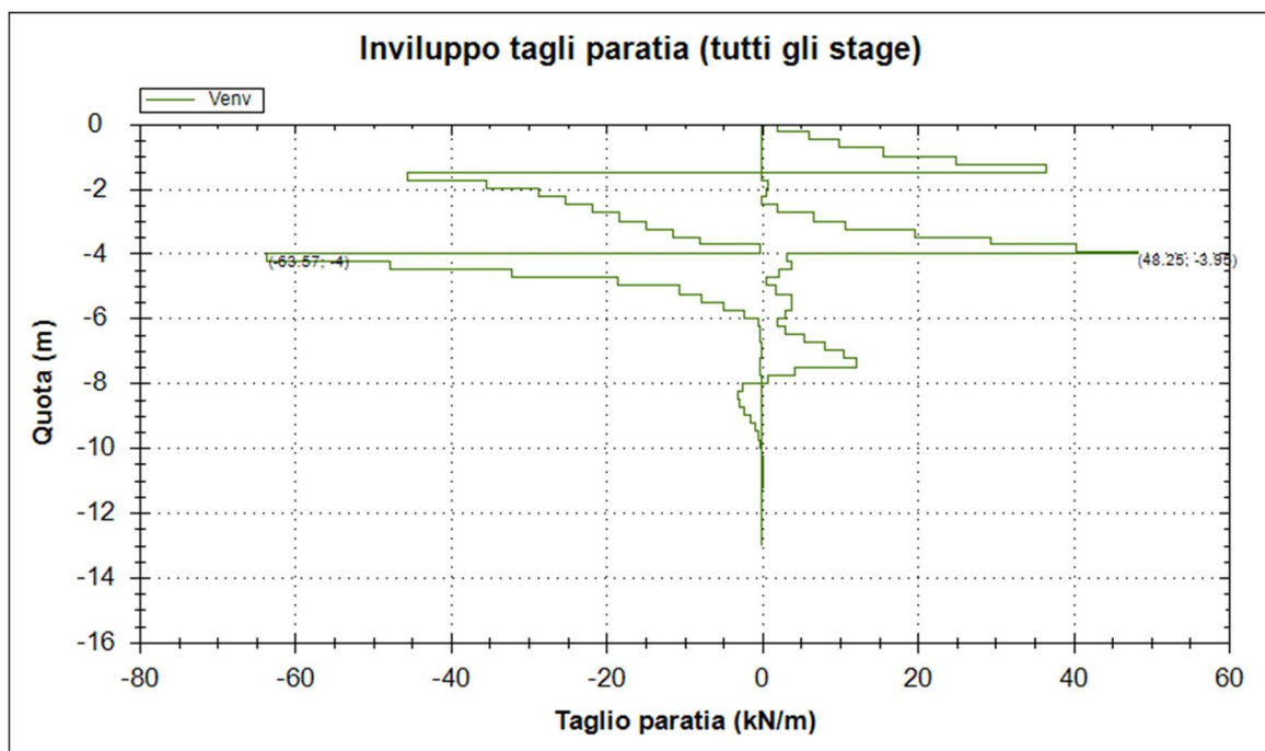
Figura 33: Diagramma del taglio (EQK+M1+R1)
