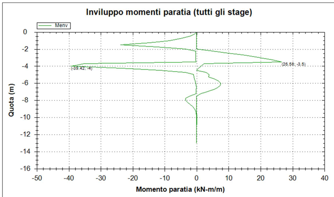
Figura 31: Diagramma dei momenti flettenti (EQK+M1+R1)
