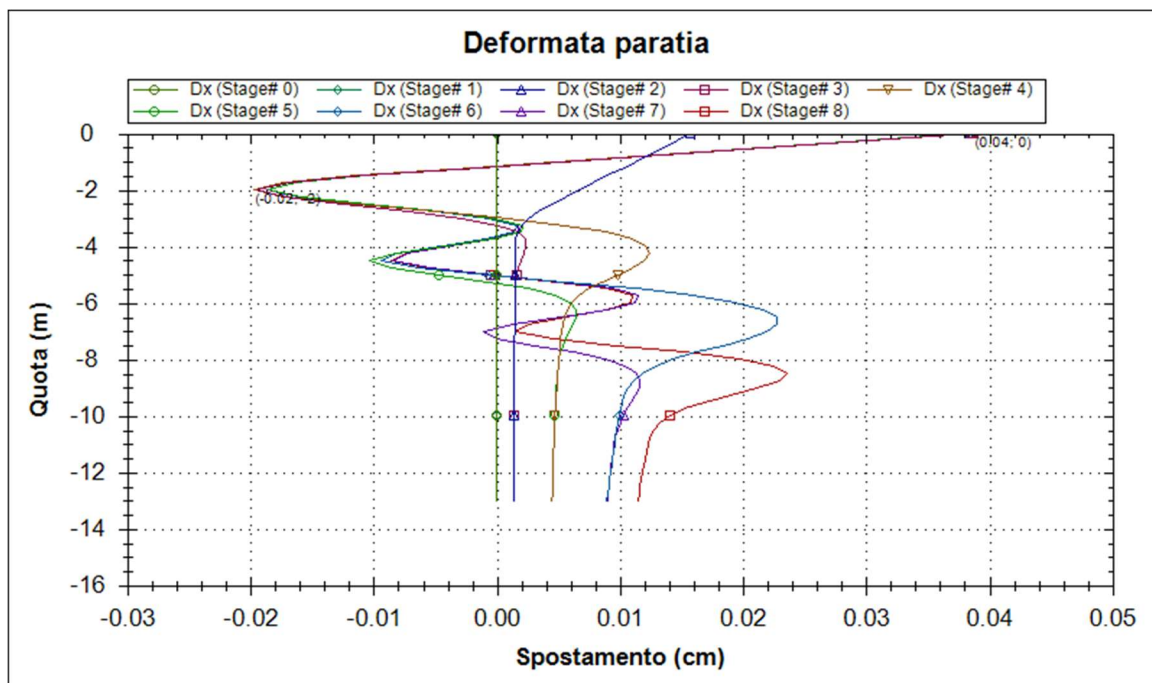
Figura 43: Diagramma degli spostamenti orizzontali (SLE)
