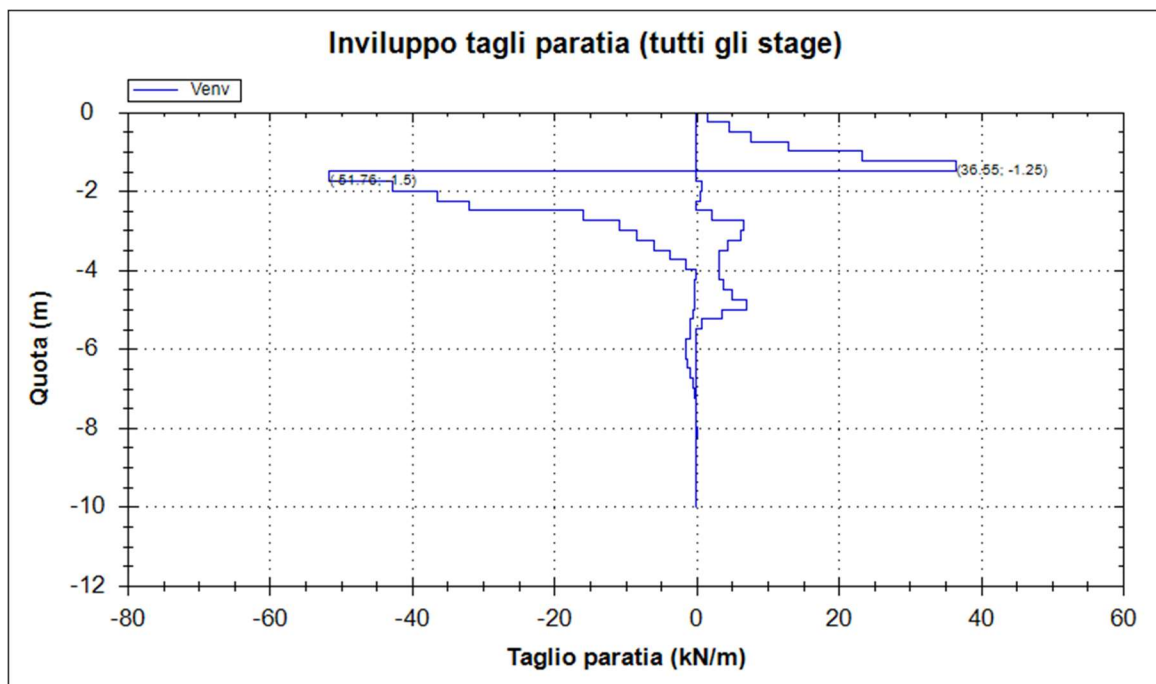
Figura 26: Diagramma del taglio (EQK+M1+R1)
