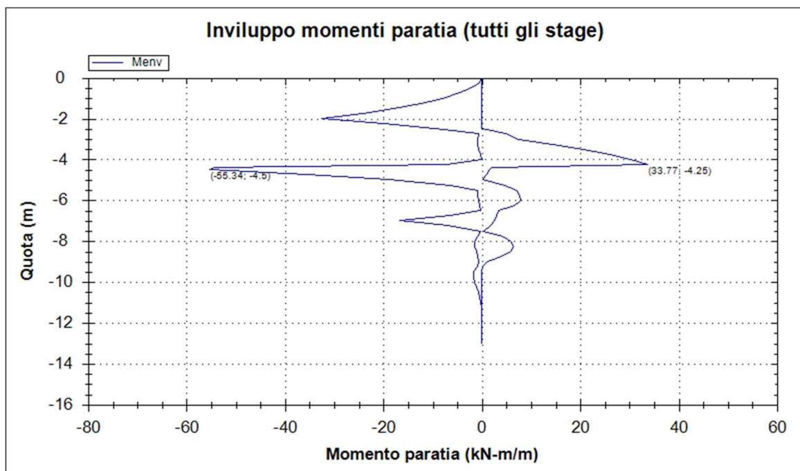
Figura 38: Diagramma dei momenti flettenti (EQK+M1+R1)
