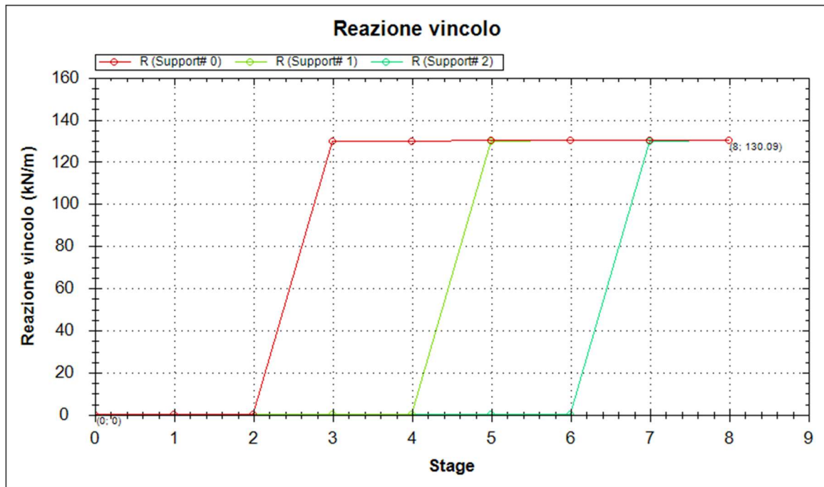
Figura 41: Reazioni tiranti (A1+M1+R1)
