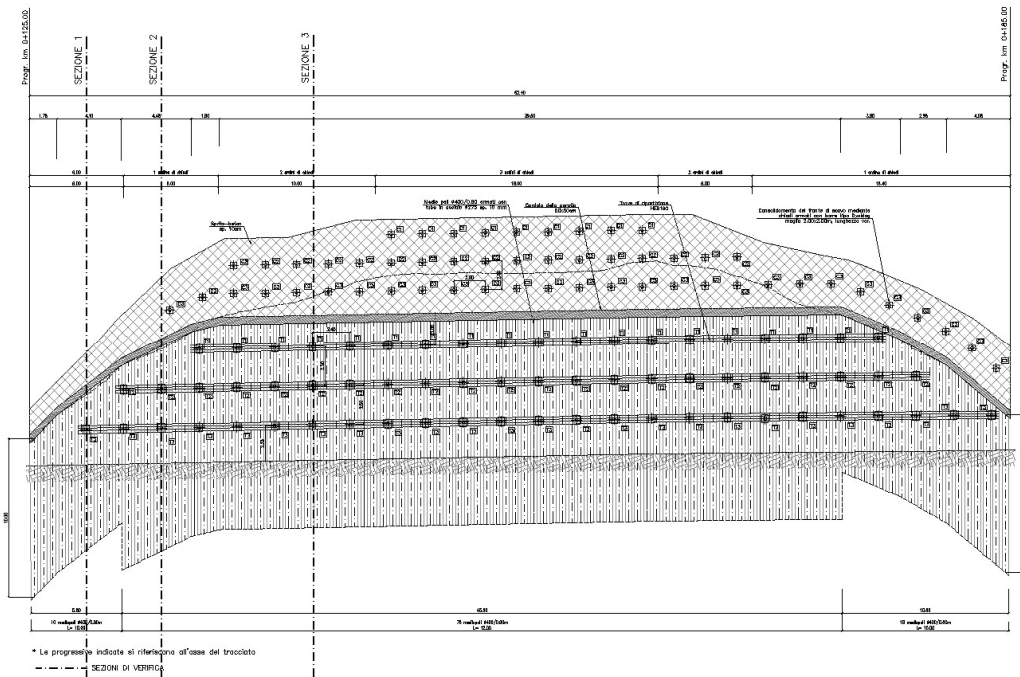
Figura 1 Sviluppata della paratia OM03
