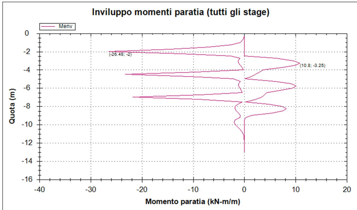
Figura 37: Diagramma dei momenti flettenti (A1+M1+R1)
