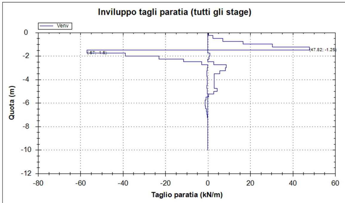
Figura 25: Diagramma del taglio (A1+M1+R1)
