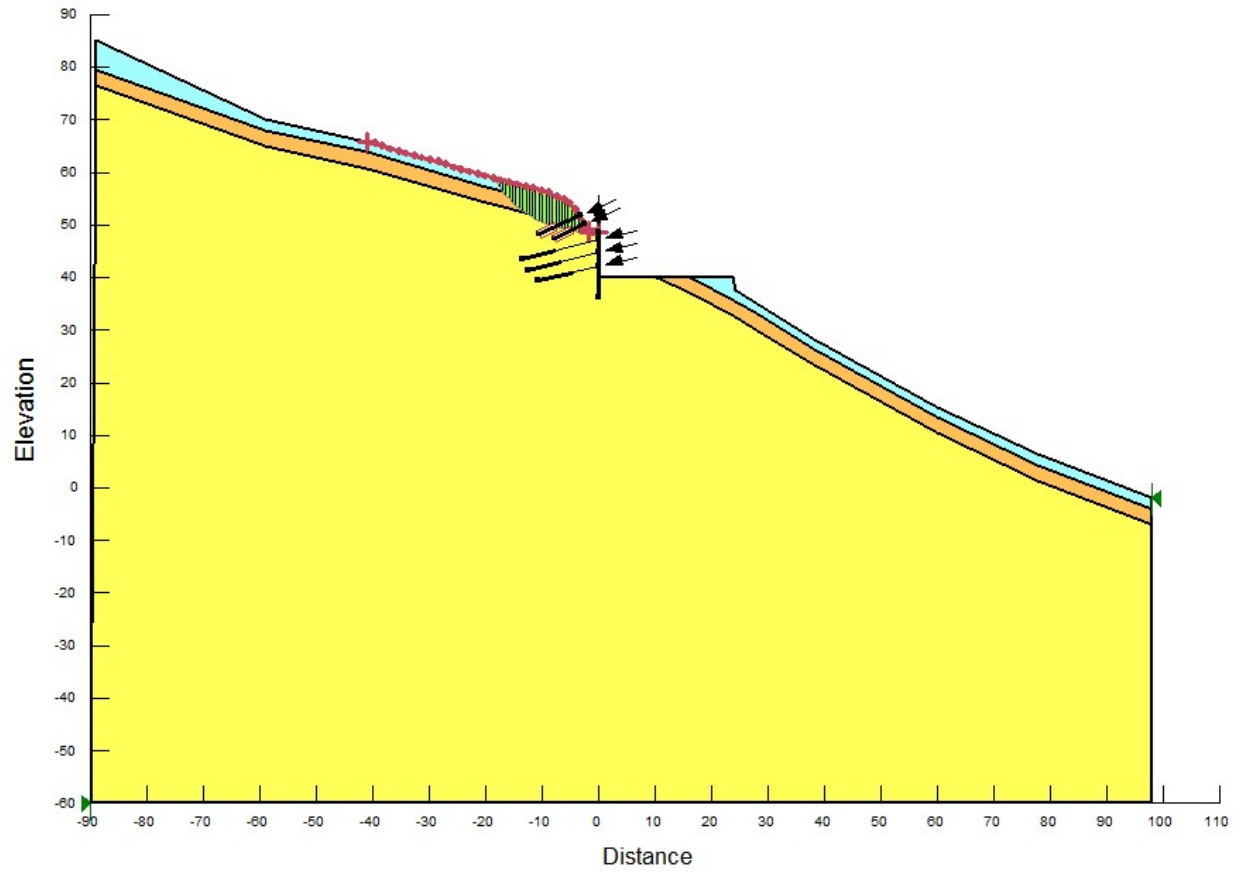
Figura 21: Coefficiente di sicurezza minimo per la stabilità globale in condizioni sismiche (EQK+M2) (+)
