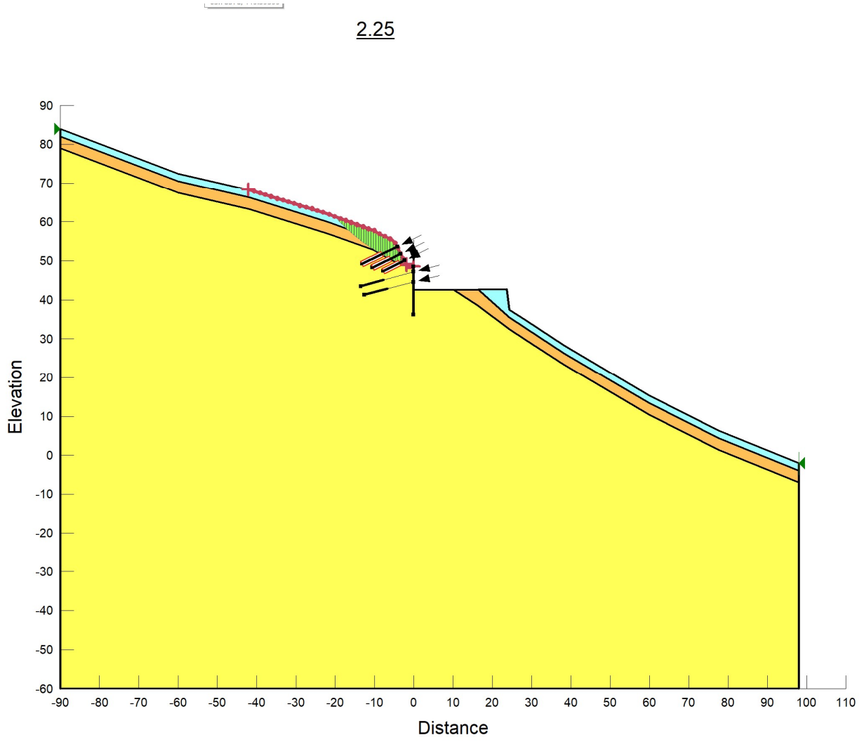
Figura 17: Coefficiente di sicurezza minimo per la stabilità globale in condizioni statiche (A2+M2)
