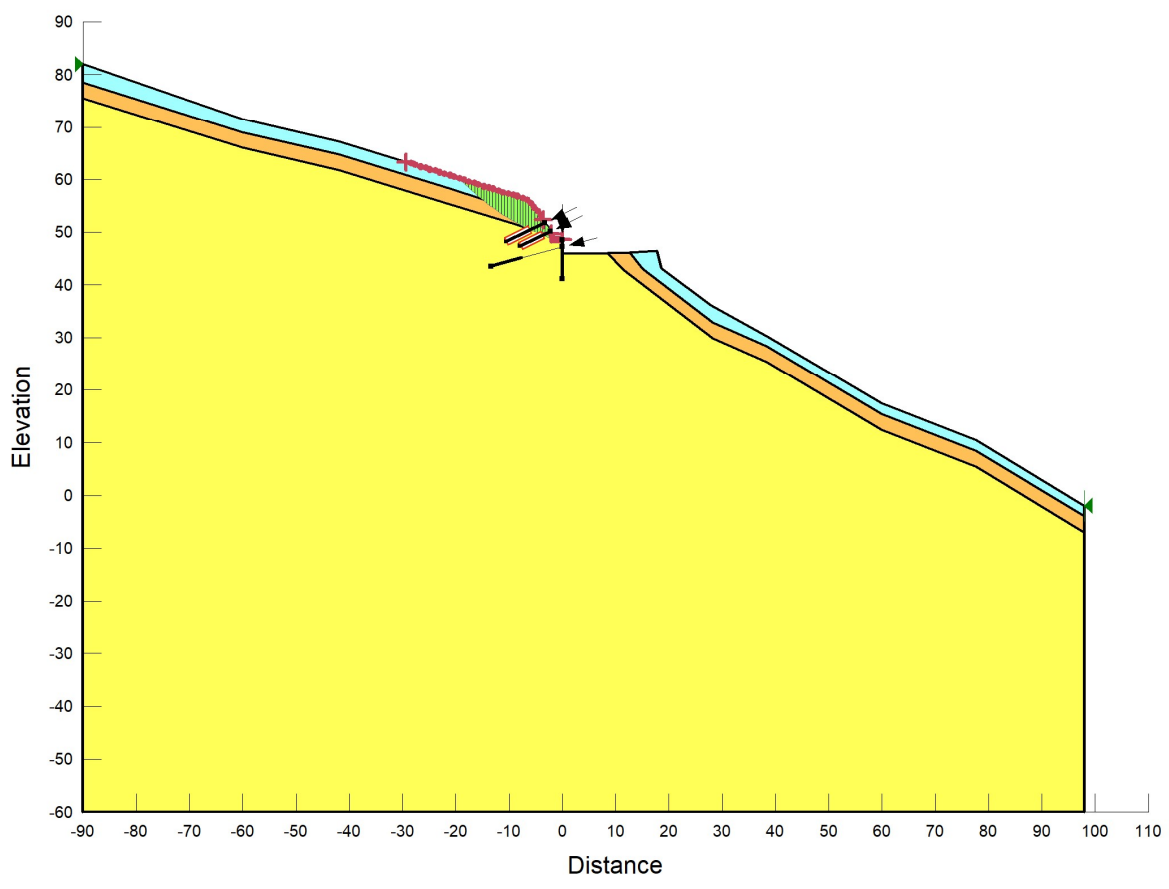
Figura 15: Coefficiente di sicurezza minimo per la stabilità globale in condizioni sismiche (EQK+M2) (+)
