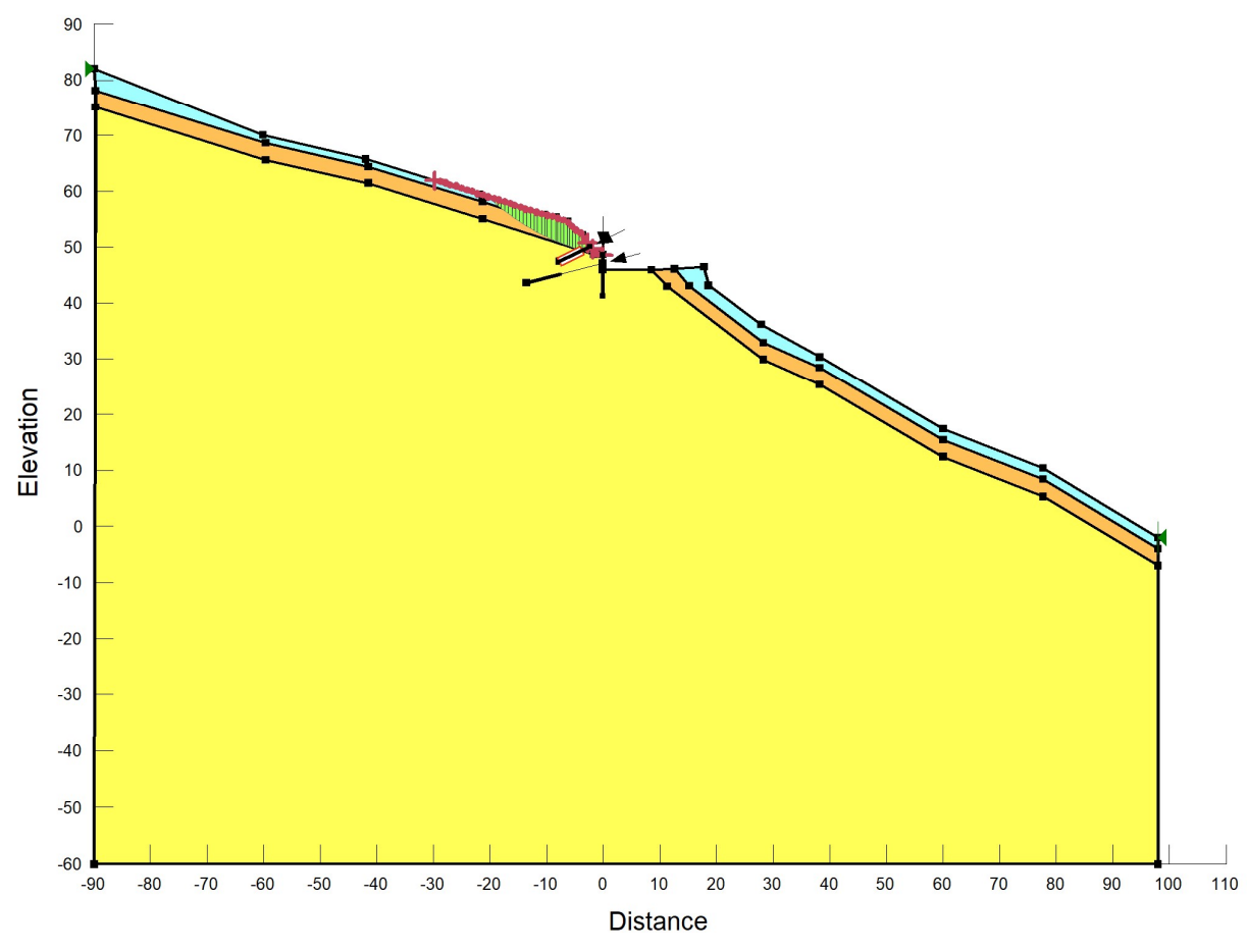
Figura 16: Coefficiente di sicurezza minimo per la stabilità globale in condizioni sismiche (EQK+M2) (-)
