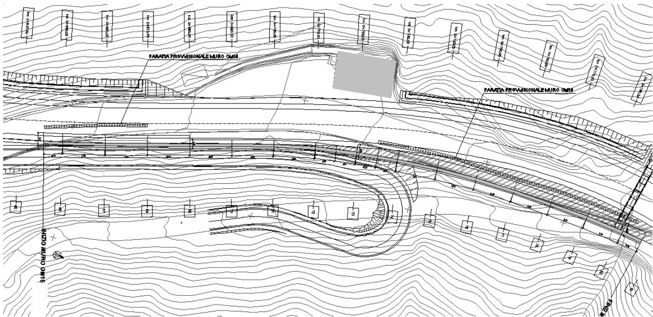
Figura 4 Planimetria d'intervento
