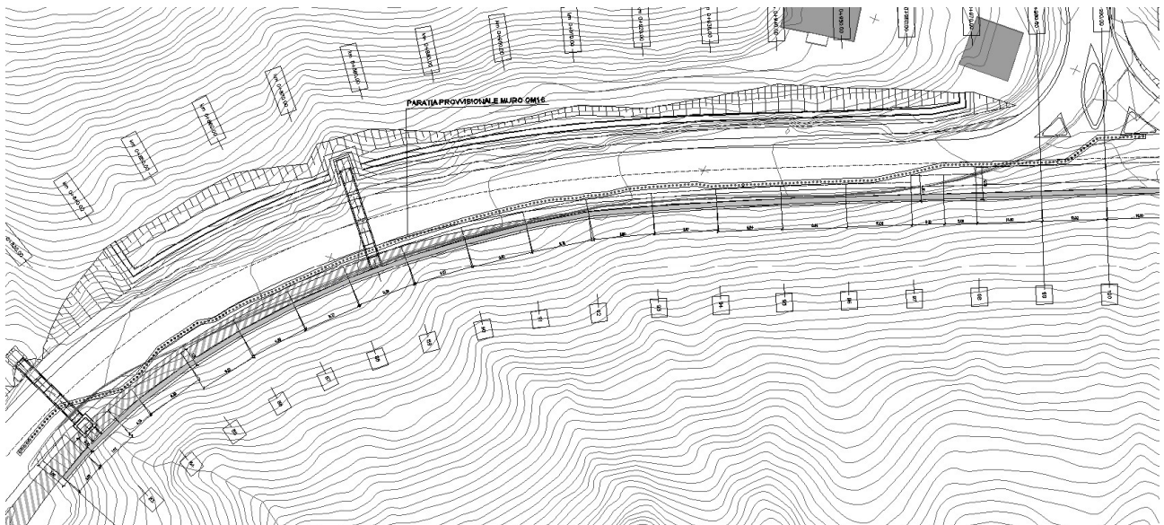
Figura 4 Planimetria d'intervento
