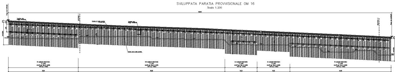
Figura 3: sviluppata paratia provvisoria
