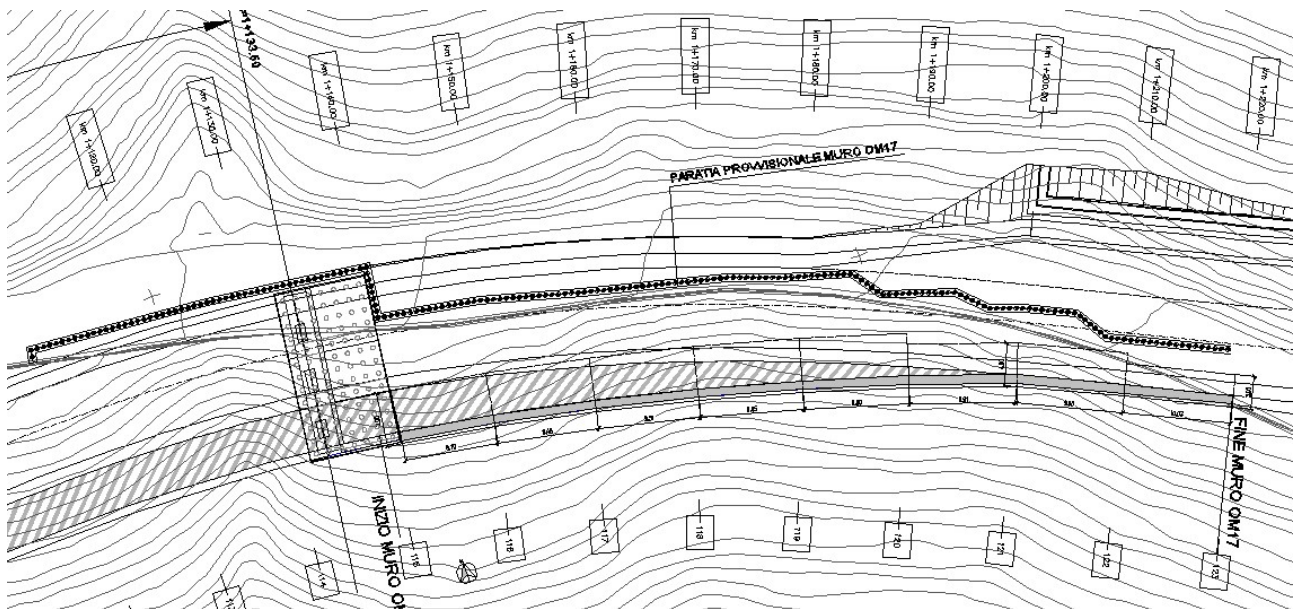
Figura 4 Planimetria d'intervento
